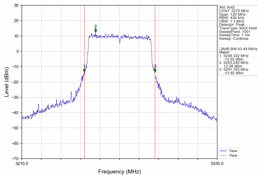
802.11be(EHT40)_LCH_5270MHz_SU_/_Ant2_NTNV
