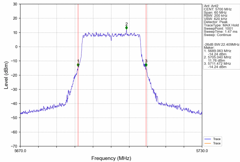
802.11be(EHT20)_HCH_5700MHz_SU_/_Ant2_NTNV
