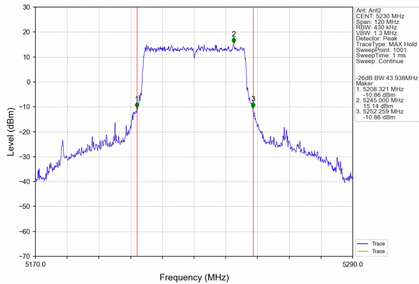
802.11be(EHT40)_HCH_5230MHz_SU_/_Ant2_NTNV
