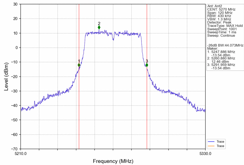
802.11ac(VHT40)_LCH_5270MHz_Ant2_NTNV
