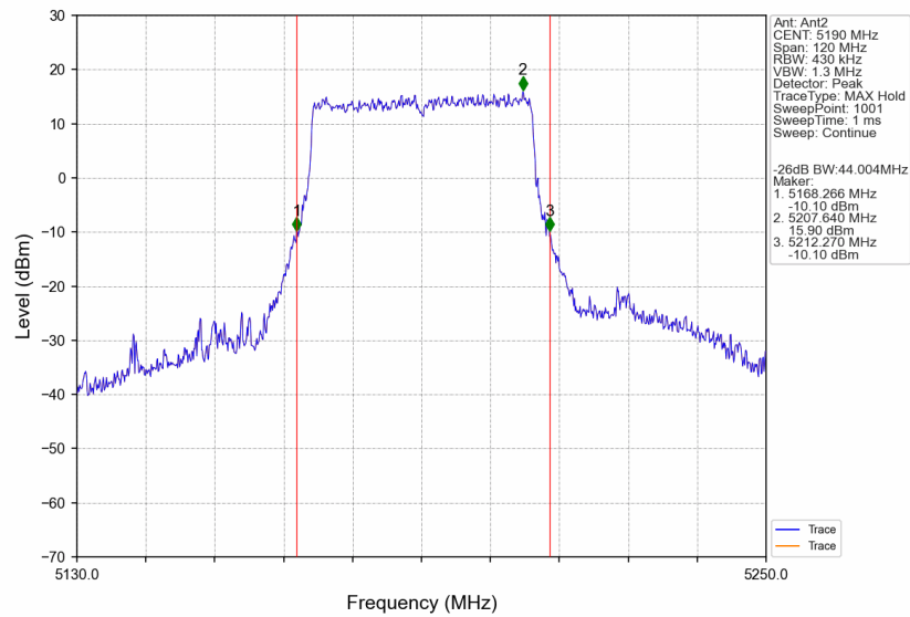
802.11be(EHT40)_LCH_5190MHz_SU_/_Ant2_NTNV
