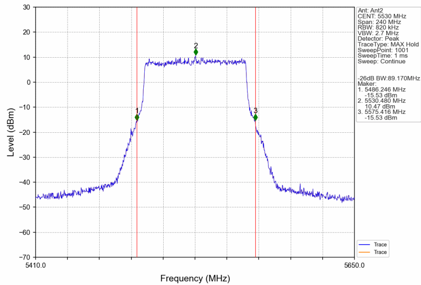
802.11ac(VHT80)_LCH_5530MHz_Ant2_NTNV
