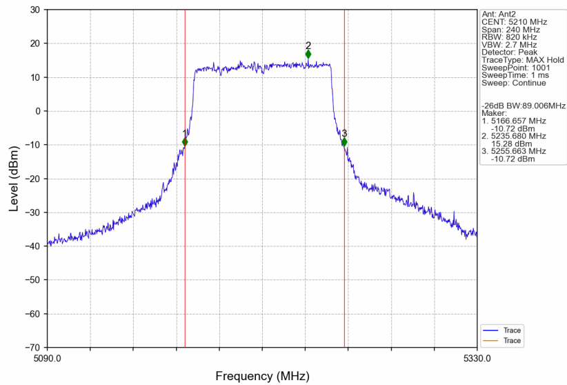
802.11ac(VHT80)_MCH_5210MHz_Ant2_NTNV
