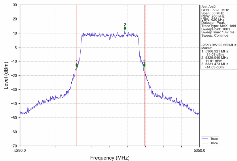
802.11be(EHT20)_HCH_5320MHz_SU_/_Ant2_NTNV
