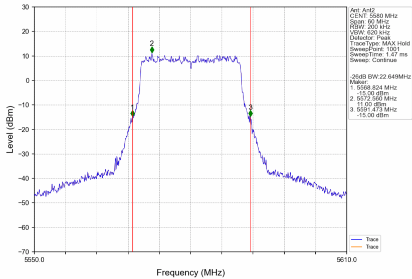
802.11be(EHT20)_MCH_5580MHz_SU_/_Ant2_NTNV
