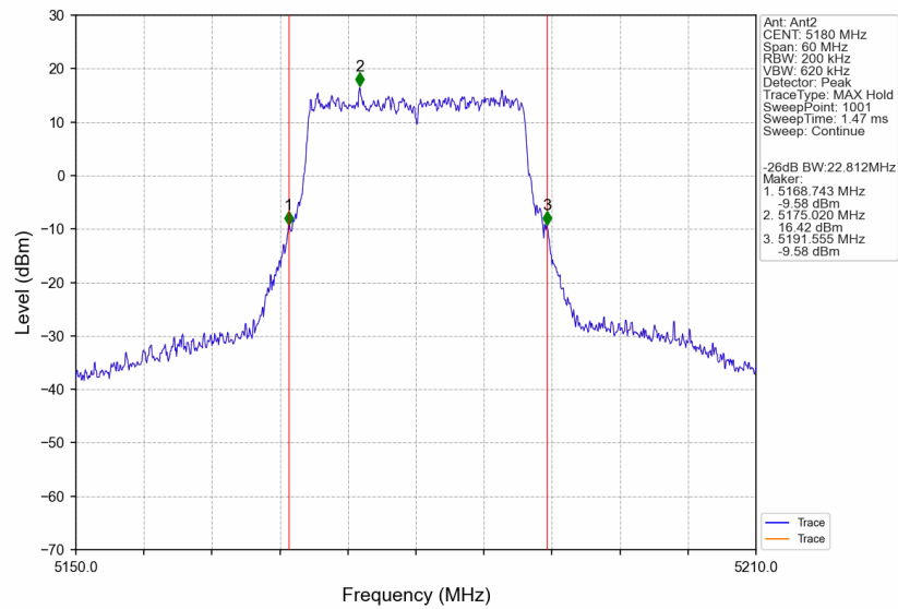
802.11be(EHT20)_LCH_5180MHz_SU_/_Ant2_NTNV
