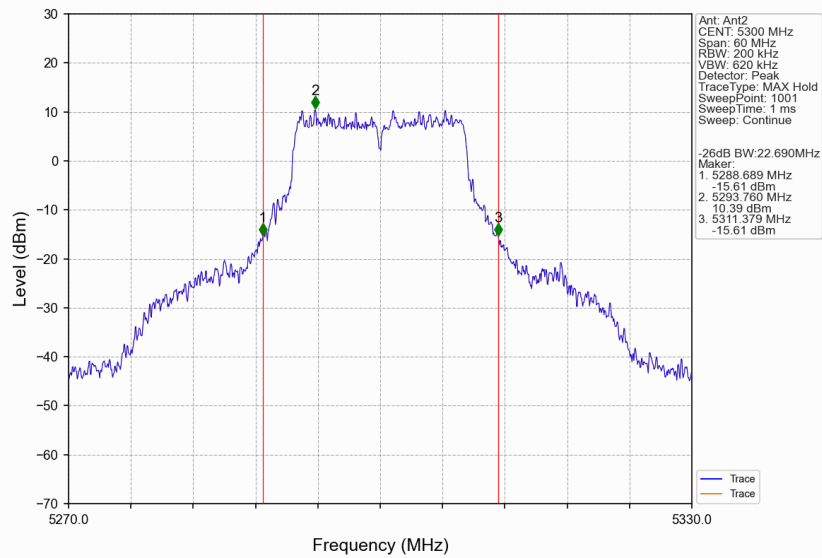
802.11a_MCH_5300MHz_Ant2_NTNV
