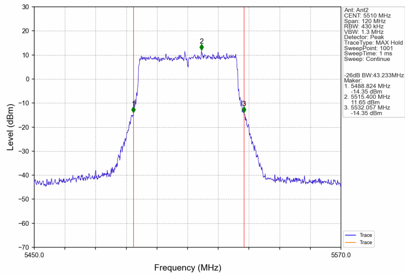
802.11be(EHT40)_LCH_5510MHz_SU_/_Ant2_NTNV
