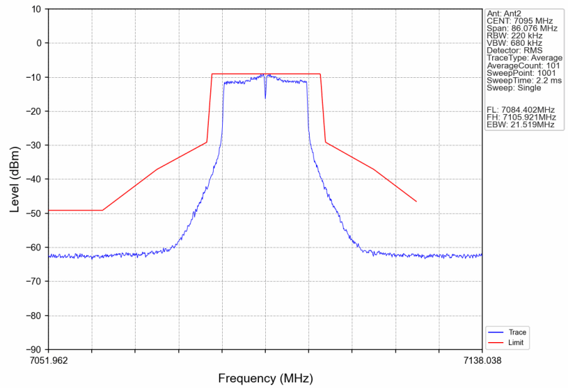
802.11a HCH 7095MHz Ant2 NTN
