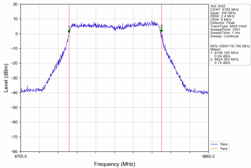
802.11ax(VHT80)_HCH_6785MHz_Ant2_NTNV
