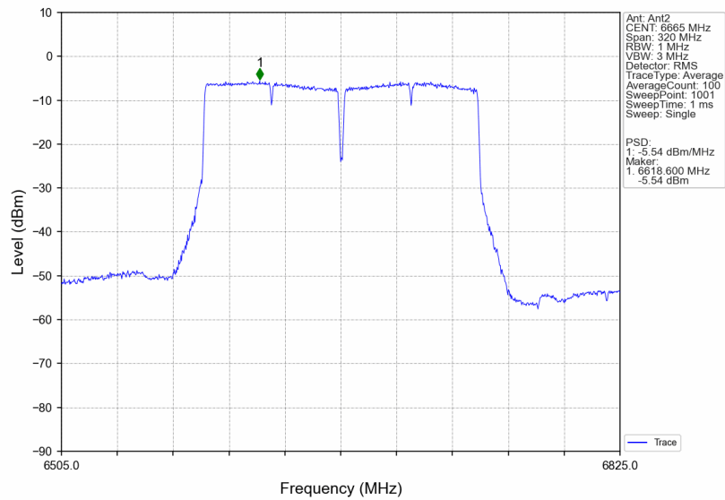
802.11ax(VHT160)_MCH_6665MHz_MIMO_NTNV
