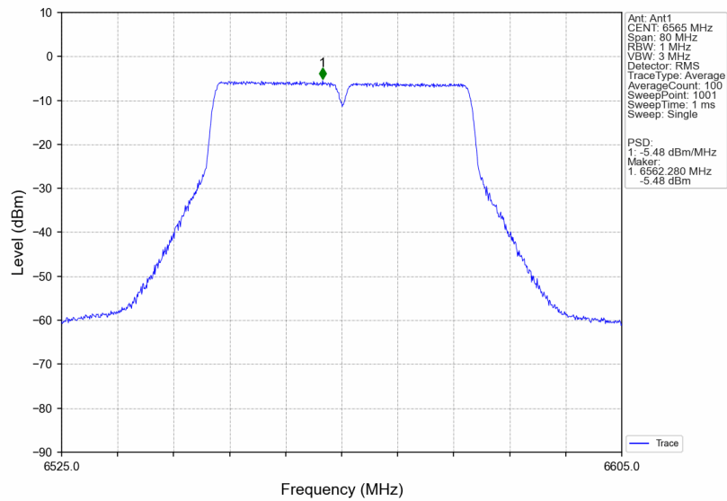
802.11ax(VHT40)_LCH_6565MHz_Ant1_NTNV
