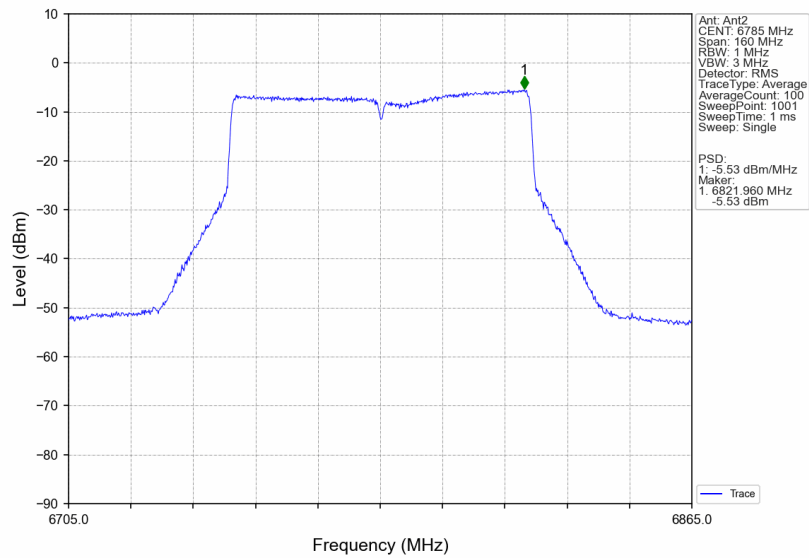
802.11ax(VHT80)_HCH_6785MHz_Ant2_NTNV
