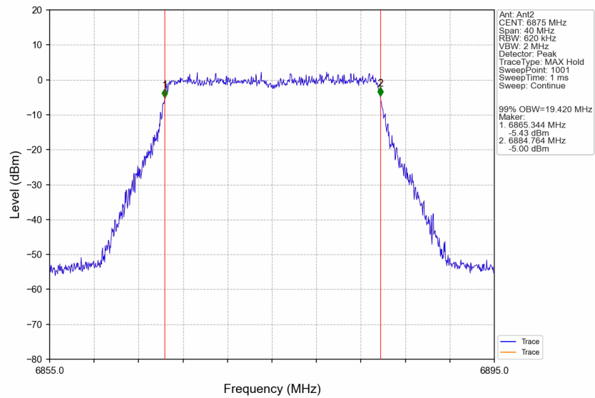
802.11be(EHT20)_HCH_6875MHz_RU242_Left_Ant2_NTNV
