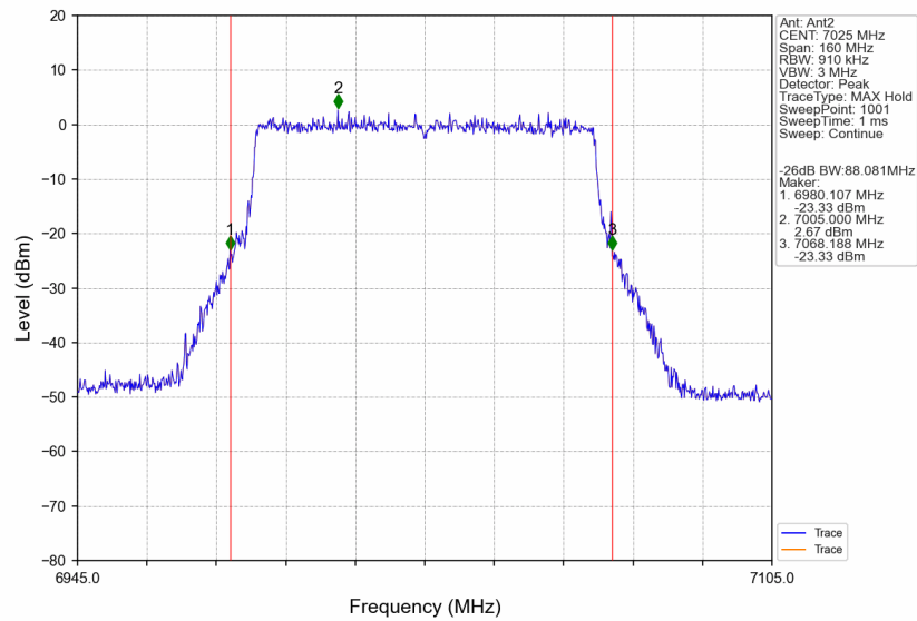
802.11be(EHT80)_HCH_7025MHz_RU996_Left_Ant2_NTNV
