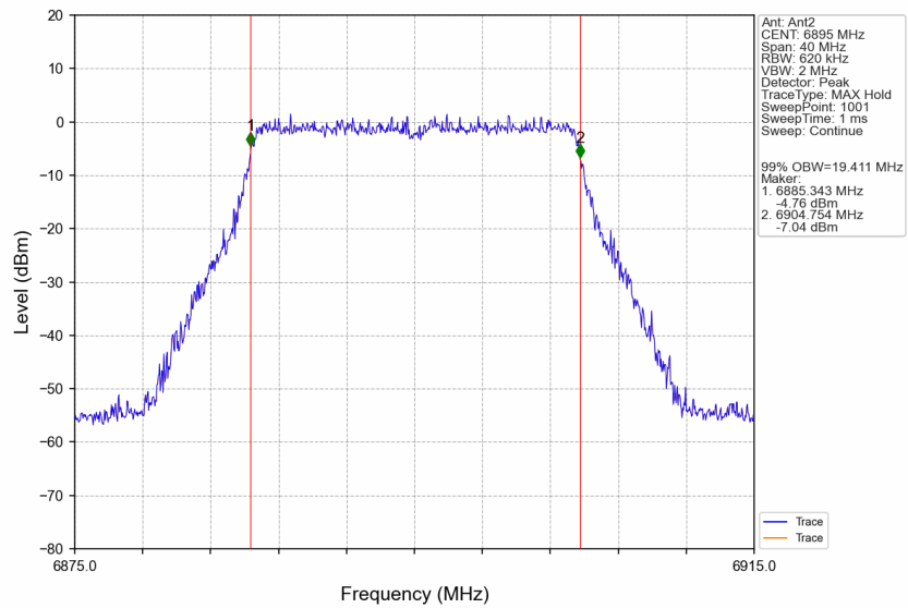
802.11be(EHT20)_LCH_6895MHz_RU242_Left_Ant2_NTNV
