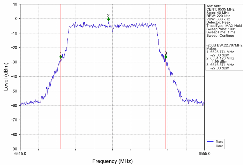
802.11be(EHT20)_LCH_6535MHz_RU242_Left_Ant2_NTNV
