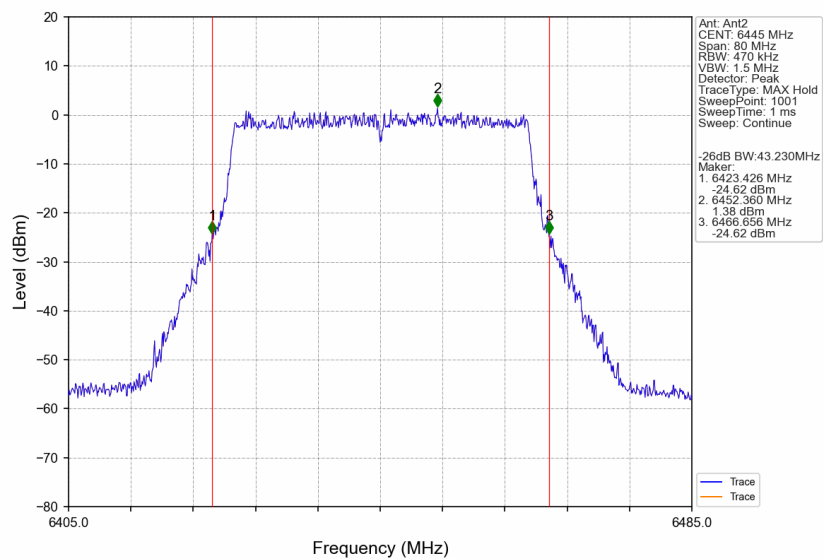
802.11be(EHT40)_LCH_6445MHz_RU484_Left_Ant2_NTNV
