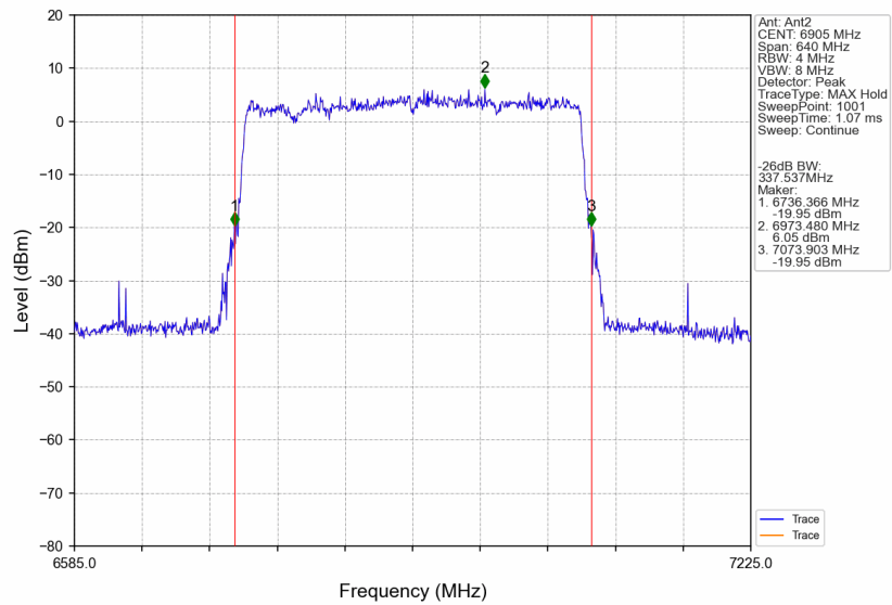
802.11be(EHT320)_HCH_6905MHz_4xRU996_Left_Ant2_NTNV
