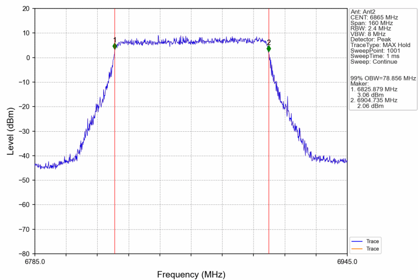
802.11be(EHT80)_HCH_6865MHz_RU996_Left_Ant2_NTNV
