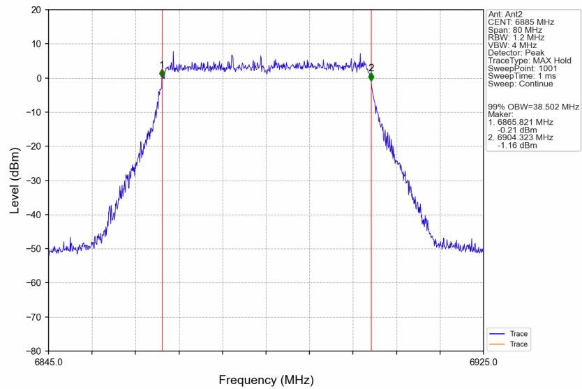
802.11be(EHT40)_HCH_6885MHz_RU484_Left_Ant2_NTNV
