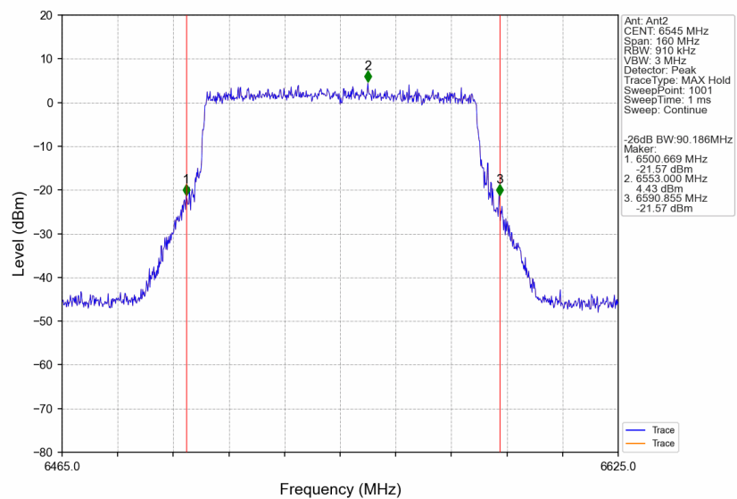
802.11be(EHT80)_HCH_6545MHz_RU996_Left_Ant2_NTNV
