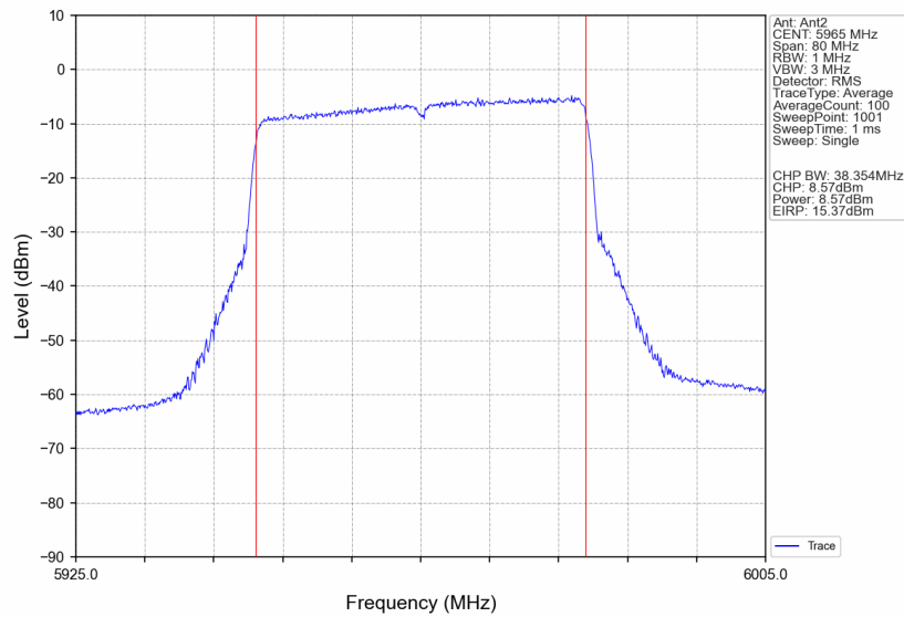
802.11be(EHT40)_LCH_5965MHz_RU484_Left_Ant2_NTNV
