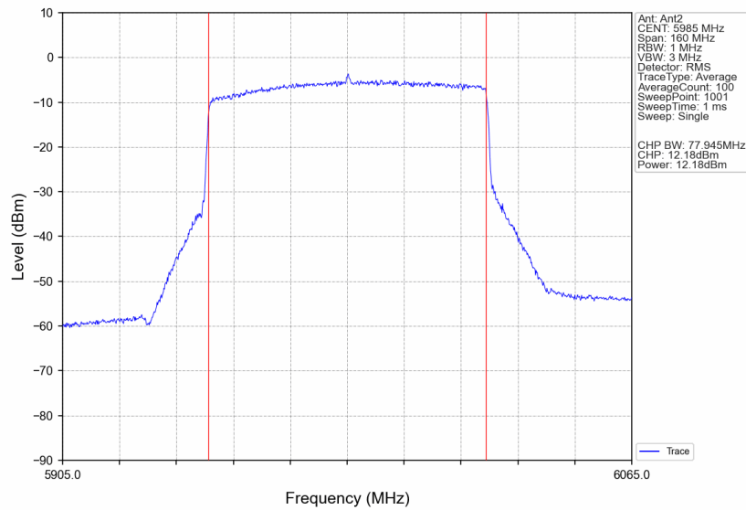
802.11be(EHT80)_LCH_5985MHz_RU996_Left_Ant2_NTNV
