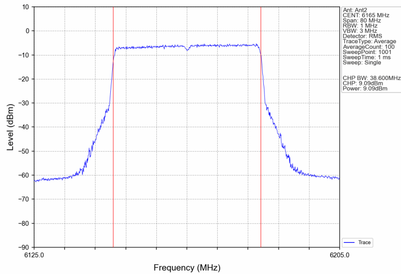
802.11be(EHT40)_MCH_6165MHz_RU484_Left_Ant2_NTNV
