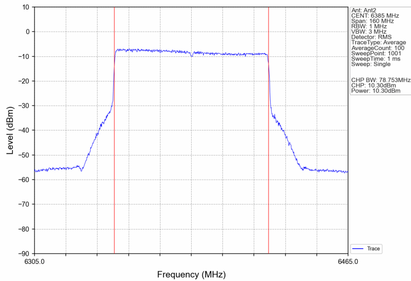
802.11be(EHT80)_HCH_6385MHz_RU996_Left_Ant2_NTNV
