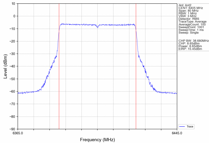
802.11be(EHT40)_HCH_6405MHz_RU484_Left_Ant2_NTNV
