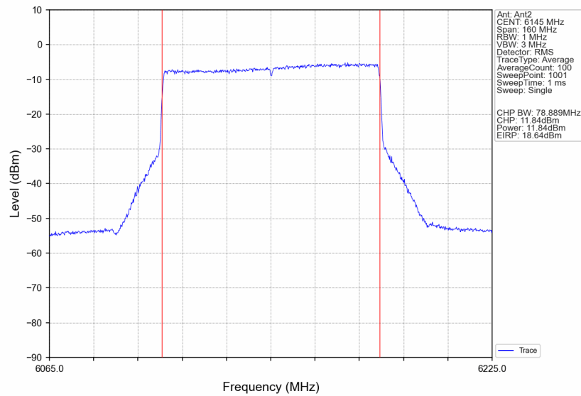
802.11be(EHT80)_MCH_6145MHz_RU996_Left_Ant2_NTNV
