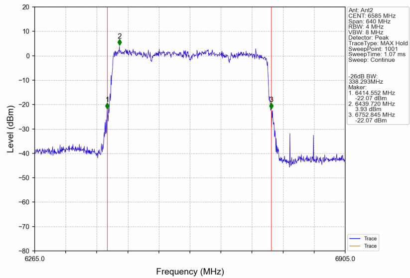
802.11be(EHT320)_MCH_6585MHz_4xRU996_Left_Ant2_NTNV
