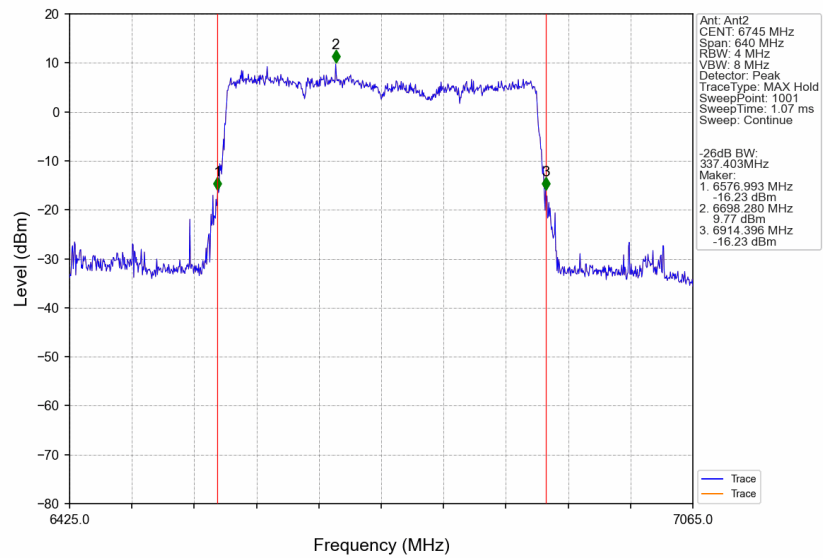
802.11be(EHT320)_LCH_6745MHz_4xRU996_Left_Ant2_NTNV
