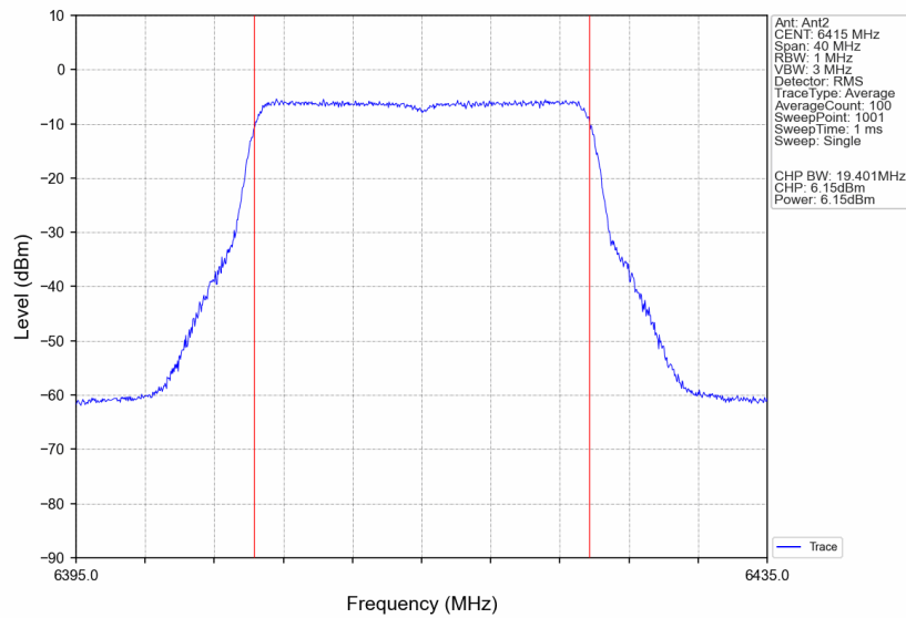
802.11be(EHT20)_HCH_6415MHz_RU242_Left_Ant2_NTNV
