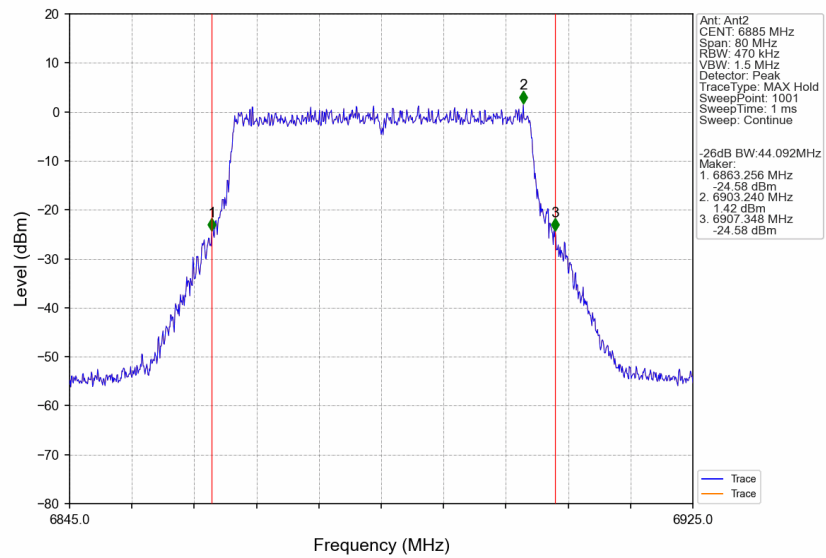
802.11be(EHT40)_HCH_6885MHz_RU484_Left_Ant2_NTNV
