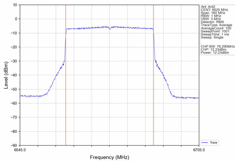
802.11be(EHT80)_LCH_6625MHz_RU996_Left_Ant2_NTNV
