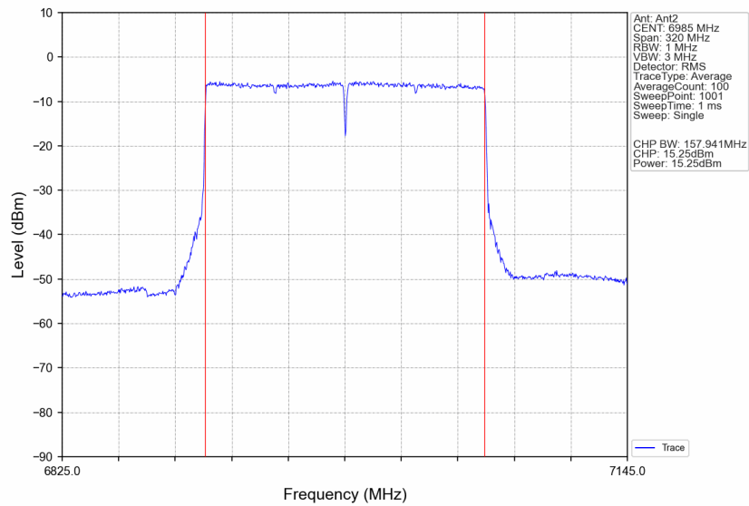
802.11be(EHT160)_MCH_6985MHz_2xRU996_Left_Ant2_NTNV
