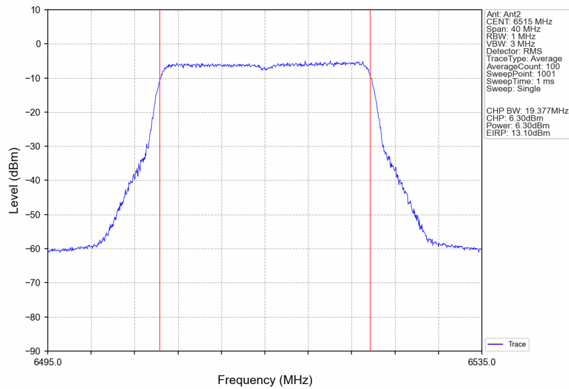
802.11be(EHT20)_HCH_6515MHz_RU242_Left_Ant2_NTNV
