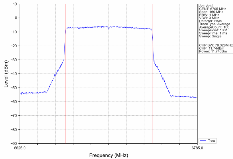
802.11be(EHT80)_MCH_6705MHz_RU996_Left_Ant2_NTNV
