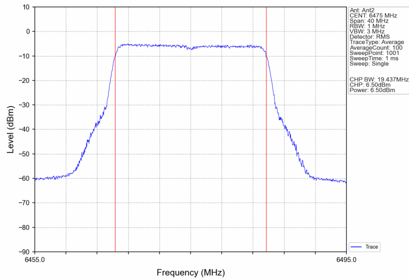
802.11be(EHT20)_MCH_6475MHz_RU242_Left_Ant2_NTNV
