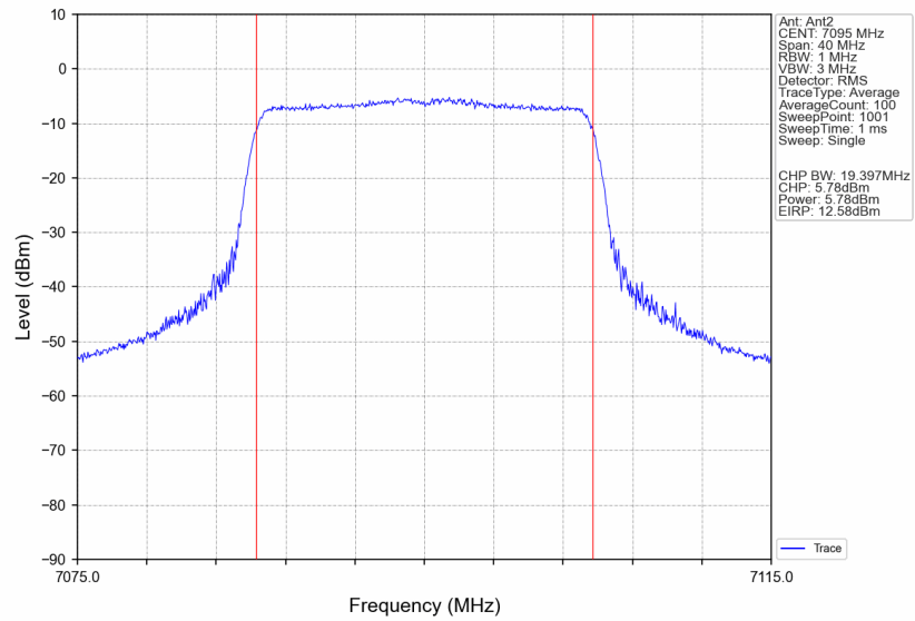
802.11be(EHT20)_HCH_7095MHz_RU242_Left_Ant2_NTNV
