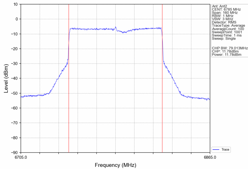
802.11be(EHT80)_HCH_6785MHz_RU996_Left_Ant2_NTNV
