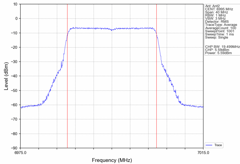
802.11be(EHT20)_MCH_6995MHz_RU242_Left_Ant2_NTNV
