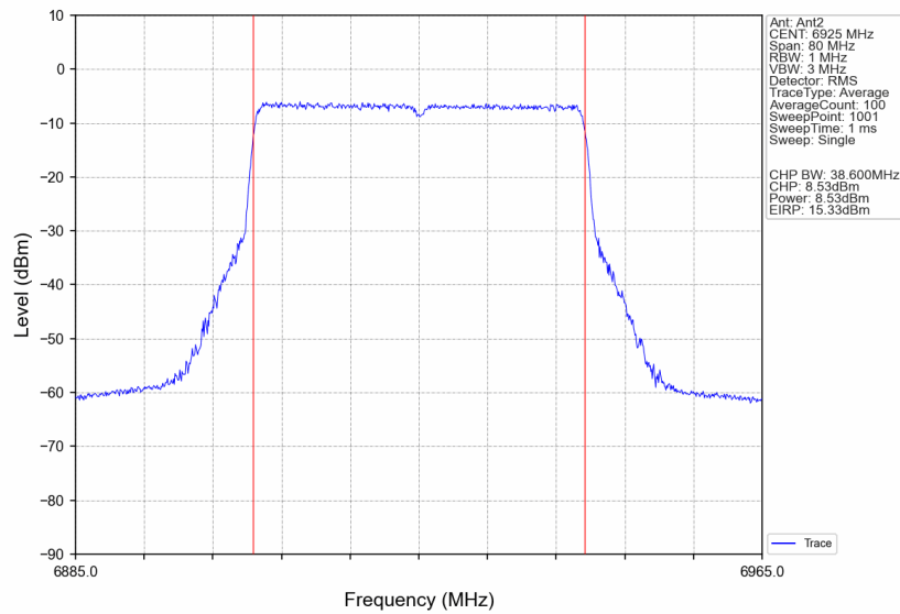
802.11be(EHT40)_LCH_6925MHz_RU484_Left_Ant2_NTNV
