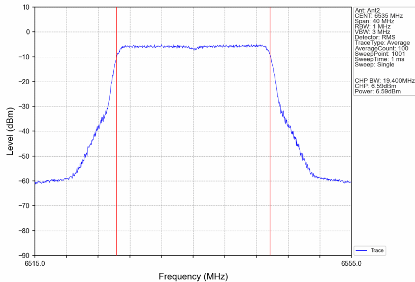
802.11be(EHT20)_LCH_6535MHz_RU242_Left_Ant2_NTNV
