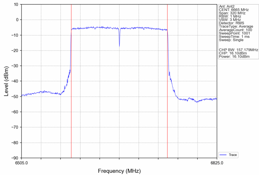
802.11be(EHT160)_MCH_6665MHz_2xRU996_Left_Ant2_NTNV
