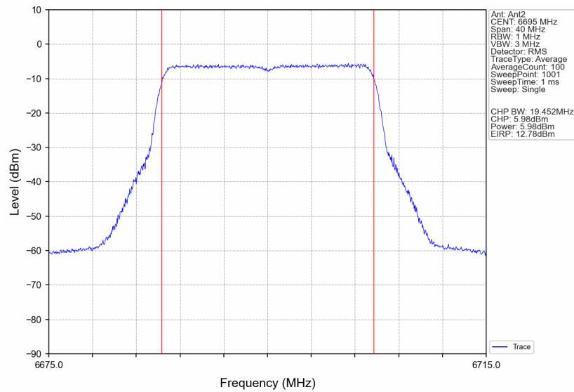
802.11be(EHT20)_MCH_6695MHz_RU242_Left_Ant2_NTNV
