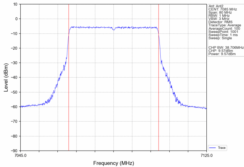
802.11be(EHT40)_HCH_7085MHz_RU484_Left_Ant2_NTNV
