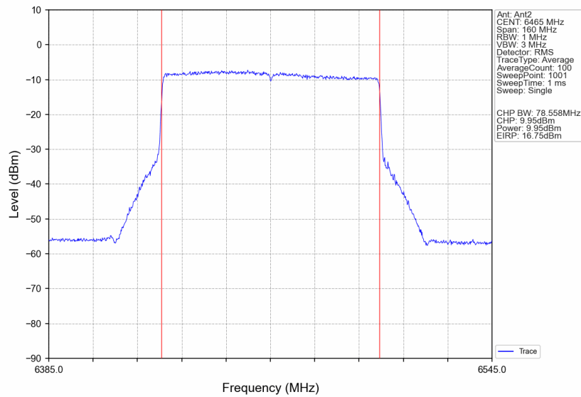
802.11be(EHT80)_LCH_6465MHz_RU996_Left_Ant2_NTNV
