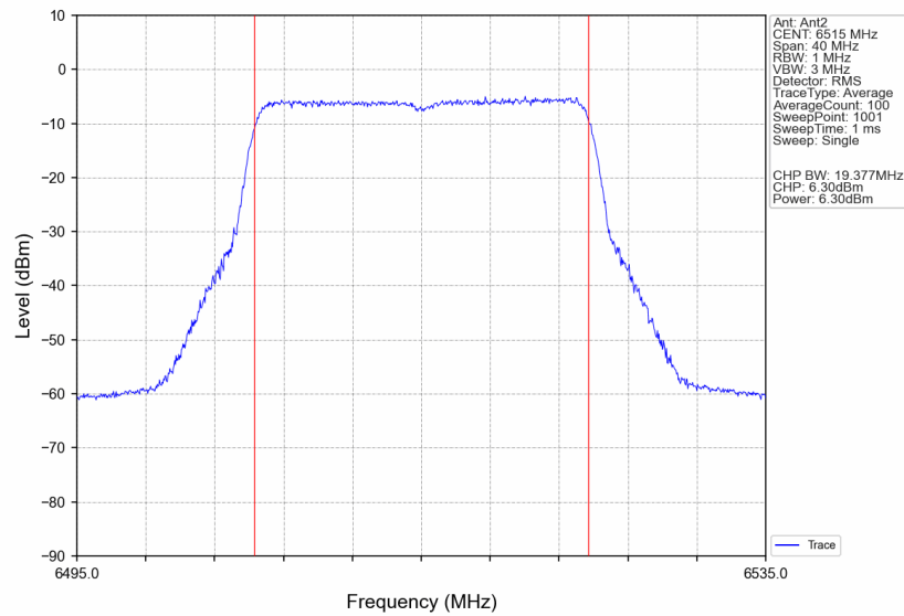
802.11be(EHT20)_HCH_6515MHz_RU242_Left_Ant2_NTNV
