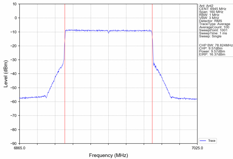
802.11be(EHT80)_LCH_6945MHz_RU996_Left_Ant2_NTNV
