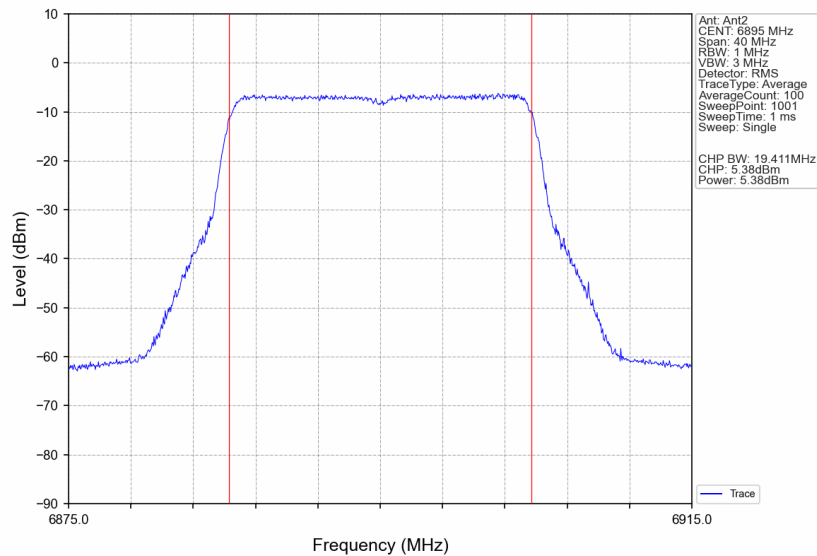
802.11be(EHT20)_LCH_6895MHz_RU242_Left_Ant2_NTNV
