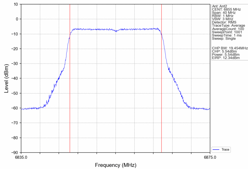
802.11be(EHT20)_HCH_6855MHz_RU242_Left_Ant2_NTNV
