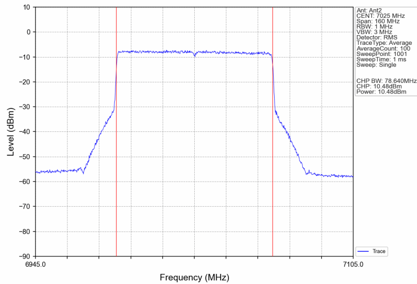
802.11be(EHT80)_HCH_7025MHz_RU996_Left_Ant2_NTNV
