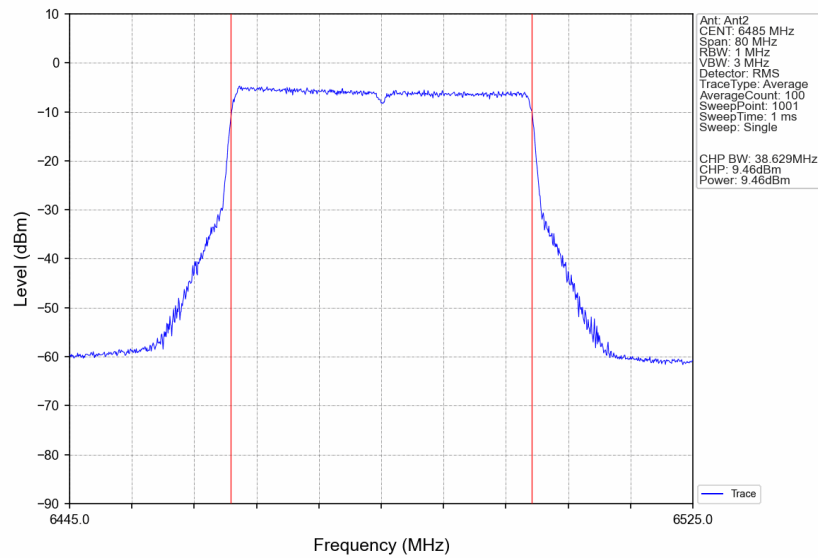
802.11be(EHT40)_MCH_6485MHz_RU484_Left_Ant2_NTNV
