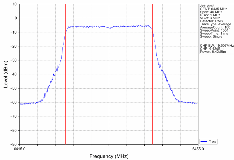
802.11be(EHT20)_LCH_6435MHz_RU242_Left_Ant2_NTNV
