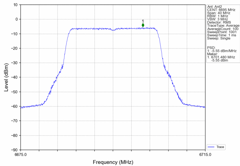
802.11be(EHT20)_MCH_6695MHz_RU242_Left_MIMO_NTNV
