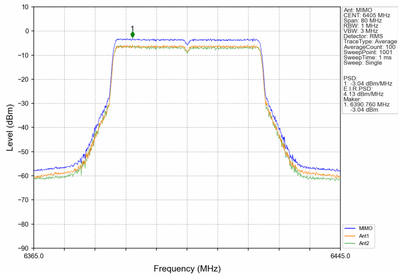
802.11be(EHT40)_HCH_6405MHz_RU484_Left_MIMO_NTNV
