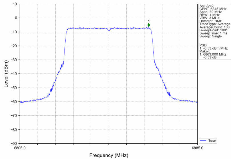
802.11be(EHT40)_HCH_6845MHz_RU484_Left_MIMO_NTNV
