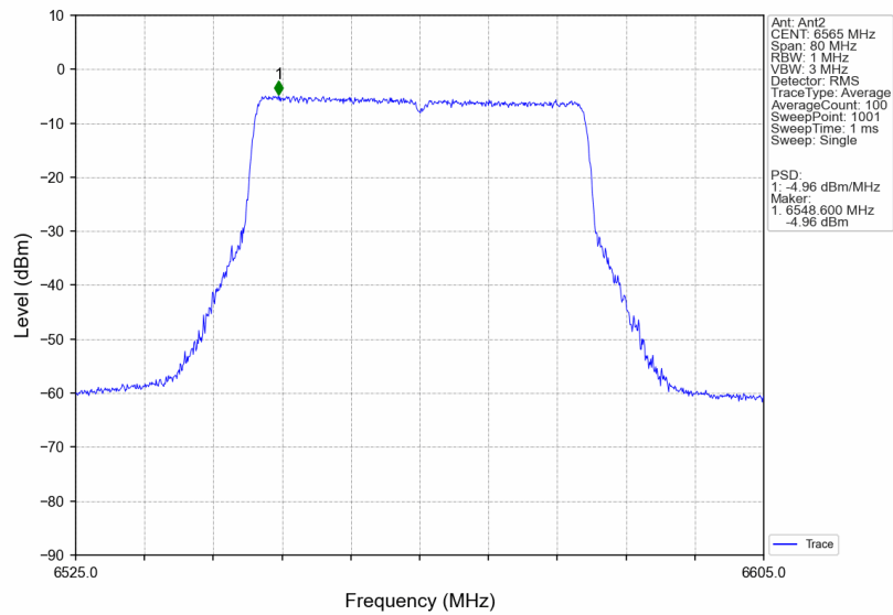
802.11be(EHT40)_LCH_6565MHz_RU484_Left_MIMO_NTNV
