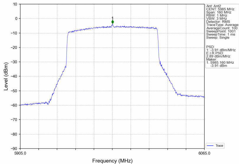
802.11be(EHT80)_LCH_5985MHz_RU996_Left_Ant2_NTNV
