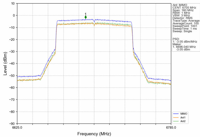
802.11be(EHT80)_MCH_6705MHz_RU996_Left_MIMO_NTNV
