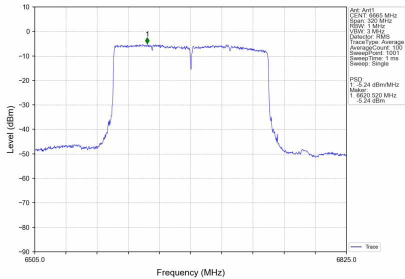
802.11be(EHT160)_MCH_6665MHz_2xRU996_Left_Ant1_NTNV
