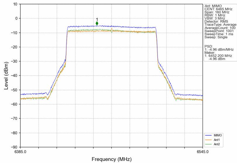
802.11be(EHT80)_LCH_6465MHz_RU996_Left_MIMO_NTNV
