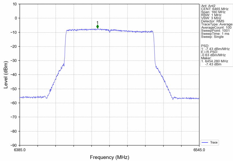
802.11be(EHT80)_LCH_6465MHz_RU996_Left_MIMO_NTNV
