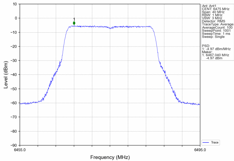
802.11be(EHT20)_MCH_6475MHz_RU242_Left_Ant1_NTNV
