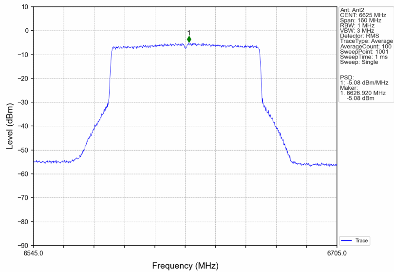
802.11be(EHT80)_LCH_6625MHz_RU996_Left_Ant2_NTNV
