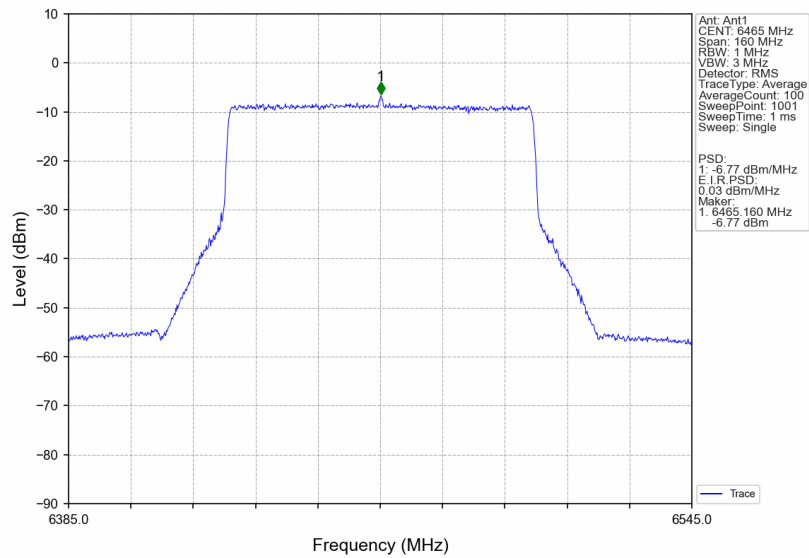
802.11be(EHT80) LCH_6465MHz_RU996_Left_Ant1_NTNV
