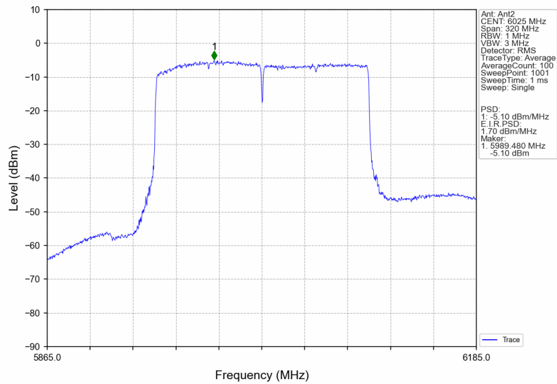
802.11be(EHT160)_LCH_6025MHz_2xRU996_Left_MIMO_NTNV
