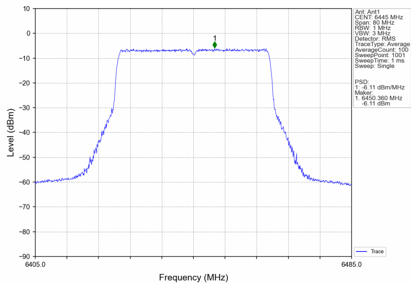
802.11be(EHT40)_LCH_6445MHz_RU484_Left_Ant1_NTNV
