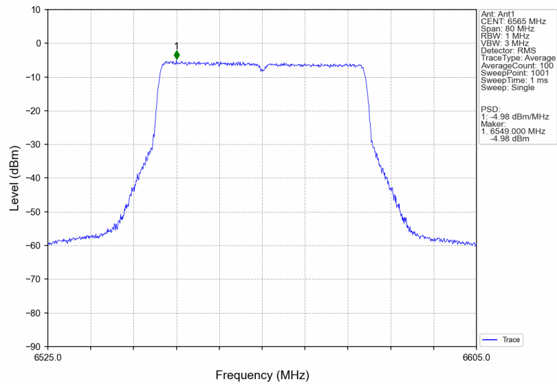
802.11be(EHT40)_LCH_6565MHz_RU484_Left_Ant1_NTNV
