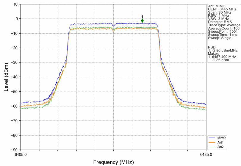
802.11be(EHT40)_LCH_6445MHz_RU484_Left_MIMO_NTNV
