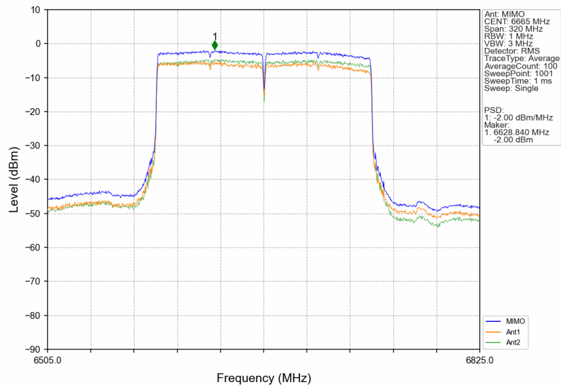
802.11be(EHT160)_MCH_6665MHz_2xRU996_Left_MIMO_NTNV
