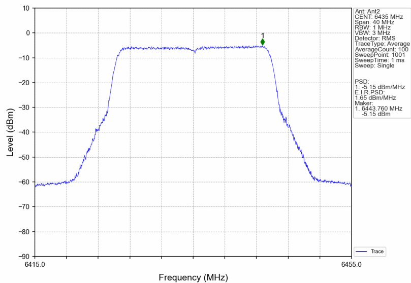
802.11be(EHT20)_LCH_6435MHz_RU242_Left_Ant2_NTNV
