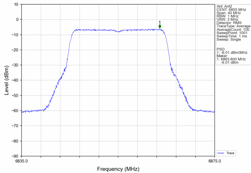
802.11be(EHT20)_HCH_6855MHz_RU242_Left_Ant2_NTNV
