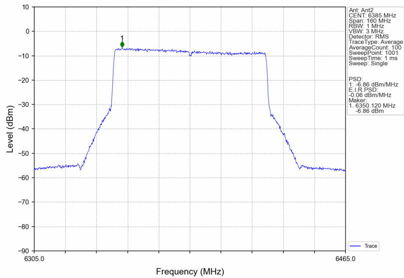
802.11be(EHT80)_HCH_6385MHz_RU996_Left_Ant2_NTNV
