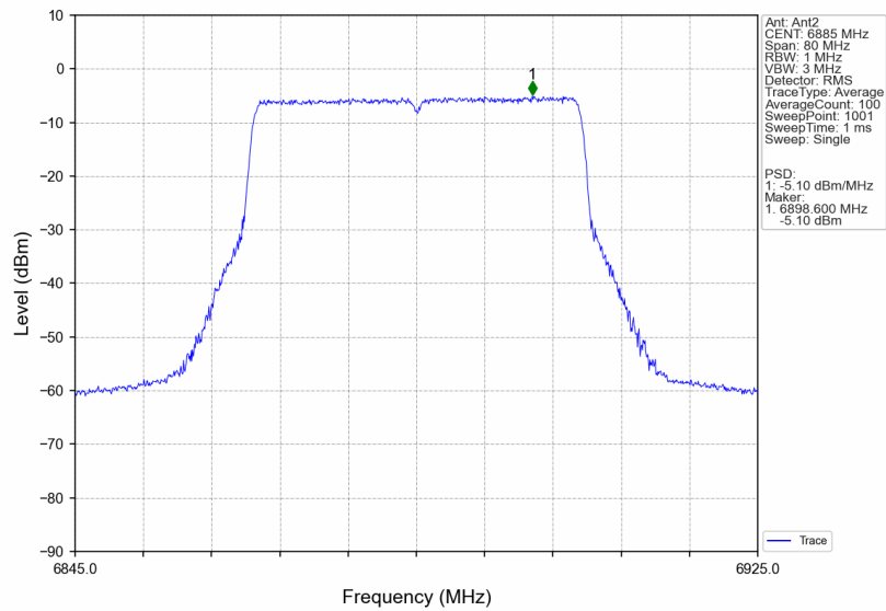
802.11be(EHT40)_HCH_6885MHz_RU484_Left_MIMO_NTNV
