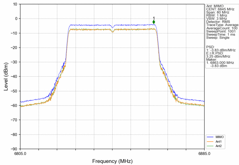
802.11be(EHT40)_HCH_6845MHz_RU484_Left_MIMO_NTNV
