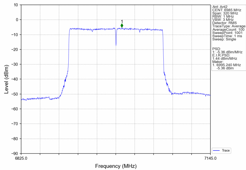
802.11be(EHT160)_MCH_6985MHz_2xRU996_Left_MIMO_NTNV
