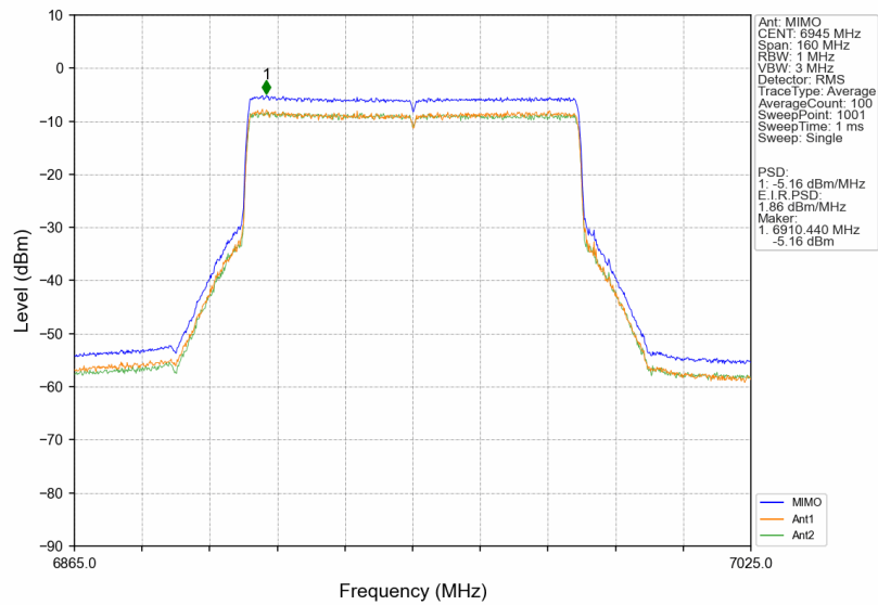
802.11be(EHT80)_LCH_6945MHz_RU996_Left_MIMO_NTNV
