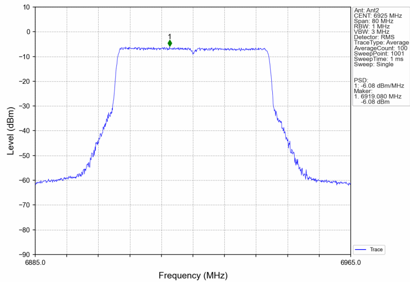
802.11be(EHT40)_LCH_6925MHz_RU484_Left_Ant2_NTNV
