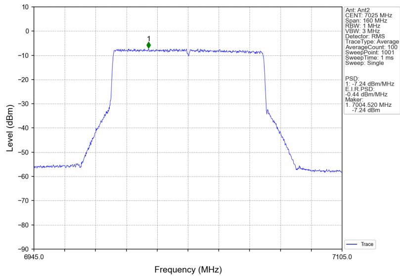
802.11be(EHT80)_HCH_7025MHz_RU996_Left_Ant2_NTNV
