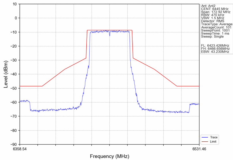
802.11be(EHT40)_LCH_6445MHz_RU484_Left_Ant2_NTNV
