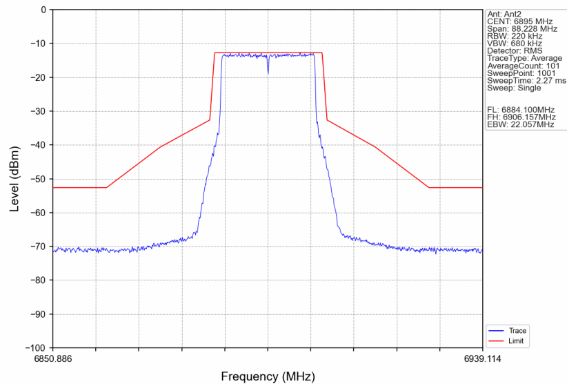
802.11be(EHT20)_LCH_6895MHz_RU242_Left_Ant2_NTNV
