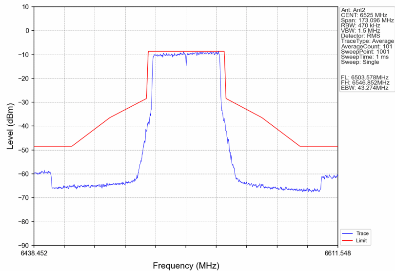
802.11be(EHT40)_HCH_6525MHz_RU484_Left_Ant2_NTNV
