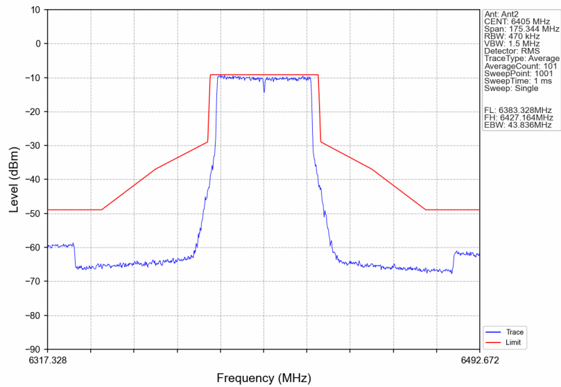
802.11be(EHT40)_HCH_6405MHz_RU484_Left_Ant2_NTNV
