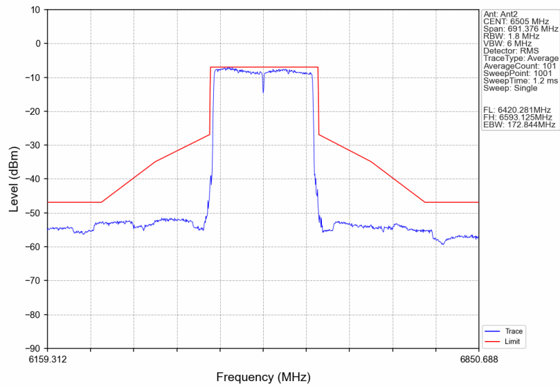
802.11be(EHT160)_HCH_6505MHz_2xRU996_Left_Ant2_NTNV
