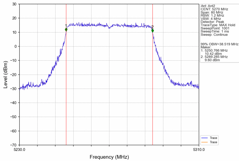
802.11be(EHT40)_LCH_5270MHz_SU_/_Ant2_NTNV
