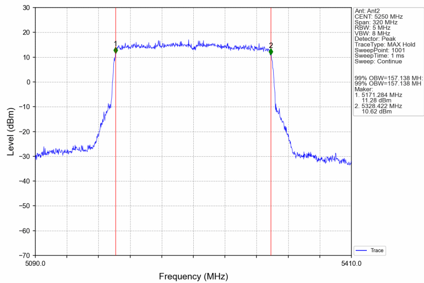
802.11be(EHT160)_MCH_5250MHz_SU_/_Ant2_NTNV
