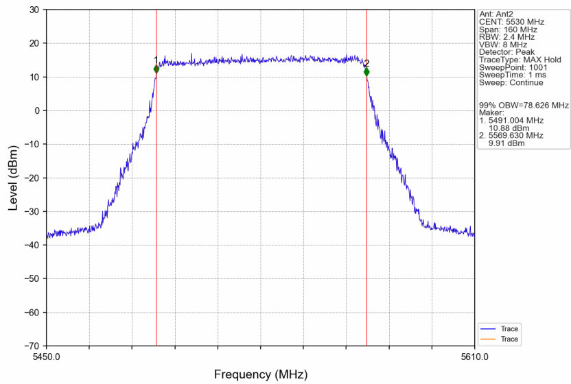
802.11be(EHT80)_LCH_5530MHz_SU_/_Ant2_NTNV
