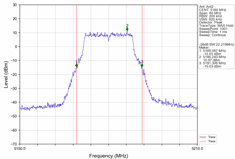
802.11a_LCH_5180MHz_Ant2_NTNV
