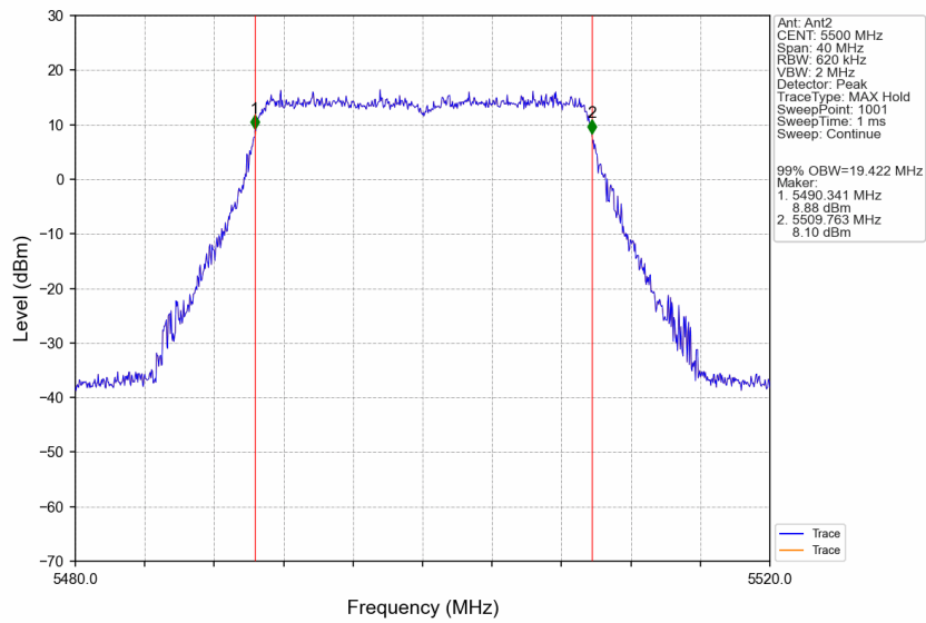
802.11be(EHT20)_LCH_5500MHz_SU_/_Ant2_NTNV
