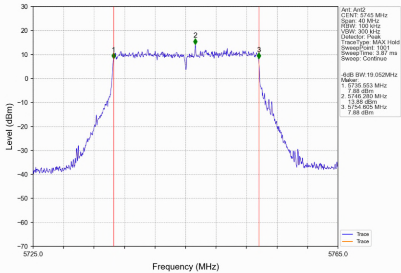
802.11be(EHT20)_LCH_5745MHz_SU_/_Ant2_NTNV
