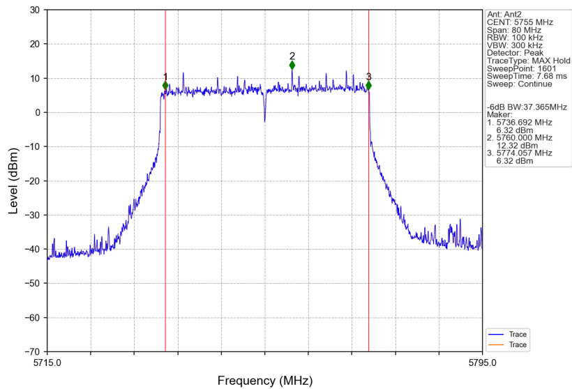
802.11be(EHT40)_LCH_5755MHz_SU_/_Ant2_NTNV
