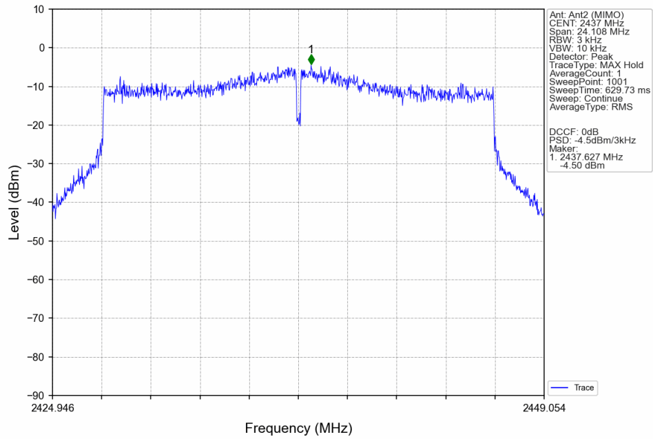
802.11be(EHT20)_MCH_2437MHz_SU / _MIMO_NTNV
