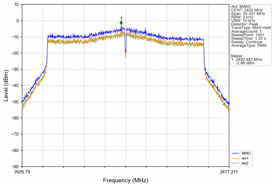
802.11be(EHT40)_HCH_2452MHz_SU / MIMO_NTNV
