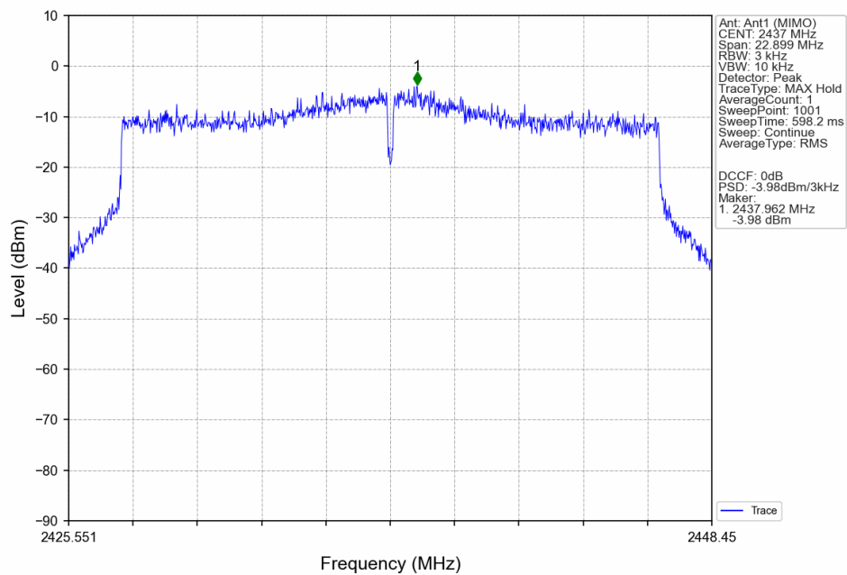
802.11be(EHT20)_MCH_2437MHz_SU / _Ant1 (MIMO)_NTNV
