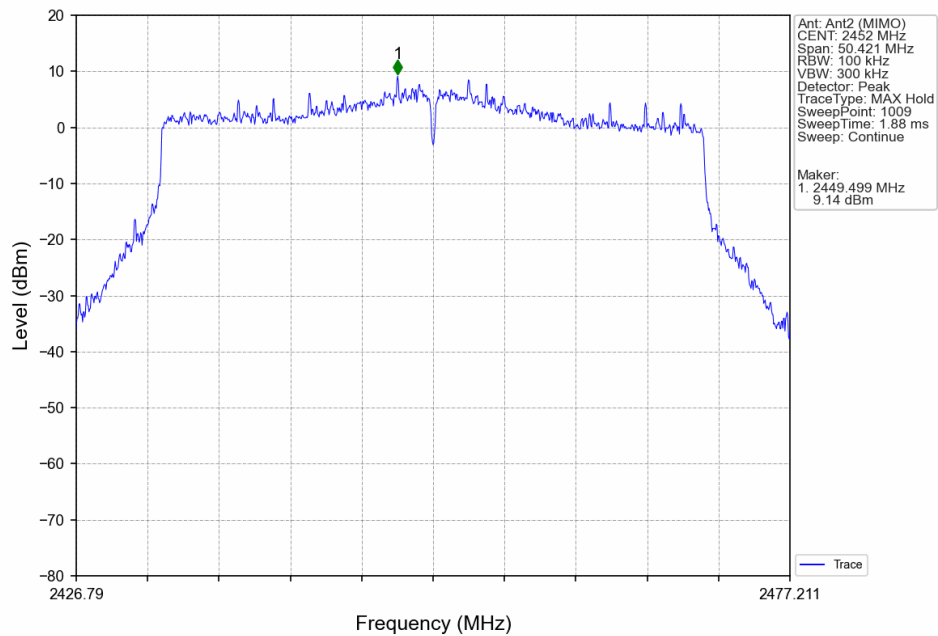
802.11be(EHT40)_HCH_2452MHz_SU_/_Ant2 (MIMO)_NTNV
