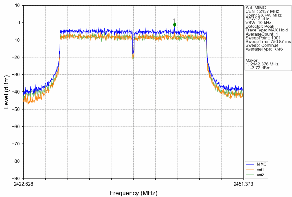
802.11ax(HEW20)_MCH_2437MHz_SU_/_MIMO_NTNV
