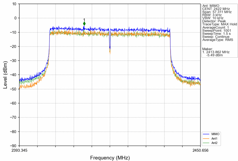
802.11ax(HEW40) LCH_2422MHz_SU / _MIMO_NTNV
