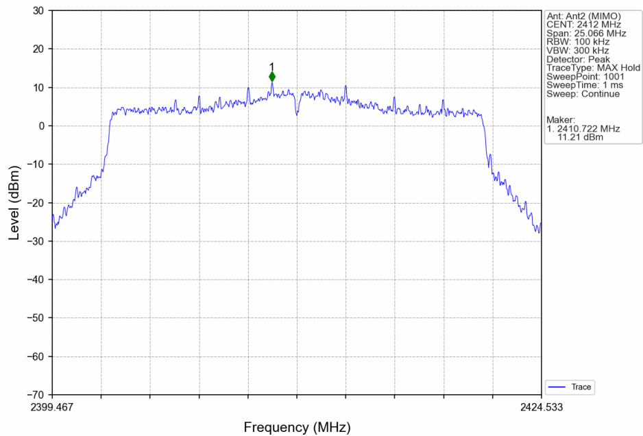
802.11be(EHT20)_LCH_2412MHz_SU_ / Ant2 (MIMO)_NTNV
