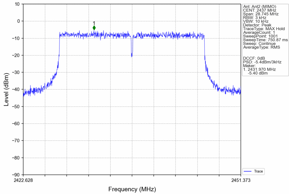
802.11ax(HEW20)_MCH_2437MHz_SU_/_MIMO_NTNV
