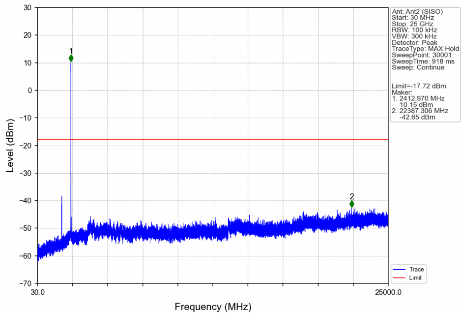
802.11b_LCH_2412MHz_Ant2 (SISO)_NTNV
