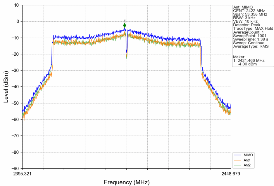
802.11be(EHT40)_LCH_2422MHz_SU_ / _MIMO_NTNV
