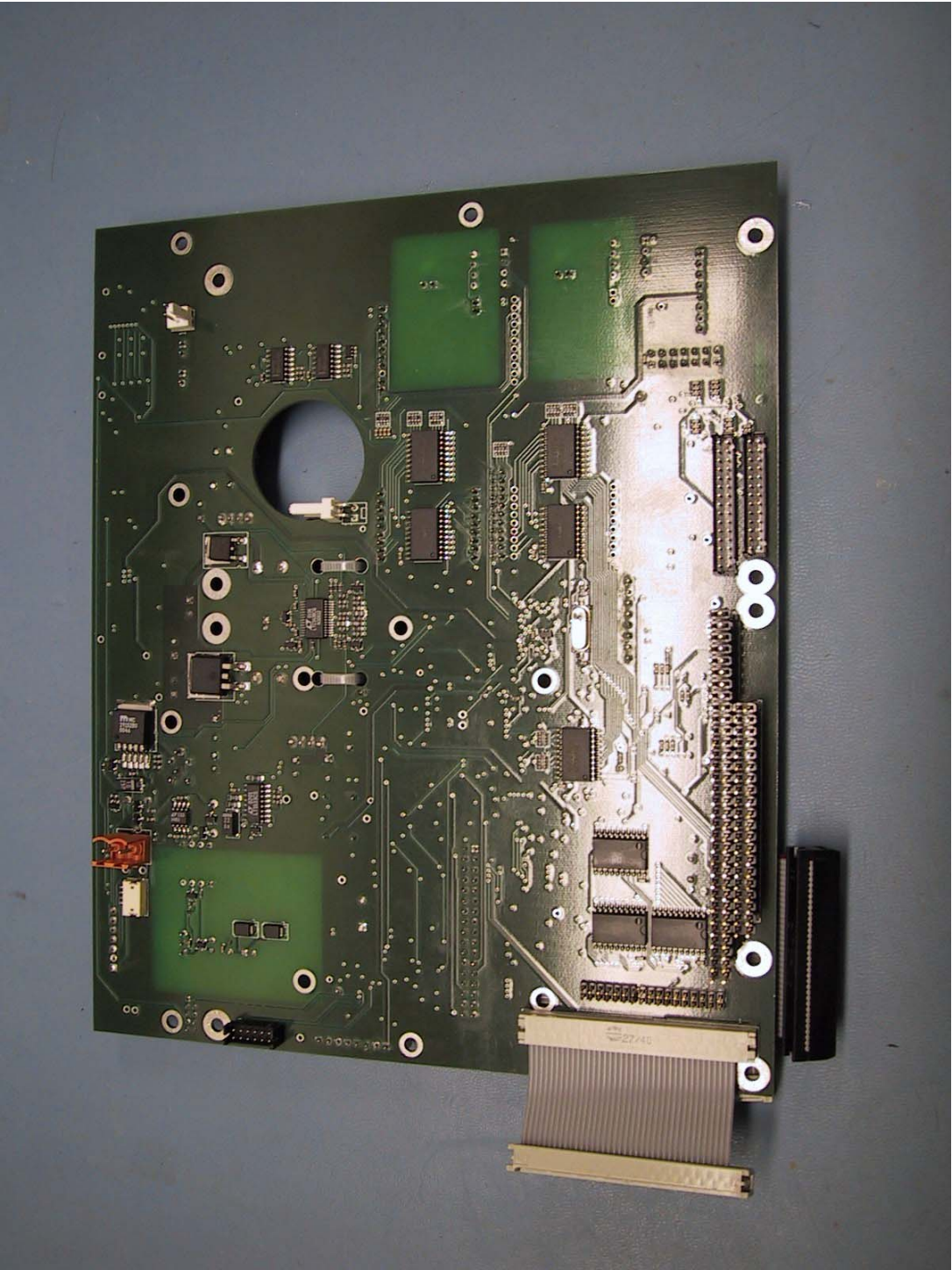
Tempus PCB 2
