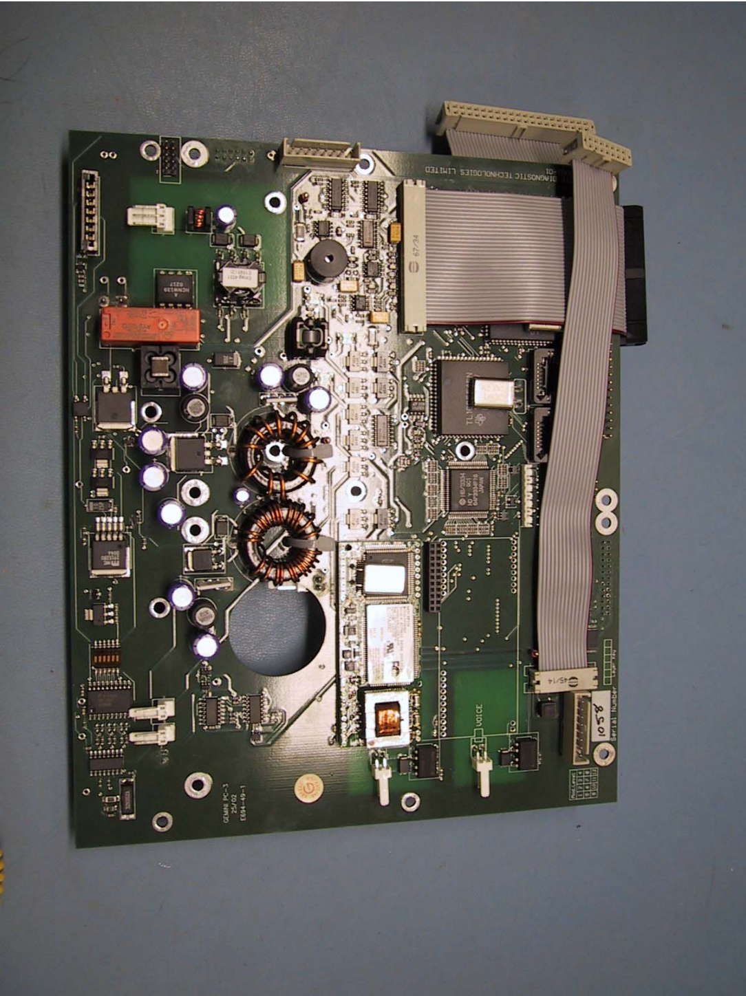
Tempus PCB 1
