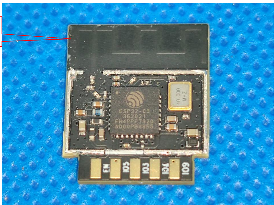
Antenna
