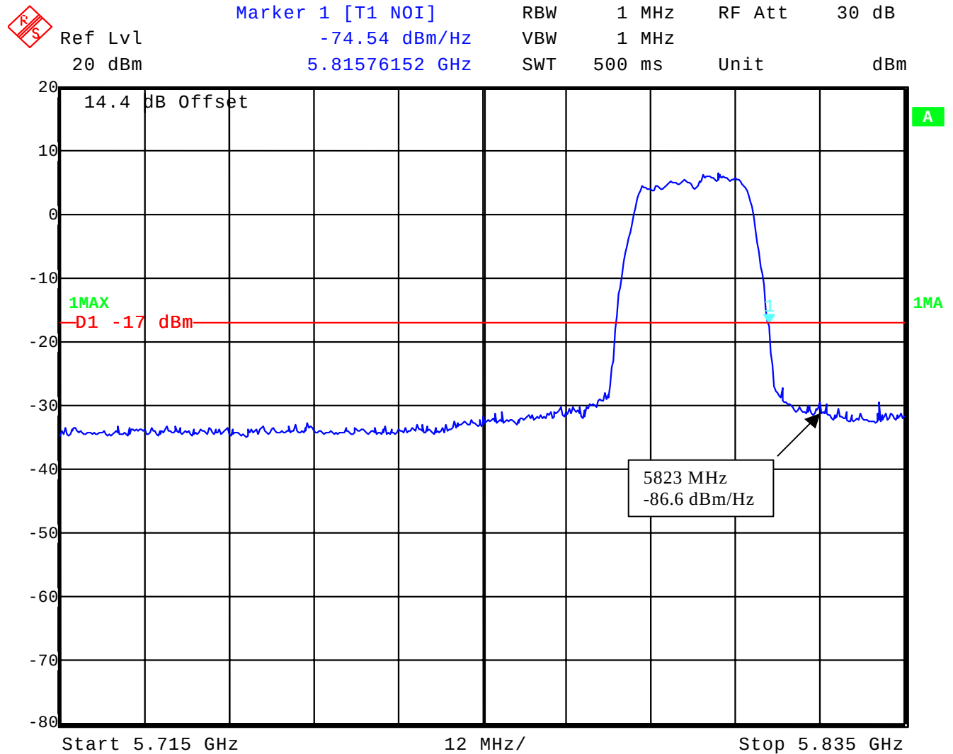
Plot 2: upper band edge
