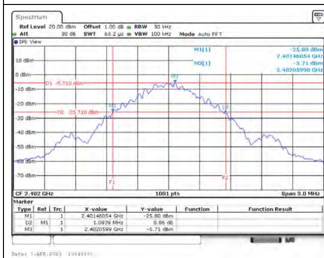
GFSK / 2402 MHz
