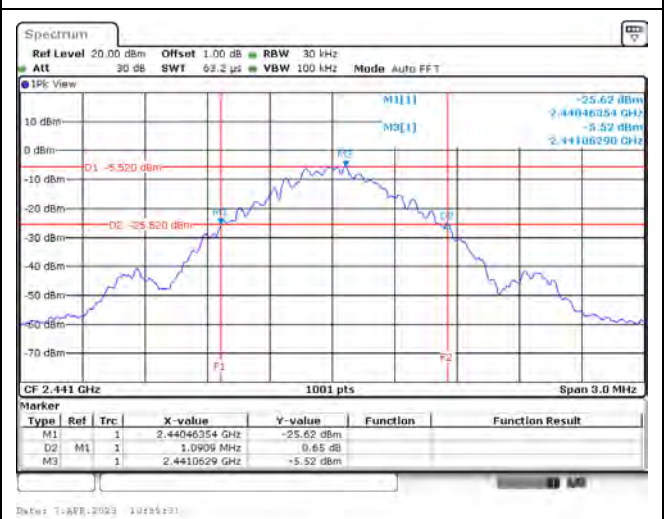
GFSK / 2441 MHz
