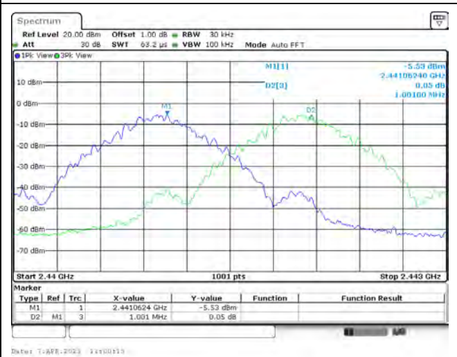
GFSK / 2441 MHz
