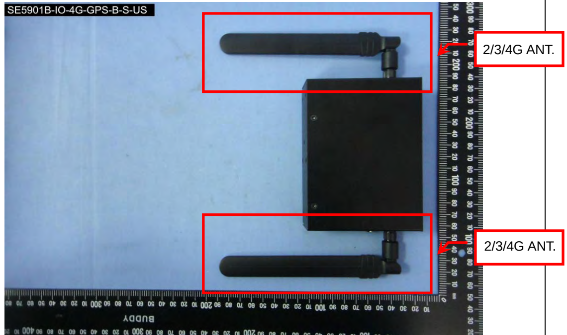
EUT Photo 1 )
