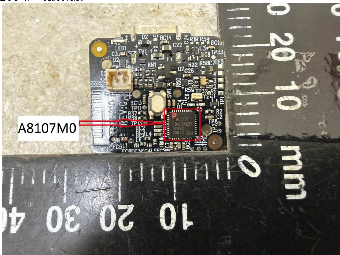
EUT-4. A8107M0
