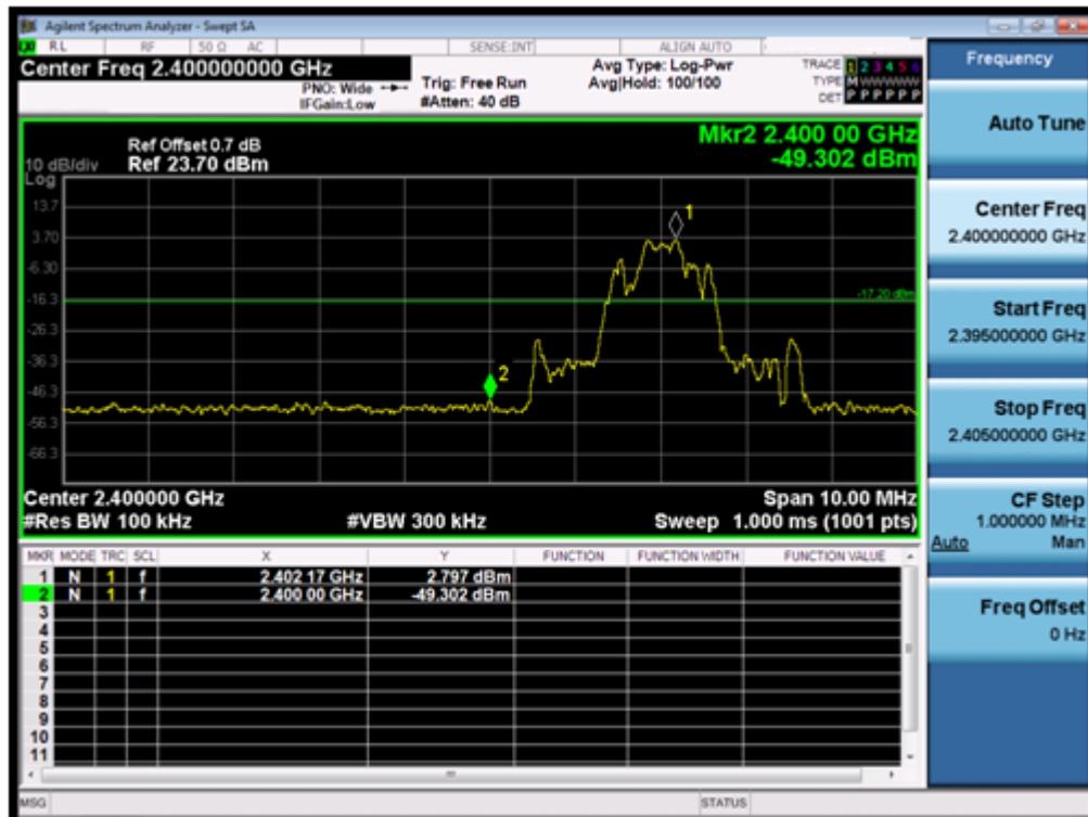
(Plot 4.5.2.3 A: Channel 00: 2402MHz @ \pi/4 DQPSK)
