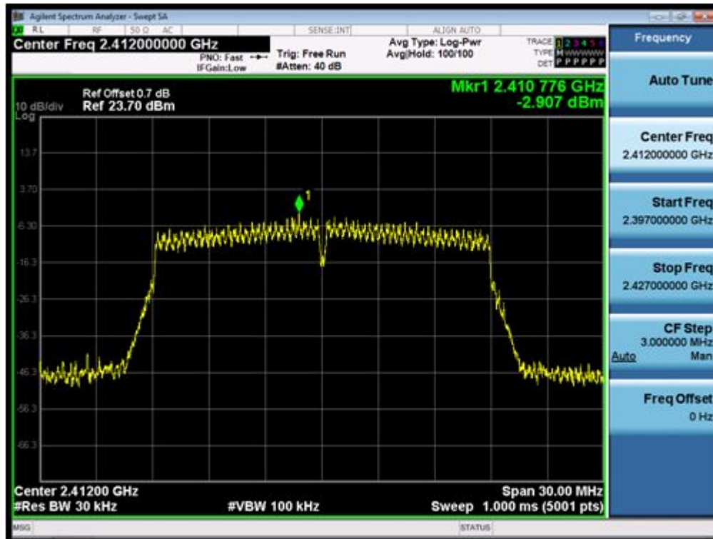
(Plot 4.4.3 A: Channel 1: 2412MHz @ 802.11n HT20)
