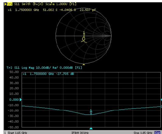
1750MHz Body
