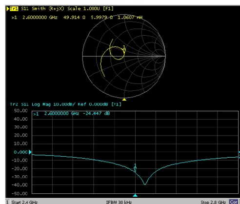
2600MHz Head
