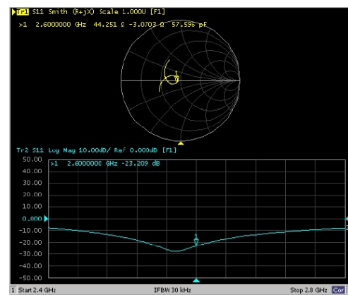
2600MHz Body
