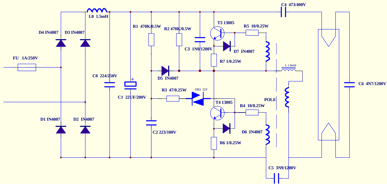
SFU-201线路原理图
