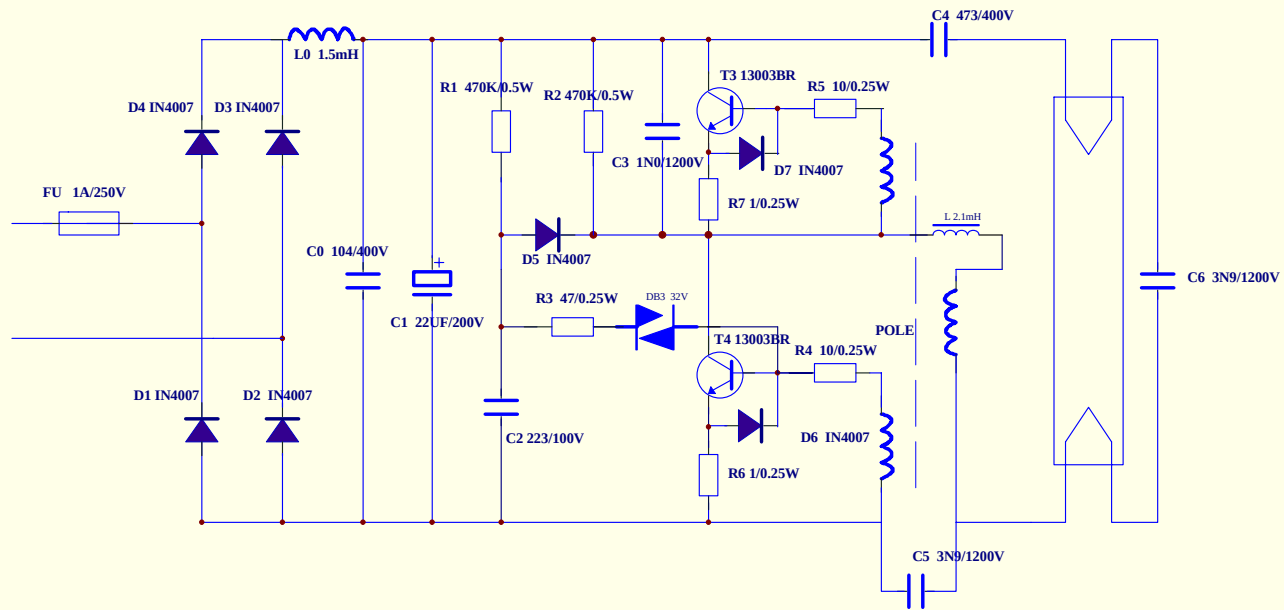
SFS-131\SFU-131线路原理图
