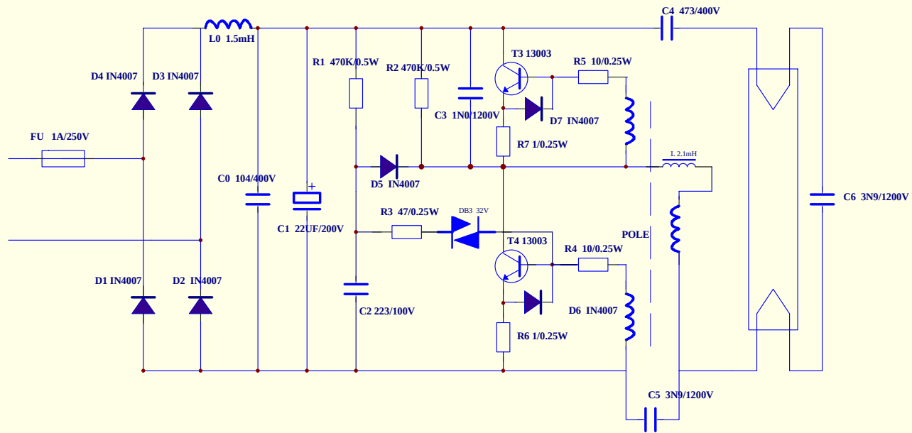
SFS-151线路原理图
