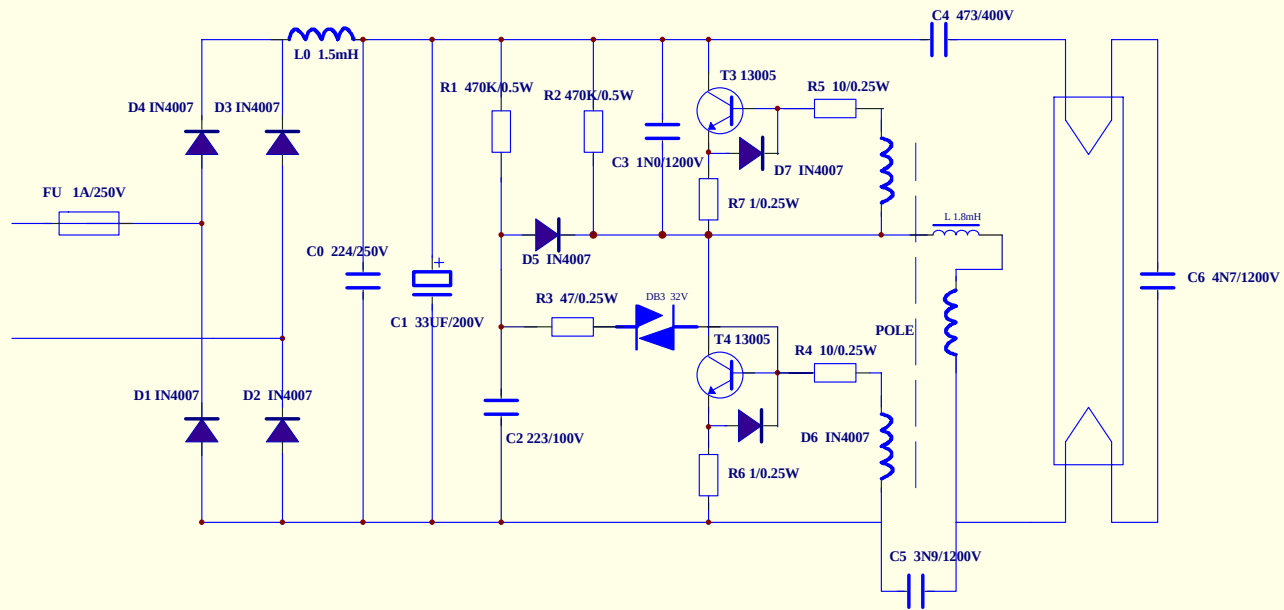
SFS-251线路原理图
