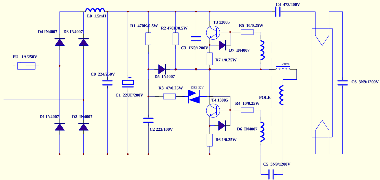
SFS-201线路原理图
