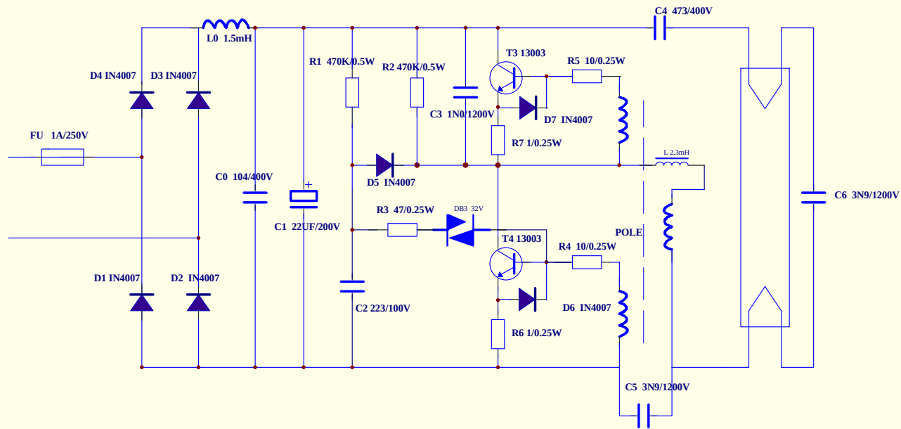
SFU-151线路原理图
