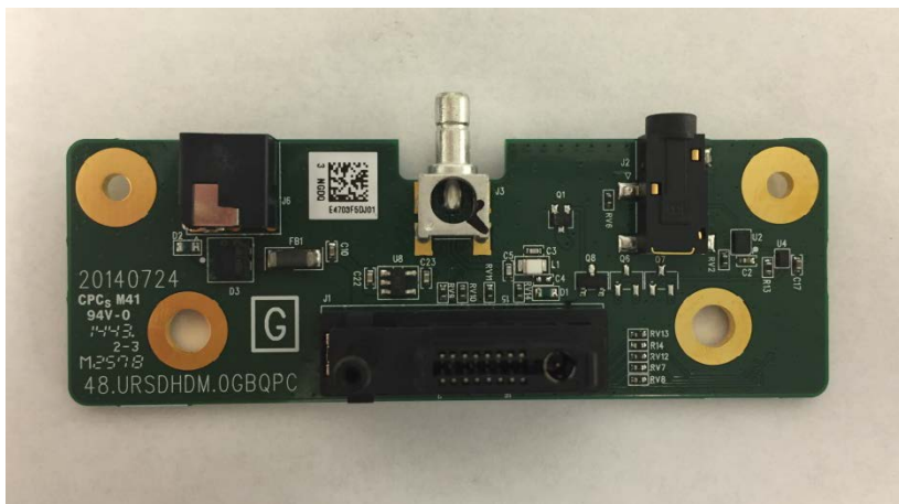
PCBA Top
