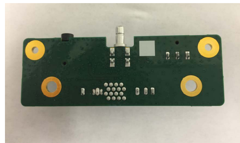
PCBA Bottom
