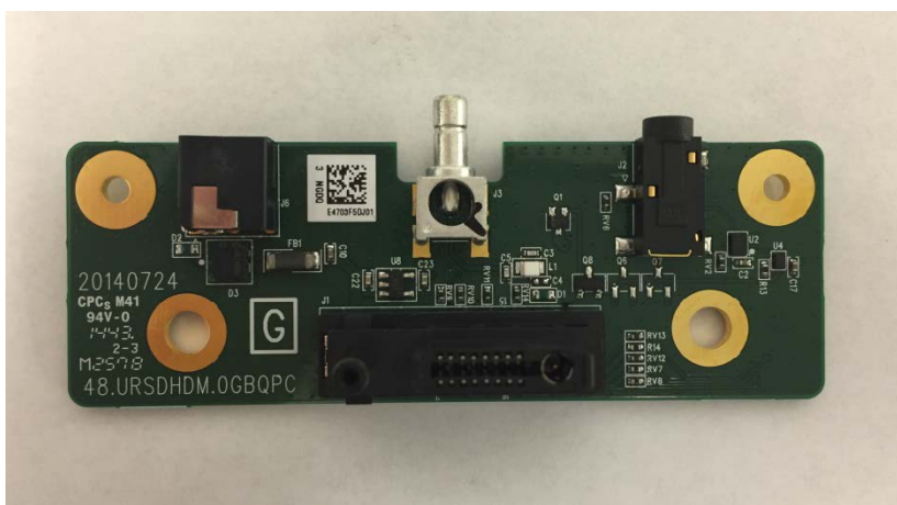
PCBA Top
