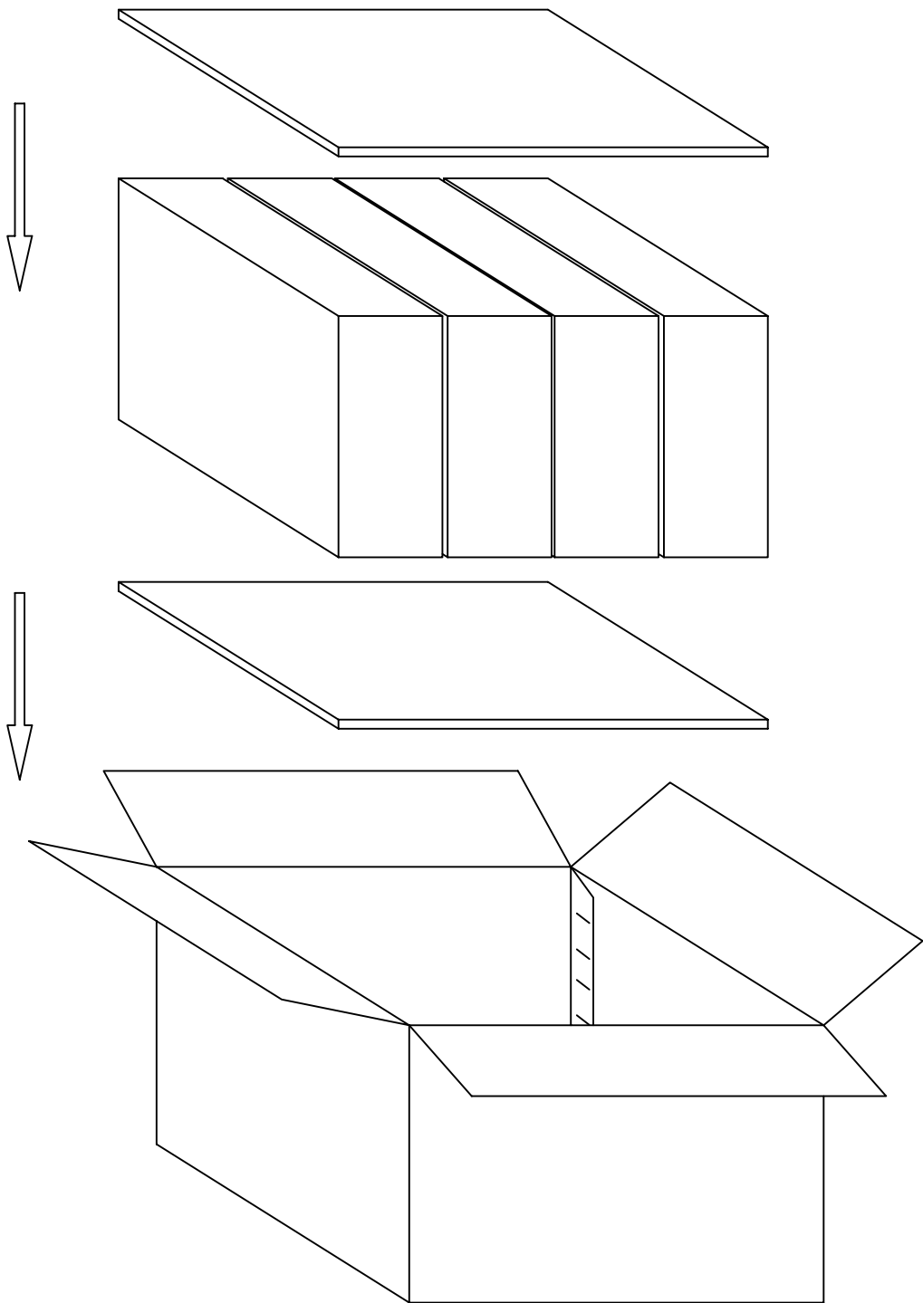
OVERPACK CARTON(KEM-PK17159)
