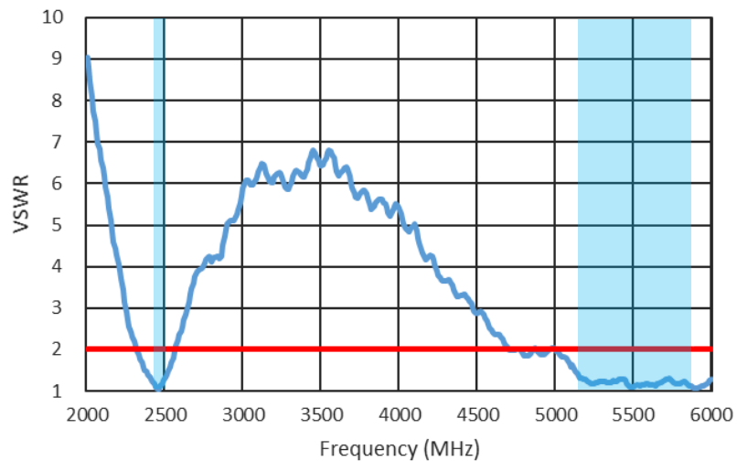
Dual1 VSWR=2
