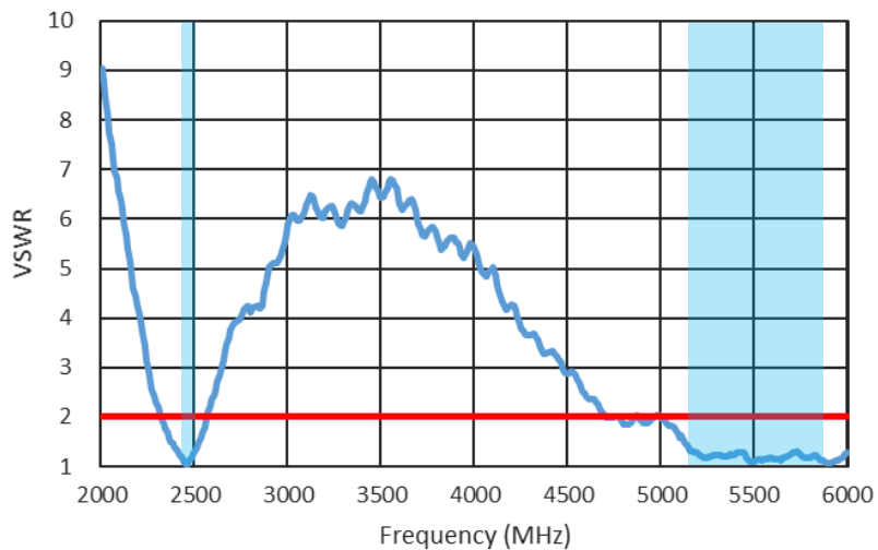
Dual1 VSWR=2
