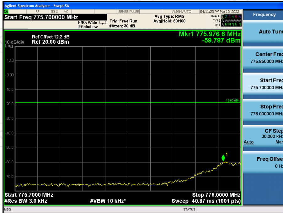
Upper700MHz GSM UL Left Side Pre AGC+10dB
