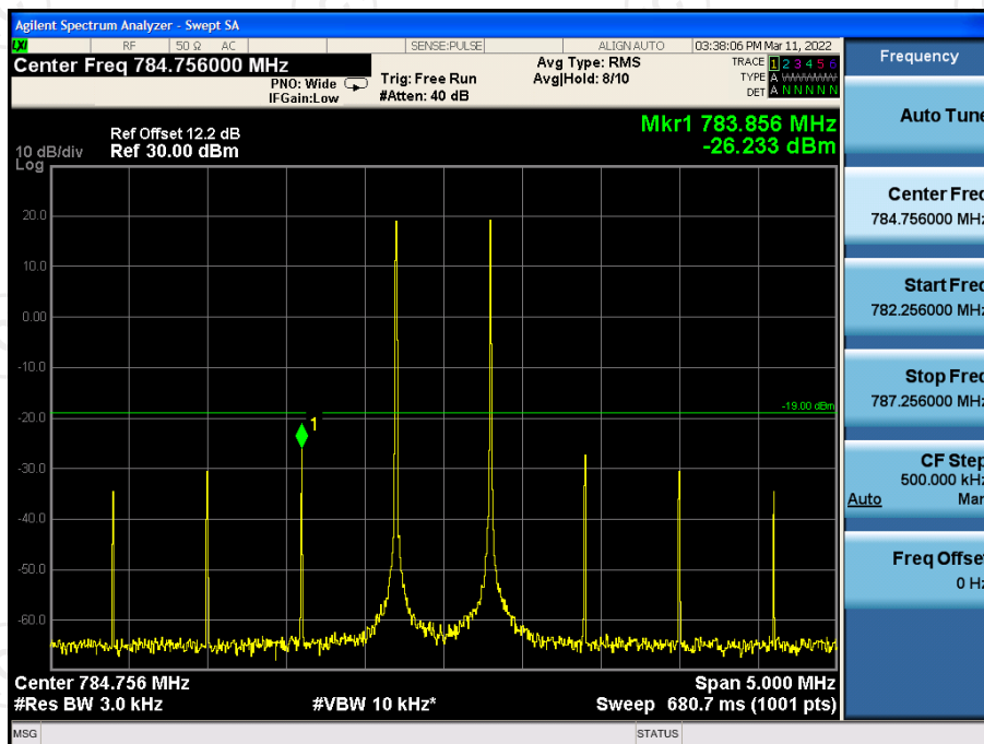
Upper700MHz AGC +10dB , UL
