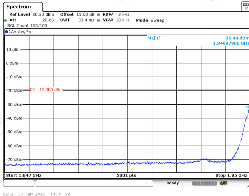
PCS GSM UL Left Side Pre AGC + 10 dB
