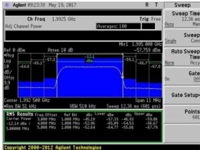
7.5_OBE_DL_1930-1995MHz_H_PreAGC_WCDMA
