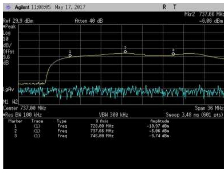
7.1_Band Verify_DL_728-746MHz
