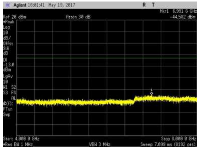
7.6_CSE_DL_728-746MHz_R2
