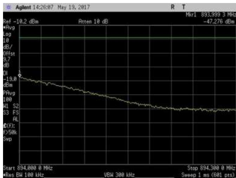
7.5_OBE_DL_869-894MHz_H_PreAGC_LTE
