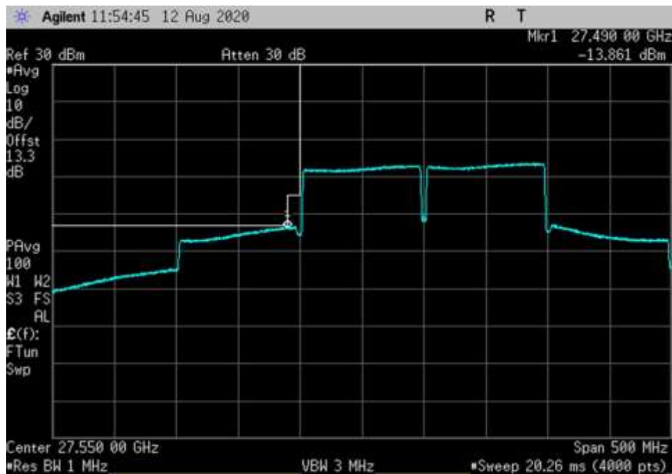
UL_27500-28350-64QAM-100MHz-V-CP OFDM_LC
