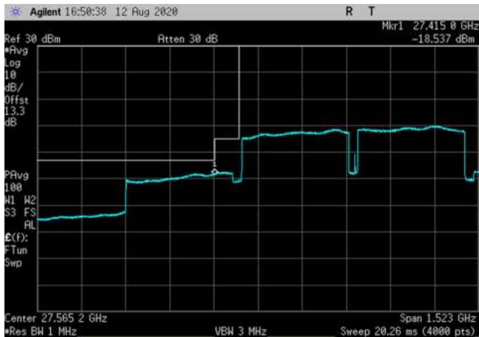
UL_27500-28350-QPSK-400MHz-V-AGC+3-DFT OFDM_LC
