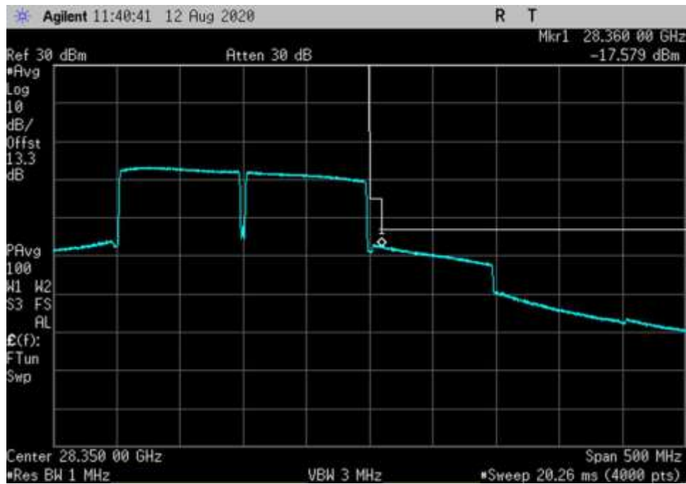
UL_27500-28350-QPSK-100MHz-V-AGC+3-CP OFDM_HC
