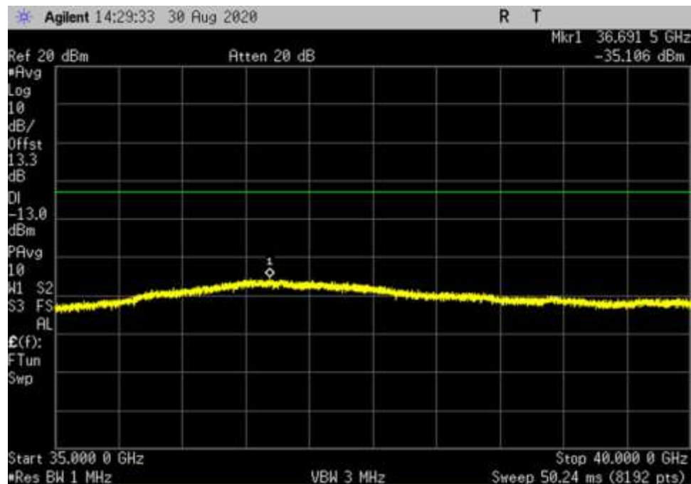
DL_H_256QAM_100MHz_RB1_CP_ 35000- 40000MHz_fo
