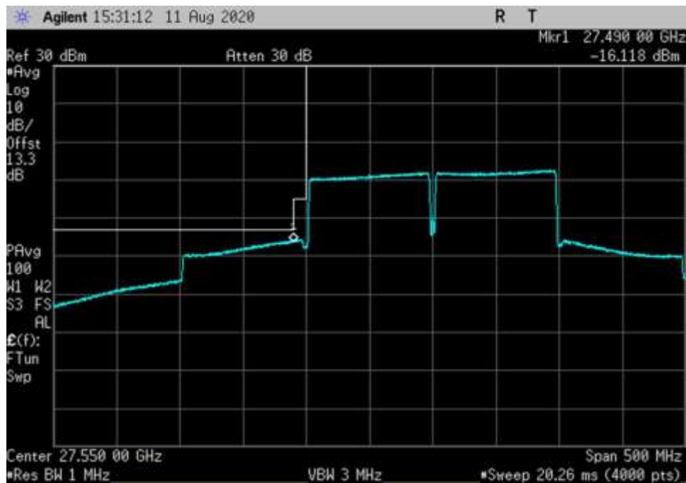
DL_27500-28350-256QAM-100MHz-V-CP OFDM_LC
