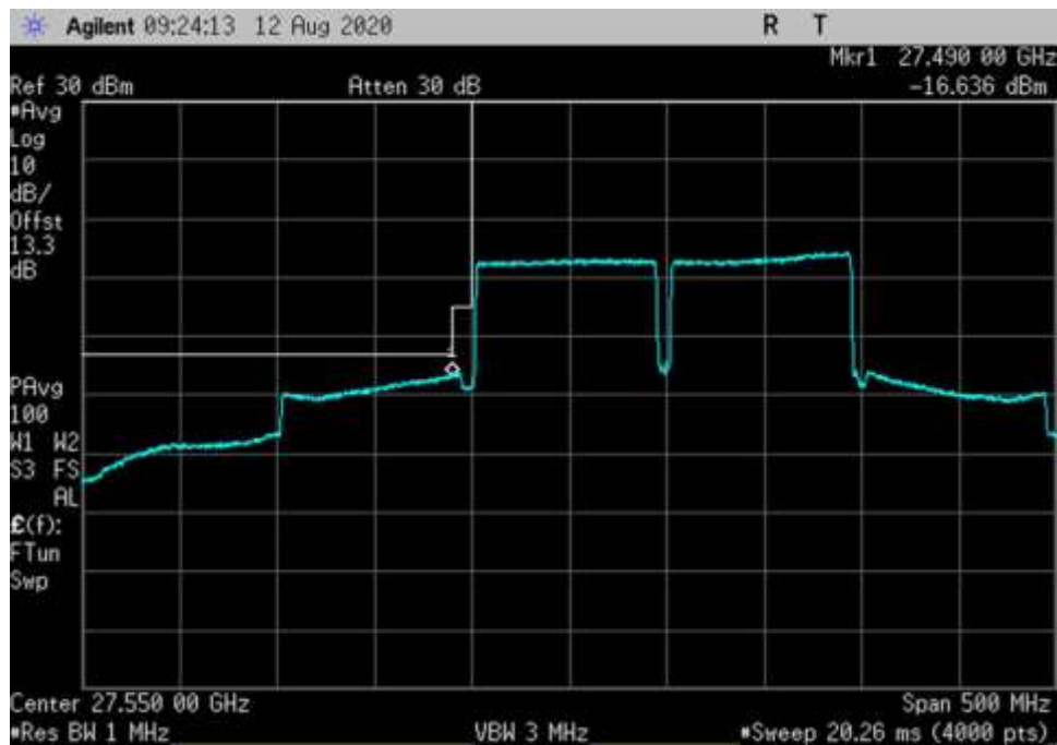
UL_27500-28350-QPSK-100MHz-H-AGC+3-DFT OFDM_LC
