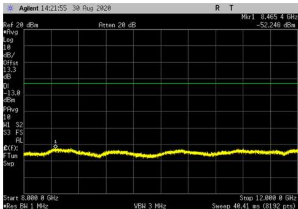
DL_H_16QAM_100MHz_RB1_CP_ 8000- 12000MHz_fo
