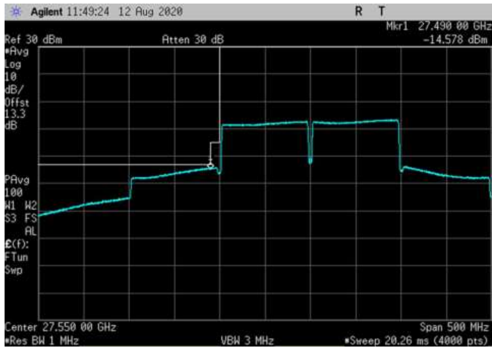
UL_27500-28350-16QAM-100MHz-V-AGC+3-CP OFDM_LC
