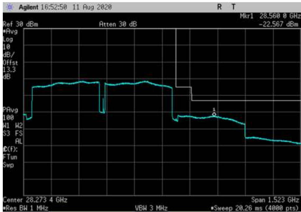
UL_27500-28350-QPSK-400MHz-H-DFT OFDM_HC
