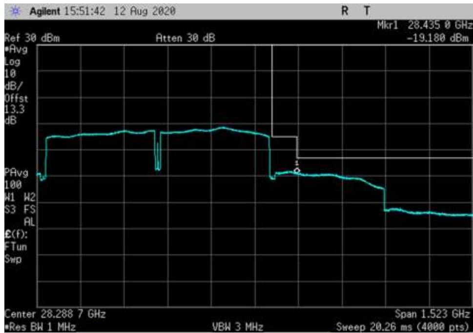
UL_27500-28350-QPSK-400MHz-V-AGC+3-CP OFDM_HC
