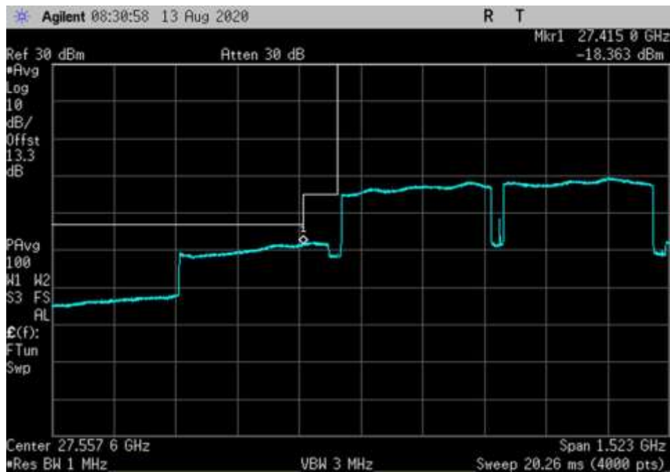
UL_27500-28350-64QAM-400MHz-V-DFT OFDM_LC
