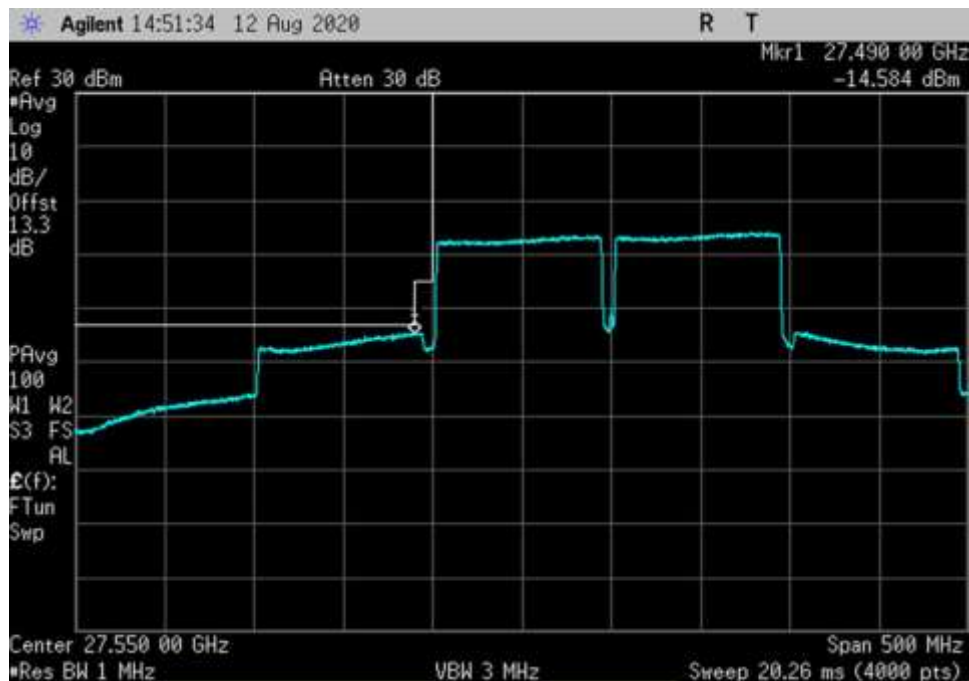
UL_27500-28350-64QAM-100MHz-V-DFT OFDM_LC
