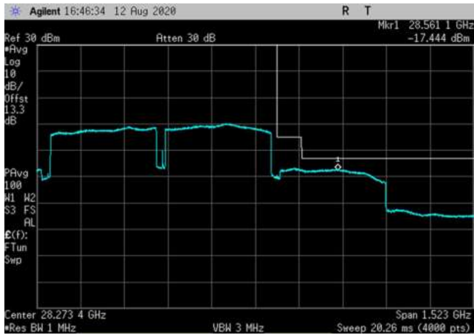
UL_27500-28350-QPSK-400MHz-V-AGC+3-DFT OFDM_HC
