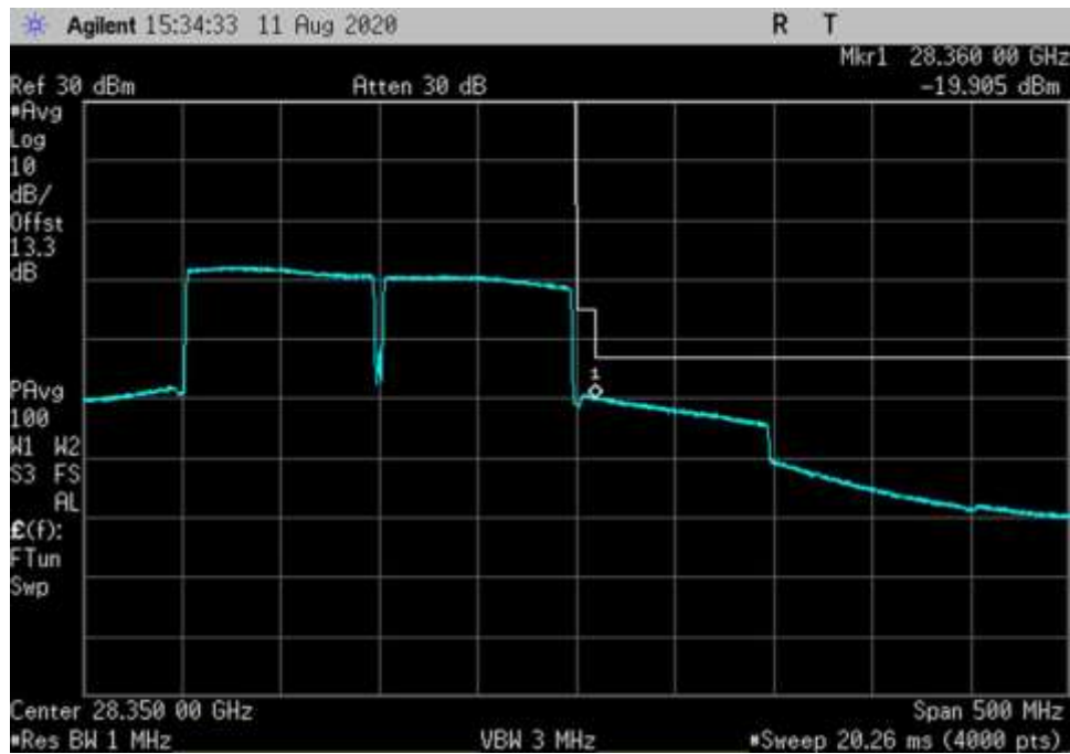
DL_27500-28350-256QAM-100MHz-V-AGC+3-CP OFDM_HC
