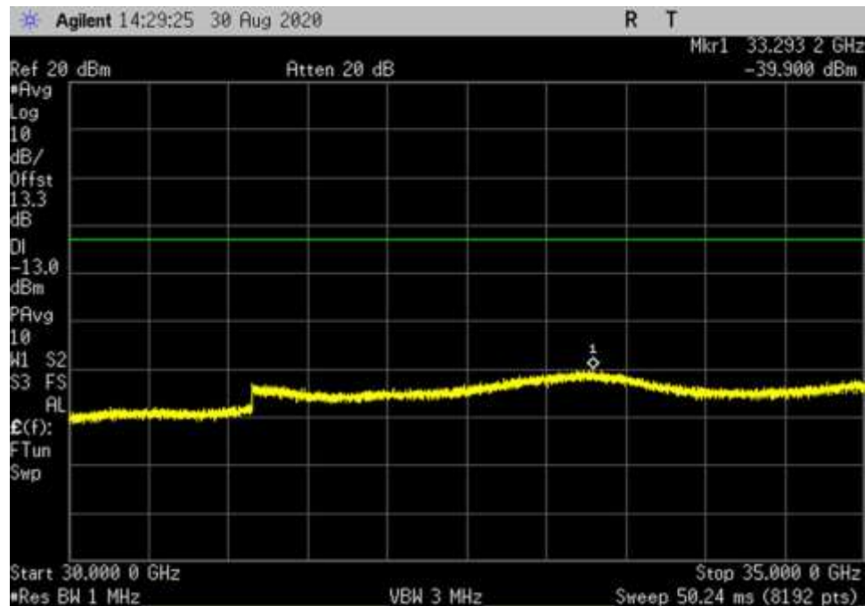
DL_H_256QAM_100MHz_RB1_CP_ 30000- 35000MHz_fo
