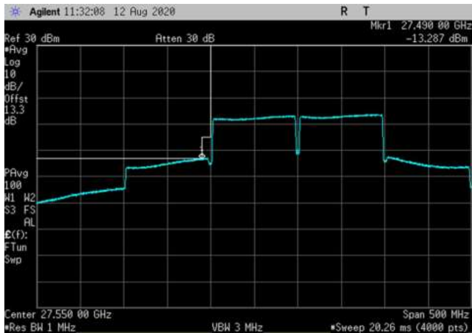
UL_27500-28350-QPSK-100MHz-V-CP OFDM_LC
