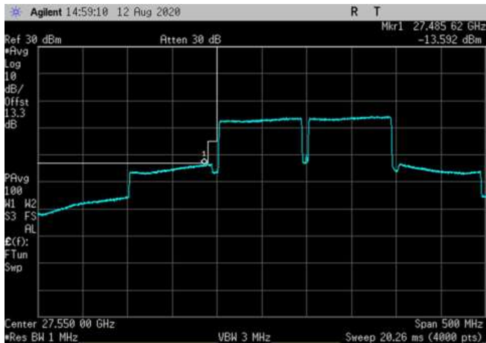
UL_27500-28350-256QAM-100MHz-V-AGC+3-DFT OFDM_LC
