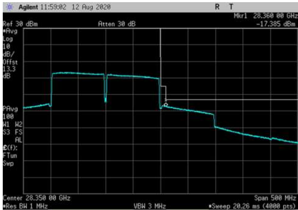
UL_27500-28350-64QAM-100MHz-V-CP OFDM_HC
