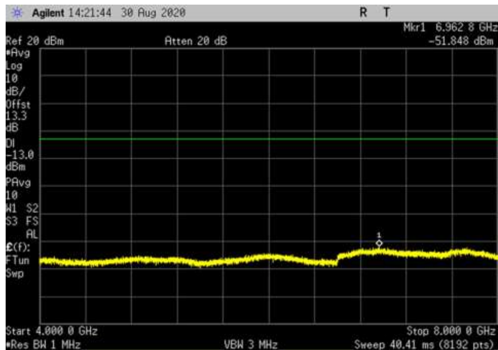
DL_H_16QAM_100MHz_RB1_CP_ 4000- 8000MHz_fo
