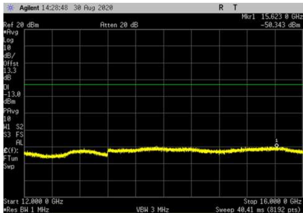
DL_H_256QAM_100MHz_RB1_CP_12000-16000MHz_fo
