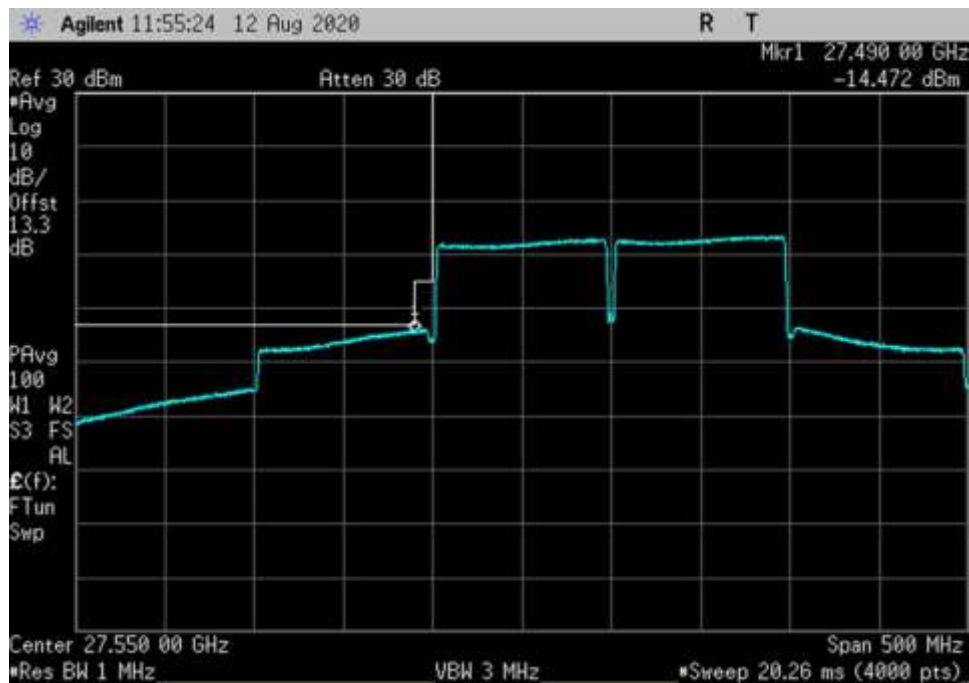
UL_27500-28350-64QAM-100MHz-V-AGC+3-CP OFDM_LC
