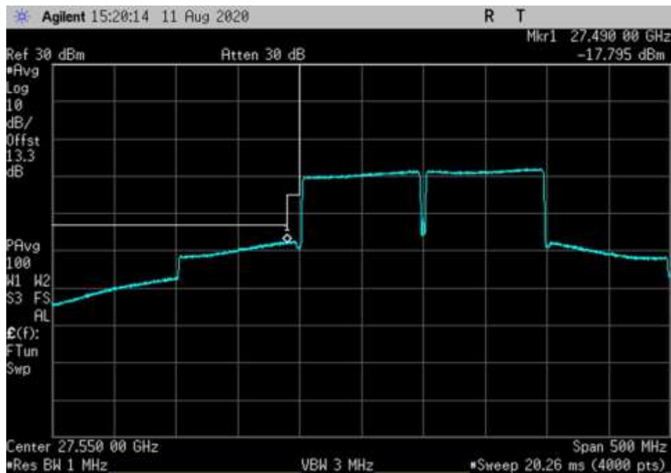
DL_27500-28350-64QAM-100MHz-V-CP OFDM_LC
