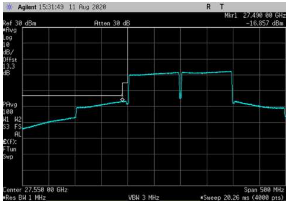
DL_27500-28350-256QAM-100MHz-V-AGC+3-CP OFDM_LC
