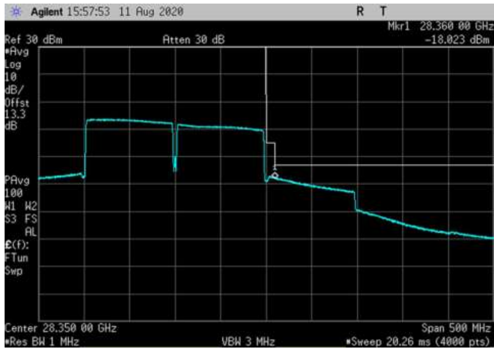
DL_27500-28350-QPSK-100MHz-H-CP OFDM_HC
