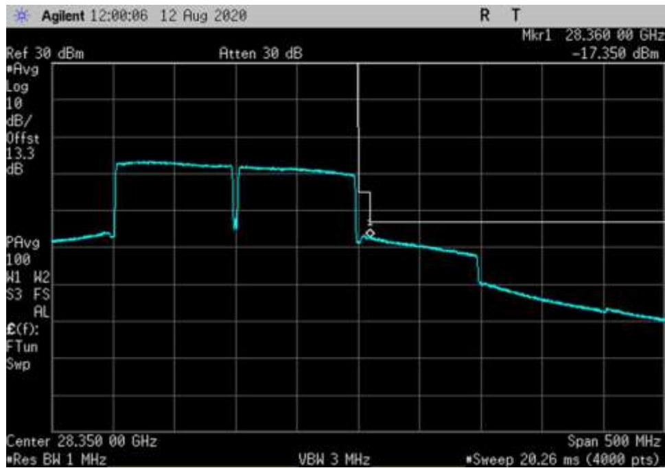
UL_27500-28350-64QAM-100MHz-V-AGC+3-CP OFDM_HC
