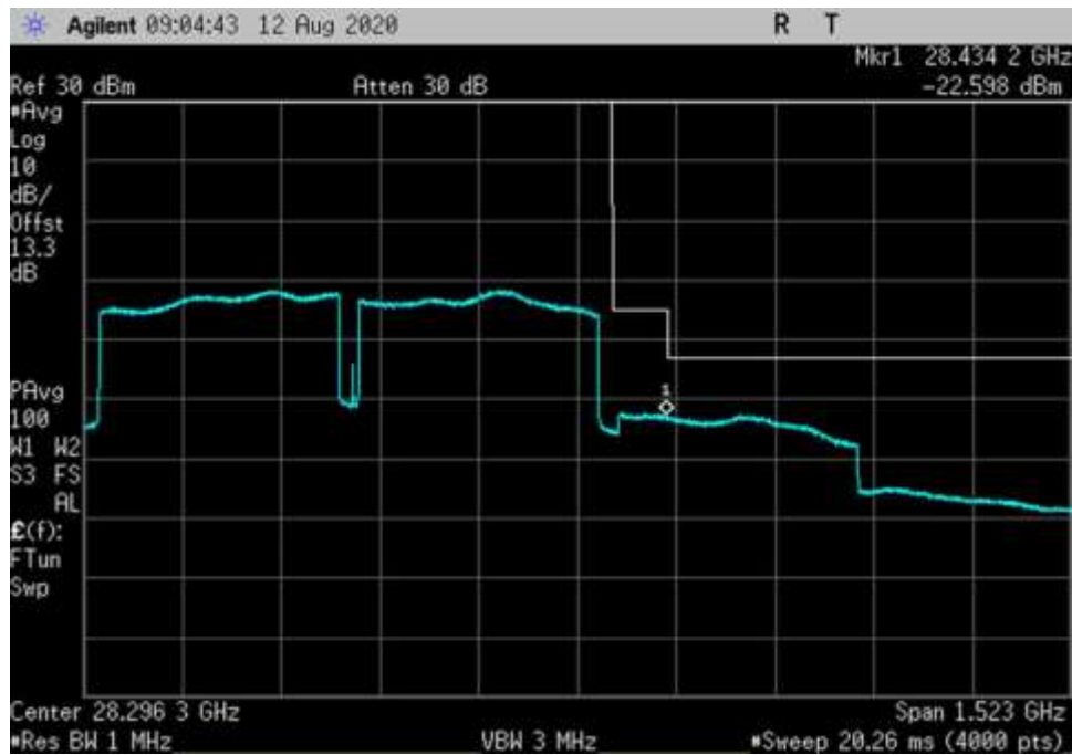
UL_27500-28350-256QAM-400MHz-H-DFT OFDM_HC
