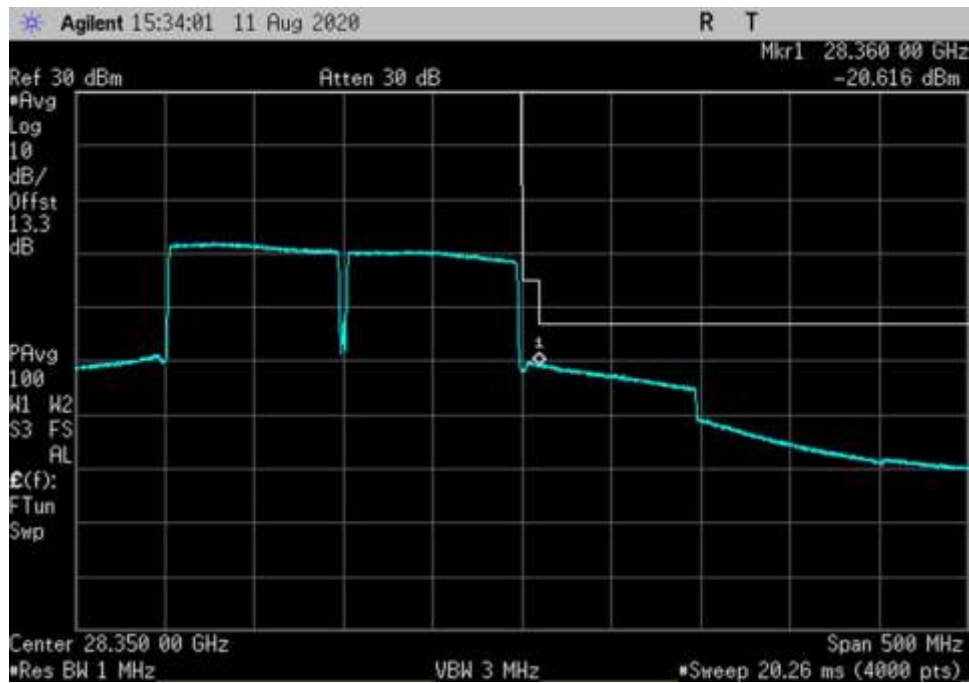
DL_27500-28350-256QAM-100MHz-V-CP OFDM_HC
