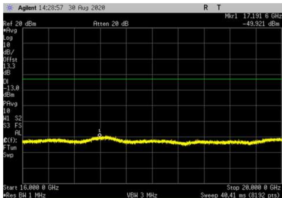
DL_H_256QAM_100MHz_RB1_CP_16000-20000MHz_fo
