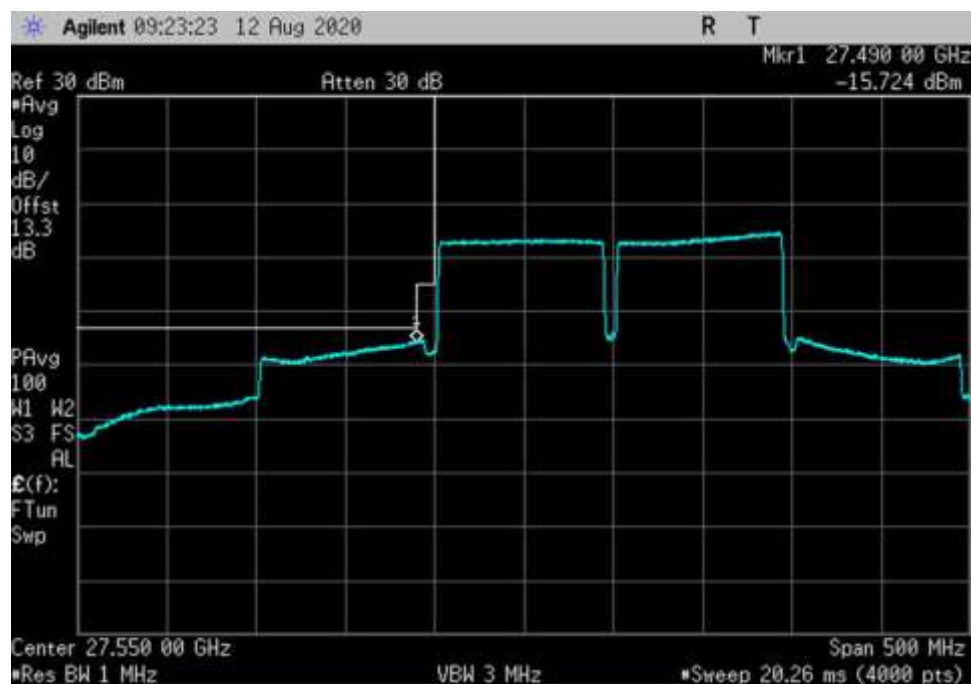
UL_27500-28350-QPSK-100MHz-H-DFT OFDM_LC
