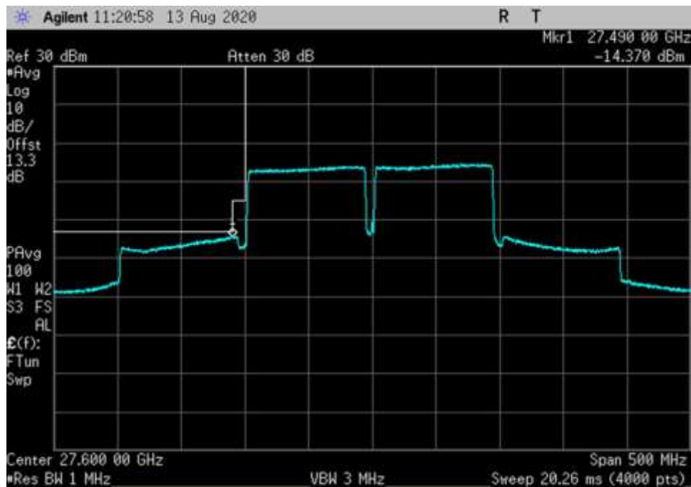
UL_27500-28350-QPSK-100MHz-V-AGC+3-DFT OFDM_LC
