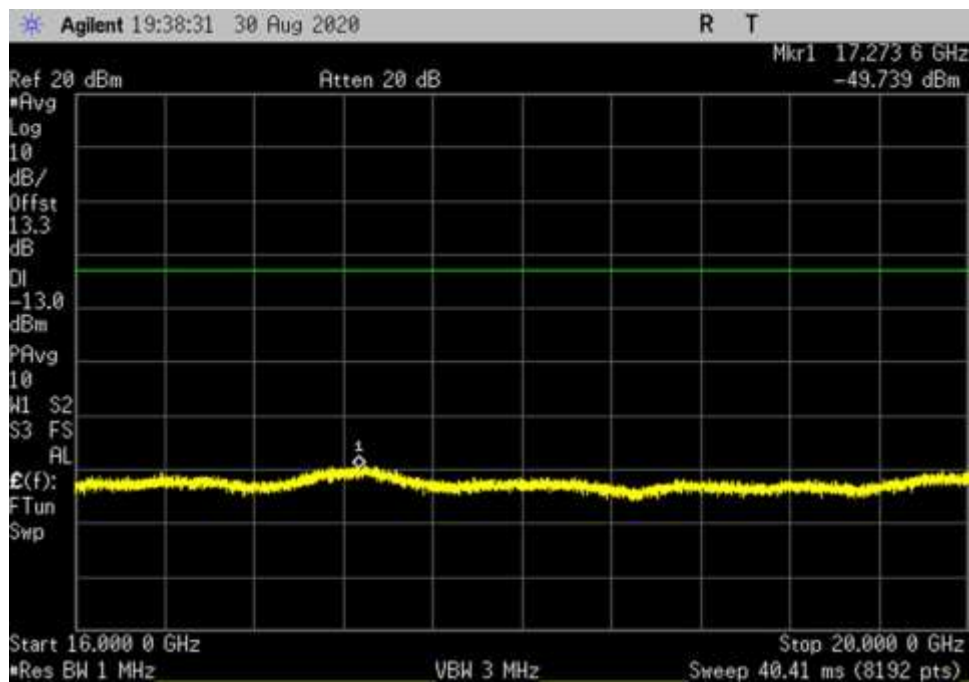
UL_V_QPSK_400MHz_Full_DFT_16000-20000MHz_fo
