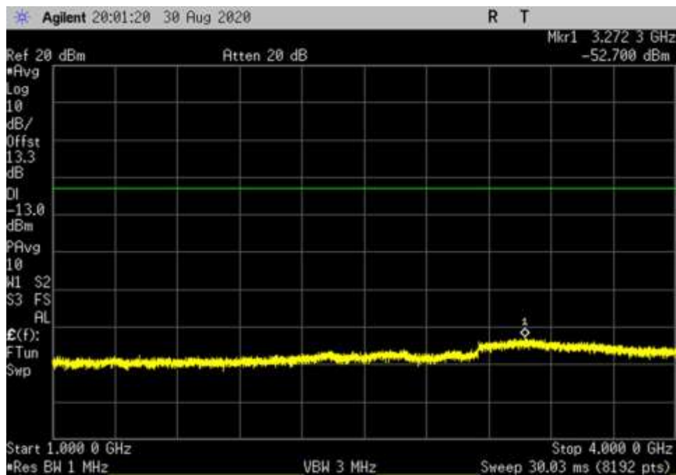
UL_V_256QAM_400MHz_RB1_DFT_1000-4000MHz_fo
