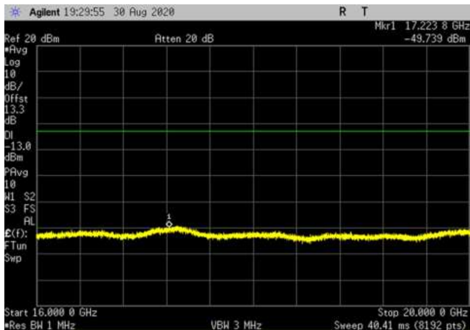
UL_V_256QAM_100MHz_RB1_DFT_16000-20000MHz_fo
