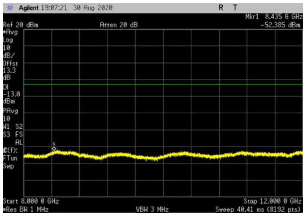
UL_V_QPSK_100MHz_Full_DFT_8000- 12000MHz_fo
