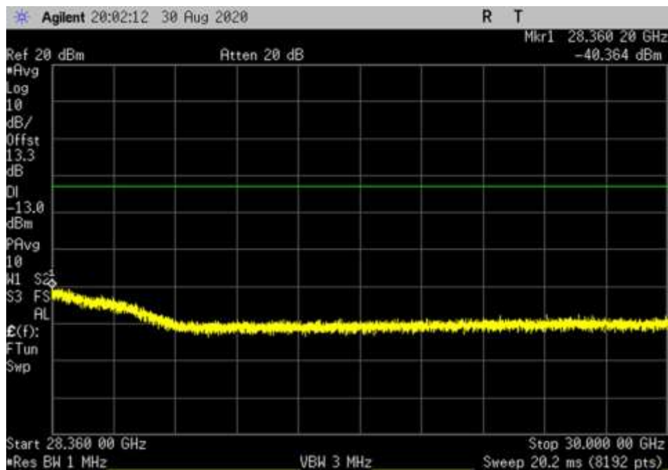
UL_V_256QAM_400MHz_RB1_DFT_28360-30000MHz_fo
