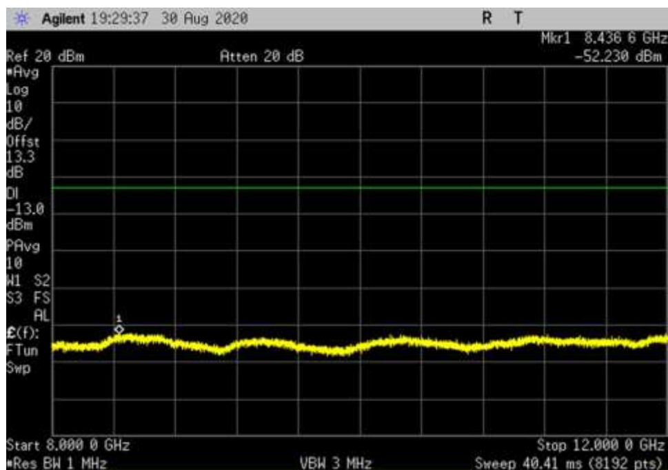
UL_V_256QAM_100MHz_RB1_DFT_8000- 12000MHz_fo
