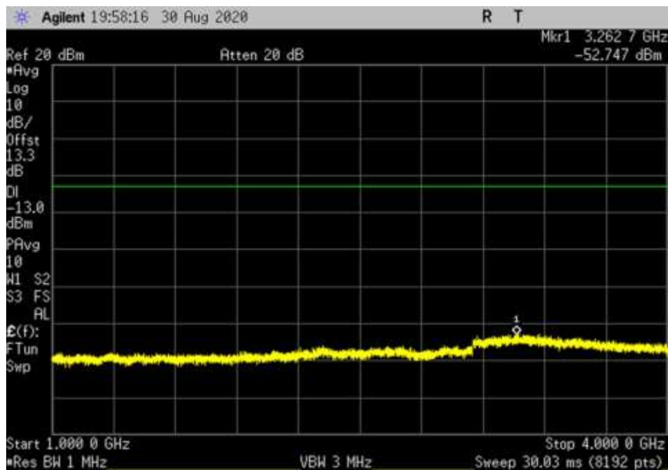
UL_V_64QAM_400MHz_RB1_DFT_1000-4000MHz_fo
