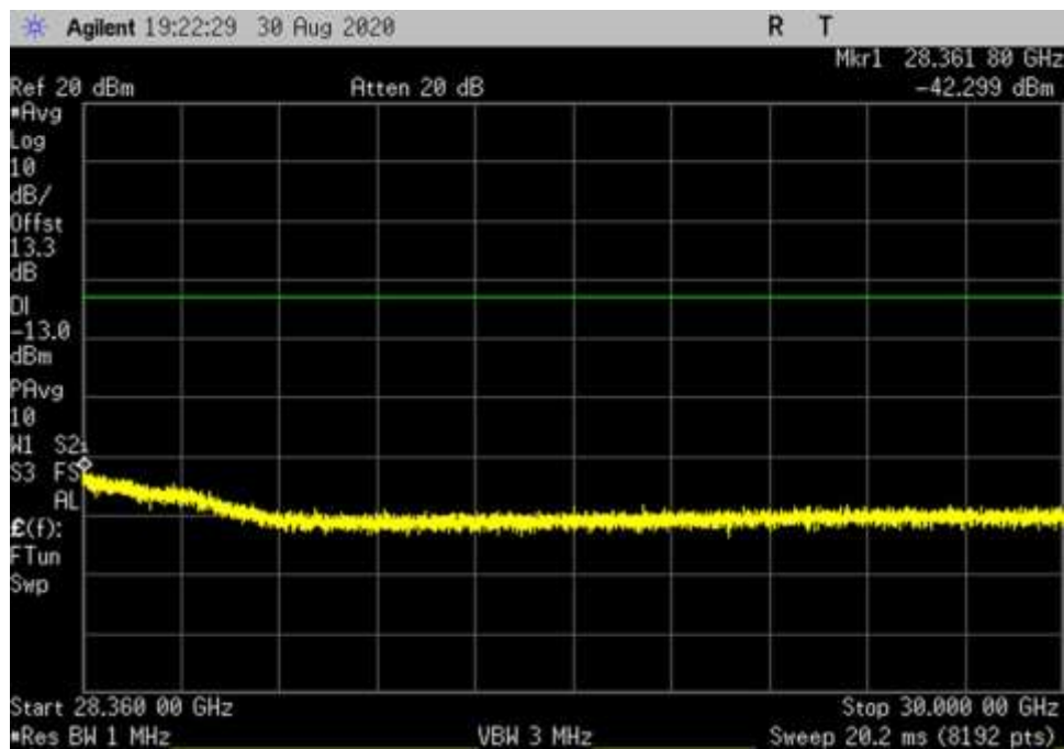
UL_V_QPSK_100MHz_RB1_DFT_28360-30000MHz_fo
