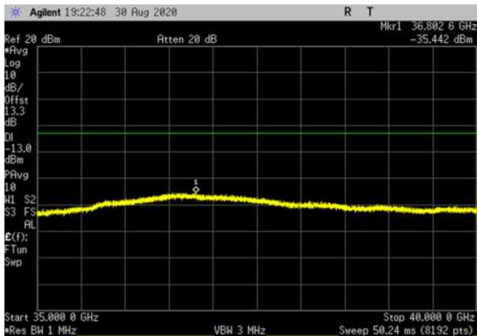
UL_V_QPSK_100MHz_RB1_DFT_35000-40000MHz_fo
