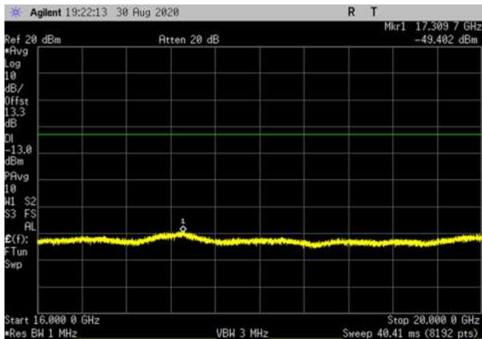
UL_V_QPSK_100MHz_RB1_DFT_16000-20000MHz_fo
