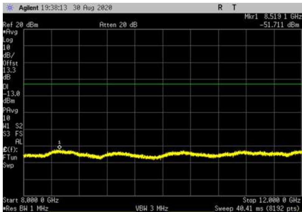
UL_V_QPSK_400MHz_Full_DFT_8000- 12000MHz_fo
