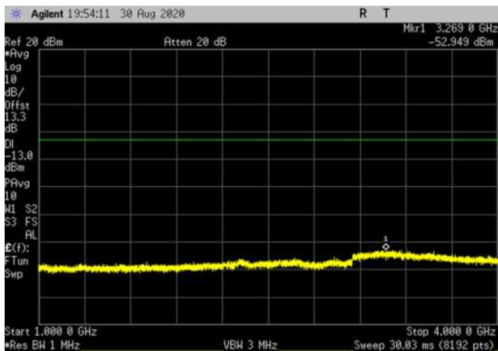
UL_V_QPSK_400MHz_RB1_DFT_1000-4000MHz_fo
