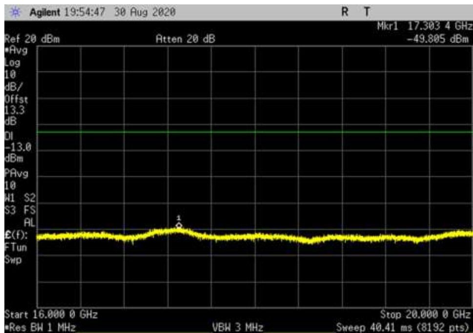
UL_V_QPSK_400MHz_RB1_DFT_16000-20000MHz_fo
