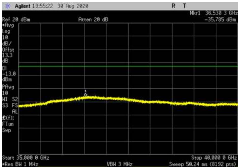
UL_V_QPSK_400MHz_RB1_DFT_35000-40000MHz_fo
