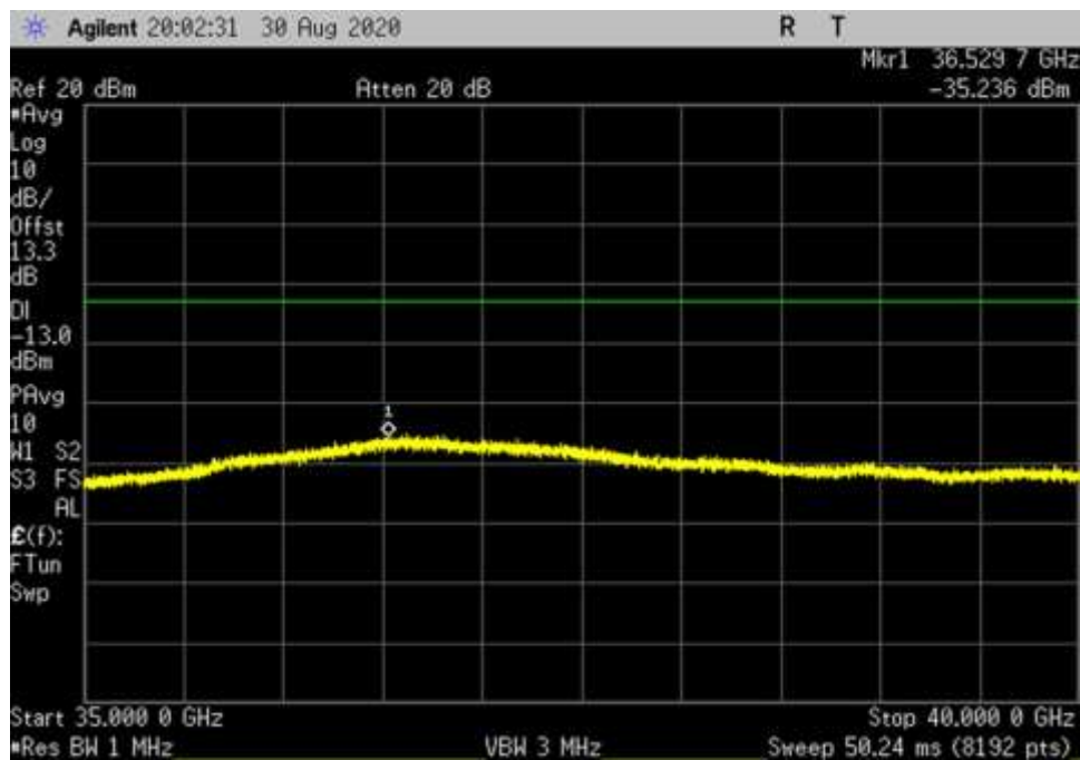
UL_V_256QAM_400MHz_RB1_DFT_35000-40000MHz_fo
