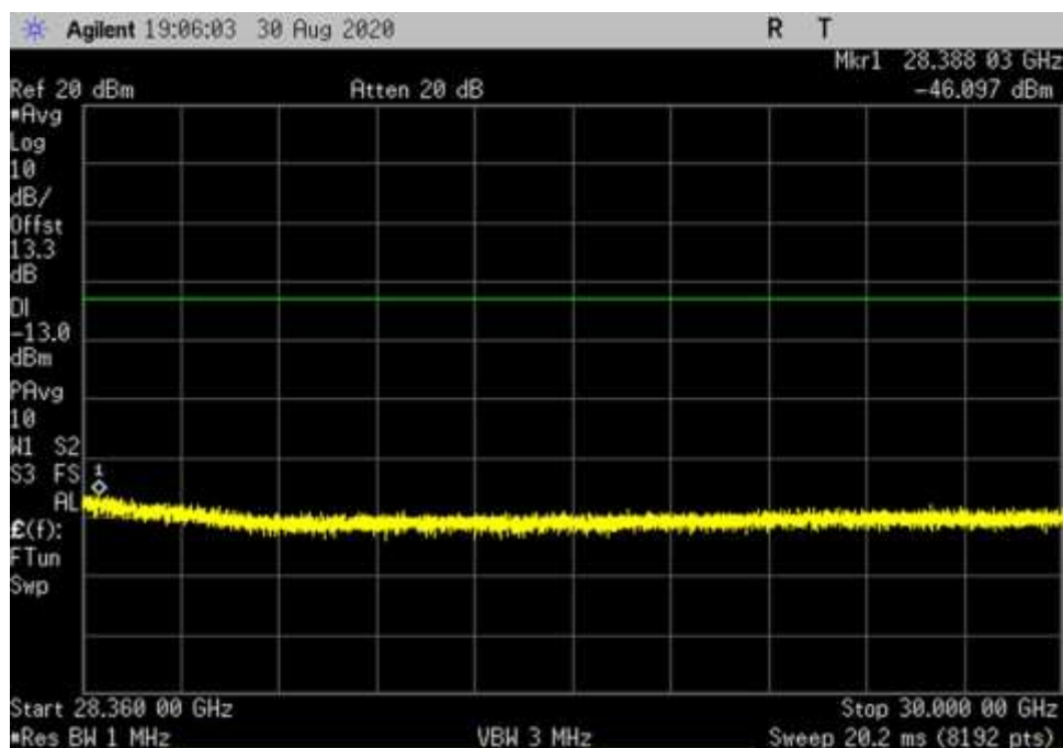
UL_V_Pi/2- BPSK_100MHz_Full_DFT_ 28360- 30000MHz_fo
