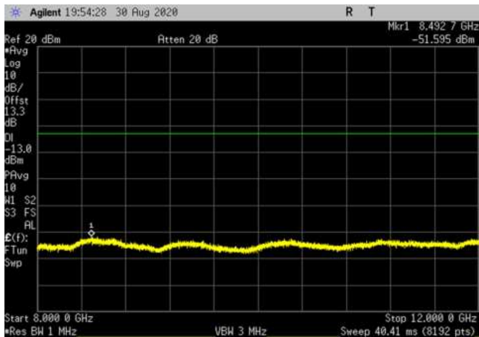
UL_V_QPSK_400MHz_RB1_DFT_8000-12000MHz_fo
