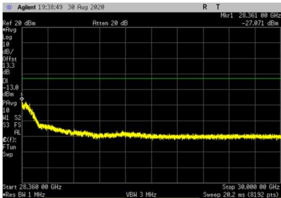
UL_V_QPSK_400MHz_Full_DFT_28360-30000MHz_fo
