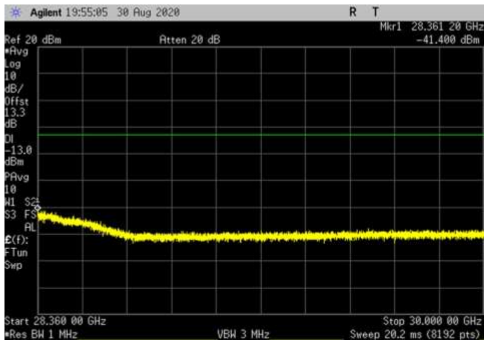
UL_V_QPSK_400MHz_RB1_DFT_28360-30000MHz_fo
