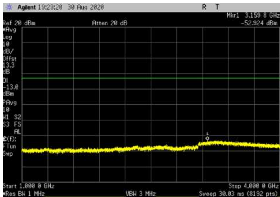
UL_V_256QAM_100MHz_RB1_DFT_1000-4000MHz_fo
