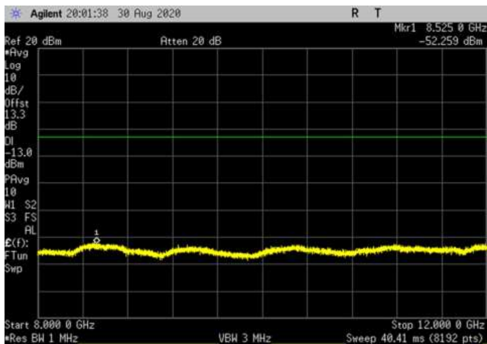
UL_V_256QAM_400MHz_RB1_DFT_8000- 12000MHz_fo
