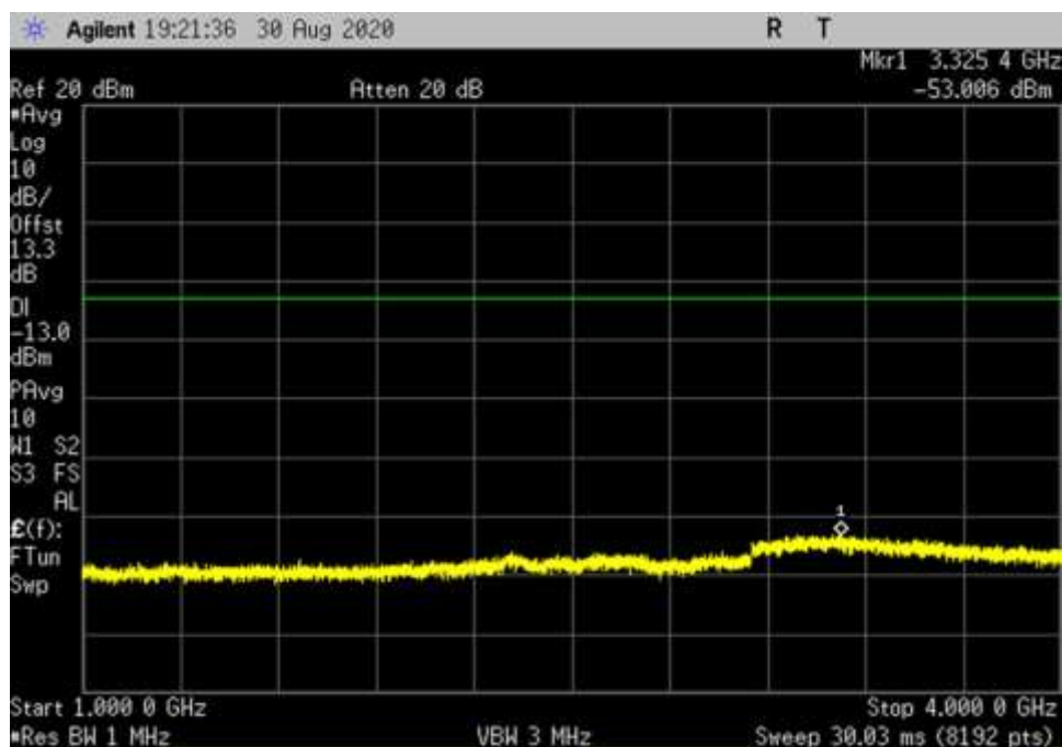
UL_V_QPSK_100MHz_RB1_DFT_1000-4000MHz_fo
