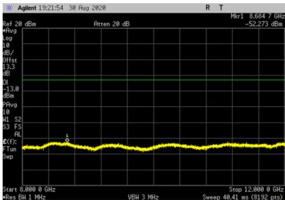
UL_V_QPSK_100MHz_RB1_DFT_8000-12000MHz_fo
