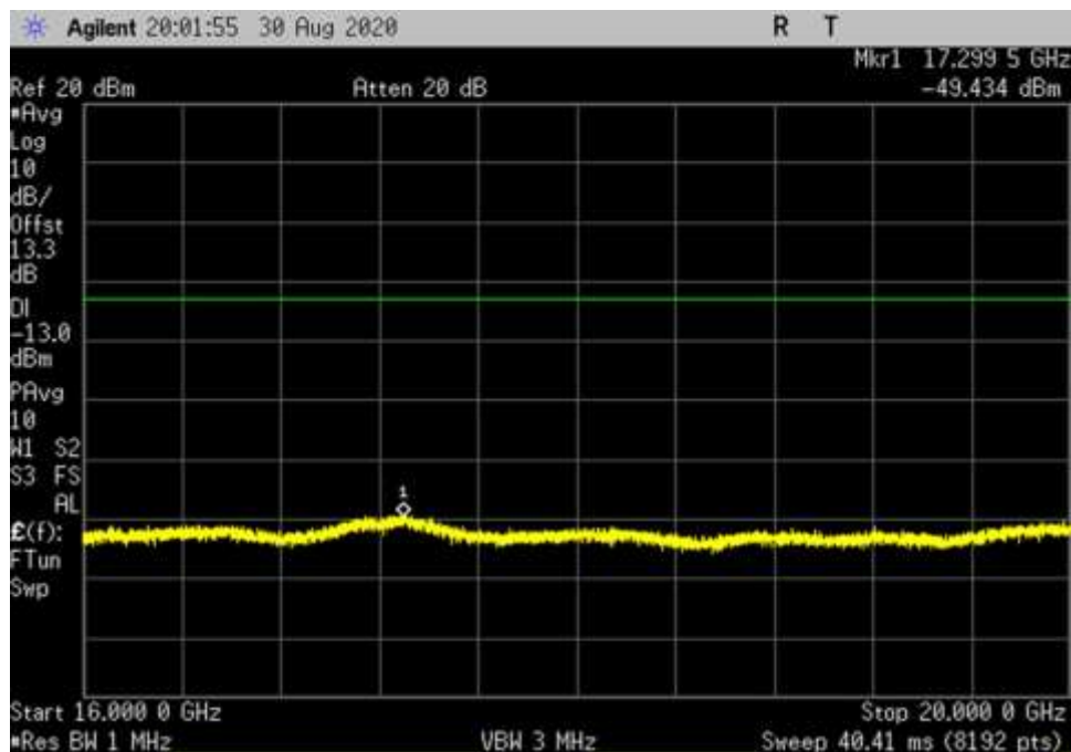
UL_V_256QAM_400MHz_RB1_DFT_16000-20000MHz_fo
