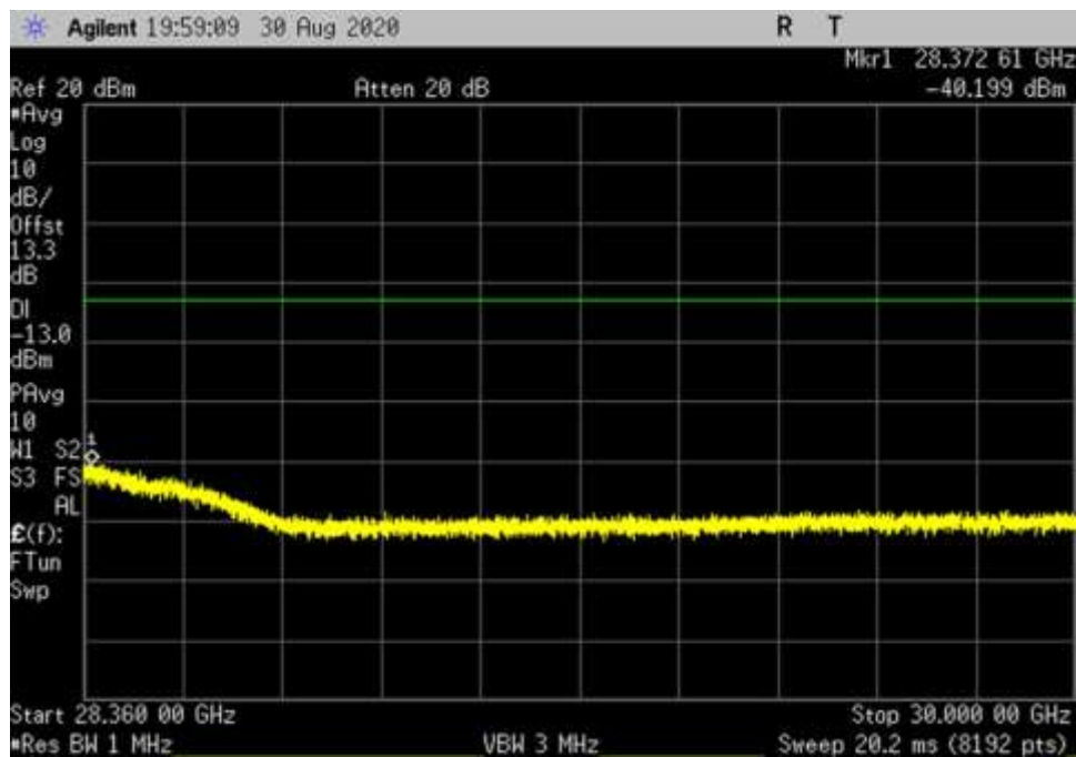
UL_V_64QAM_400MHz_RB1_DFT_28360-30000MHz_fo
