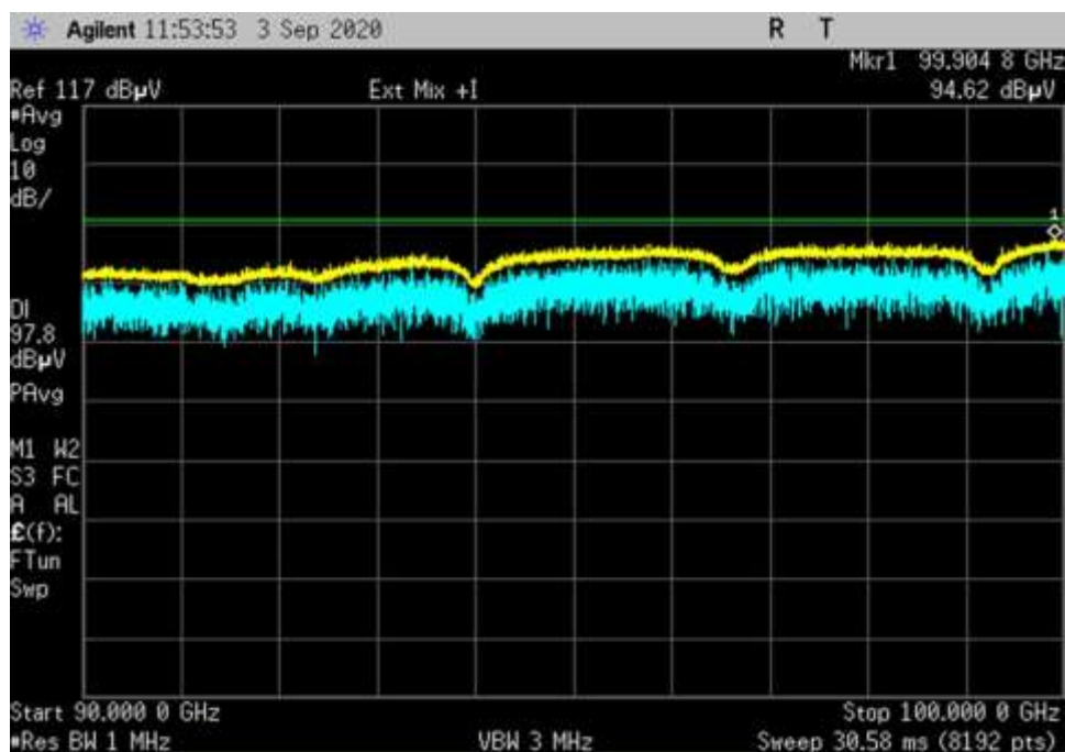
DL-Vout-64QAM-100MHz_90000-100000MHz_MC-V
