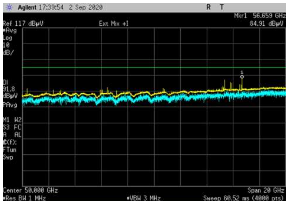
UL-Vout-Pi/2- BPSK-100MHz_ 40000- 60000MHz_MC-V
