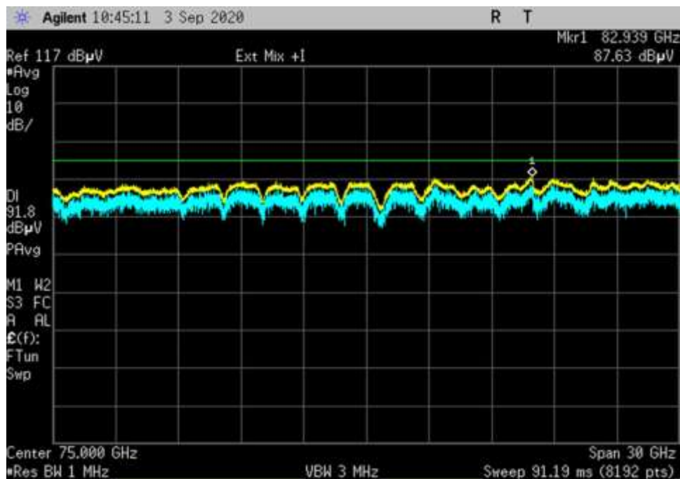
DL-Hout-QPSK-400MHz_ 60000- 90000MHz_MC-H
