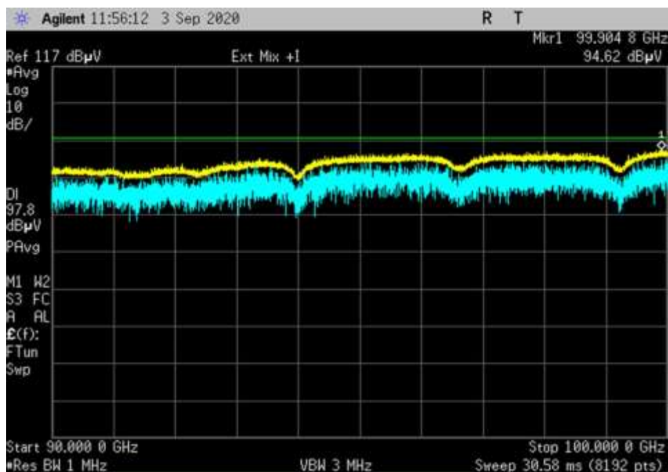
DL-Vout-256QAM-400MHz_ 90000- 100000MHz_MC-V
