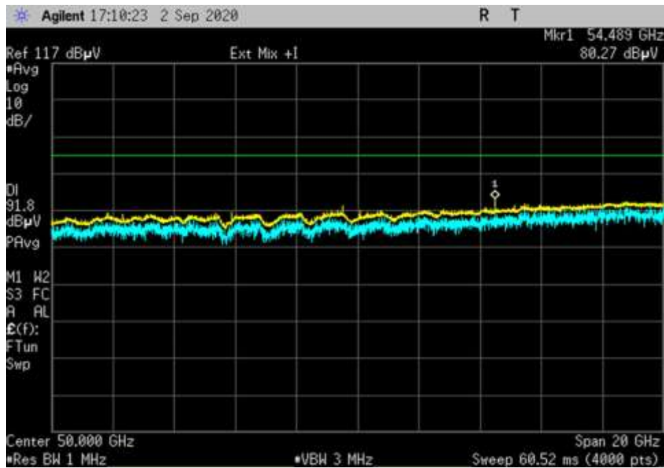
DL-Hout-QPSK-400MHz_ 40000- 60000MHz_MC-H
