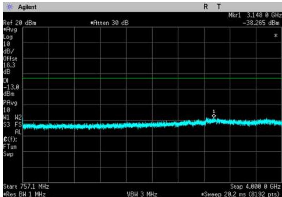
DL_746-757_757.1- 4000MHz_SN4
