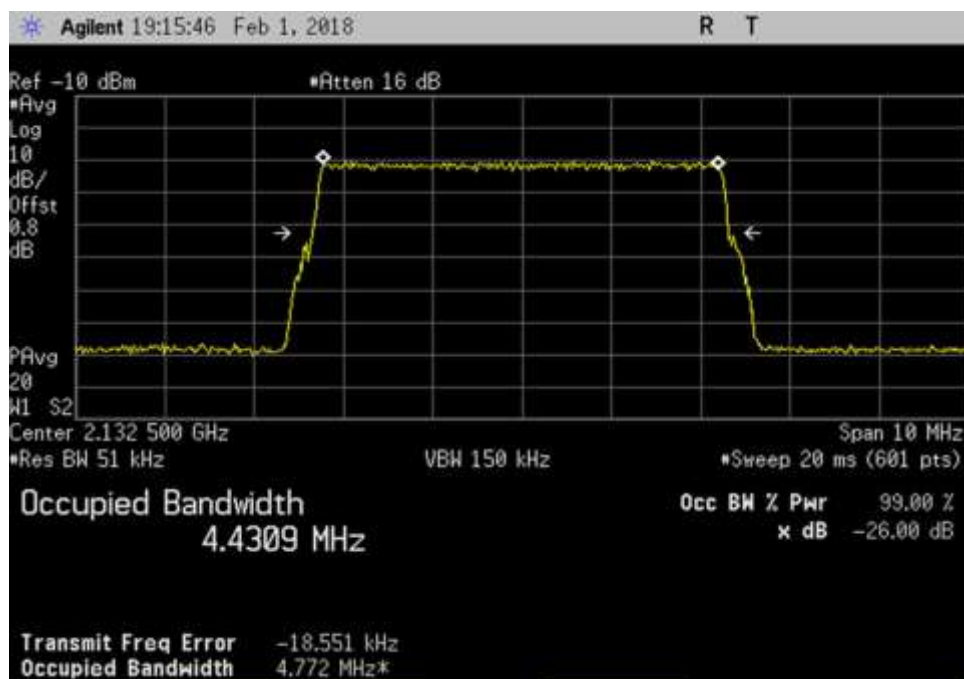
DL_2110-2155_LTE_ 2132.5MHz
