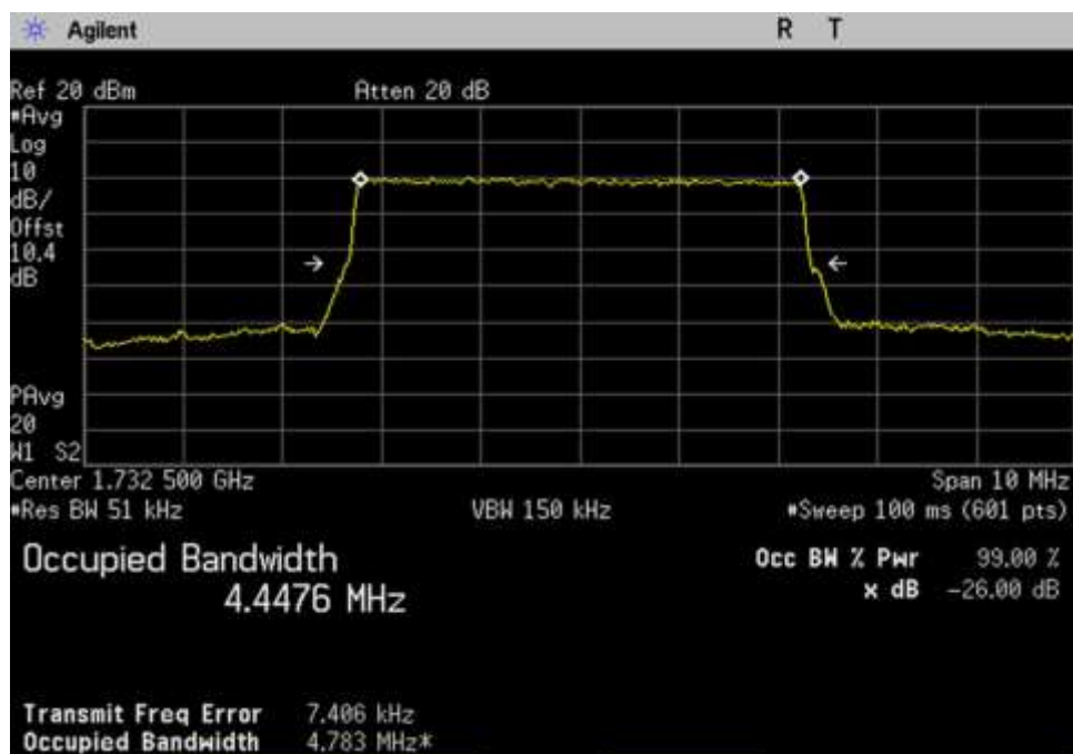
UL_1710-1755_LTE_1732.5MHz
