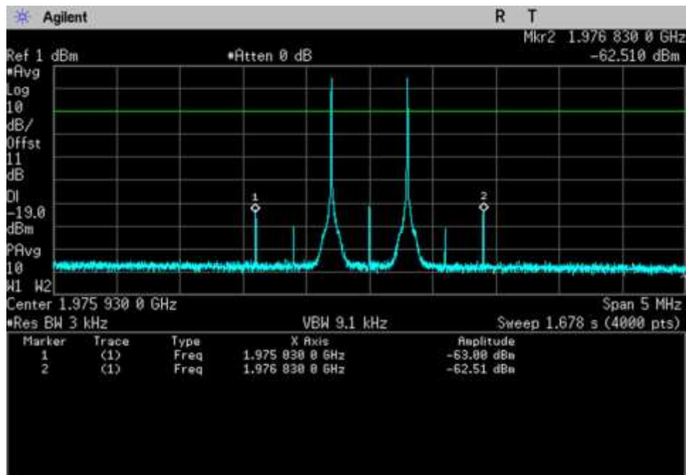
7.4_Intermod_DL_1930-1995MHz, 1975.93MHz
