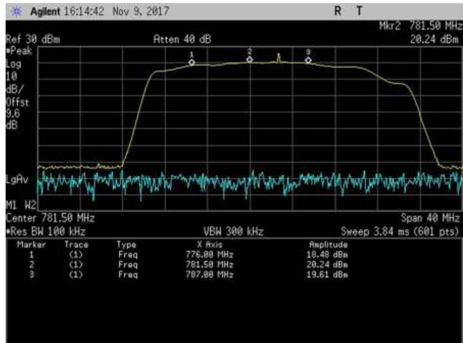
7.1_Band Verify_UL_776-787MHz_Zoom
