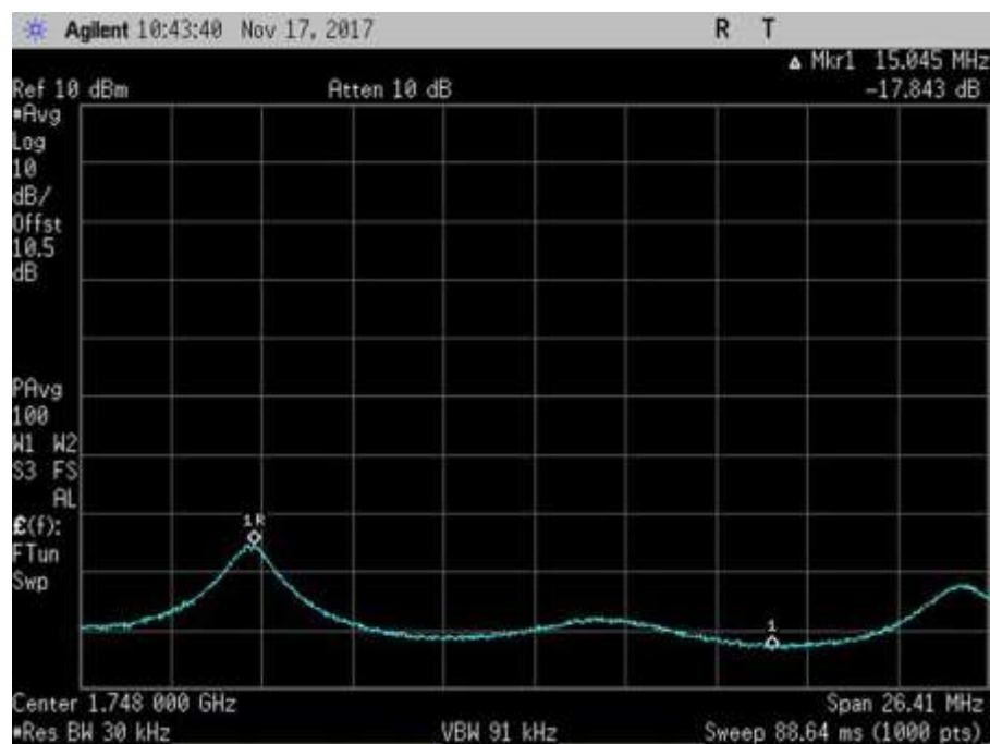
7.11.3_Osc_UL_1710-1755MHz+1_AWGNL
