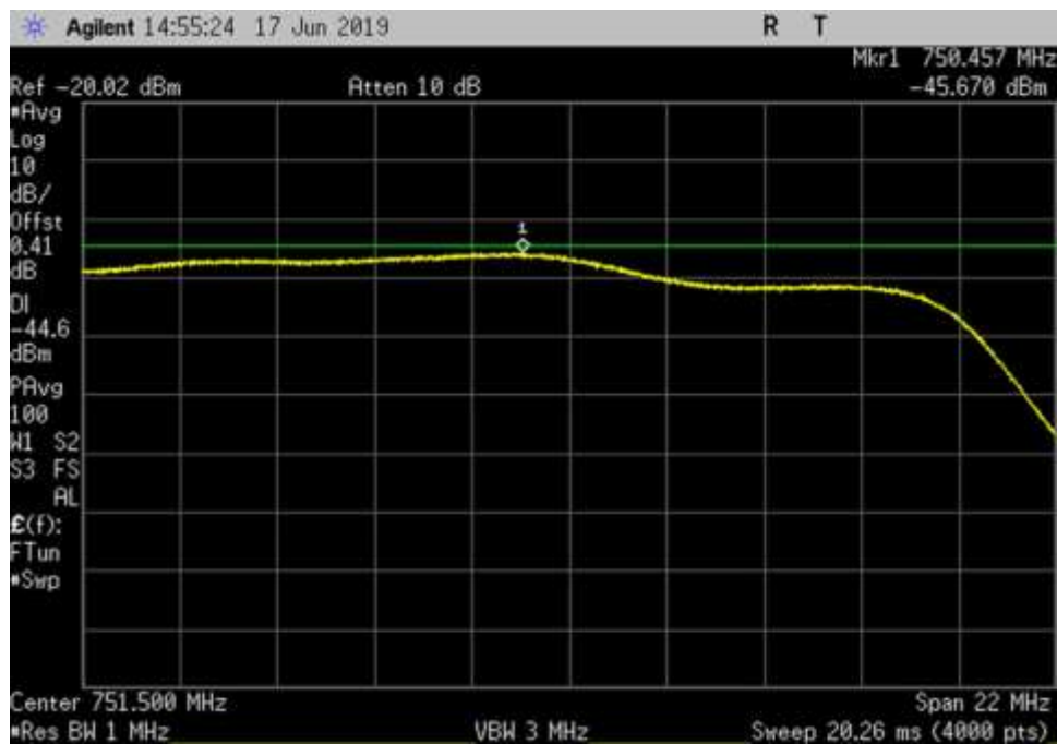
DL_746-757_ 751.5MHz
