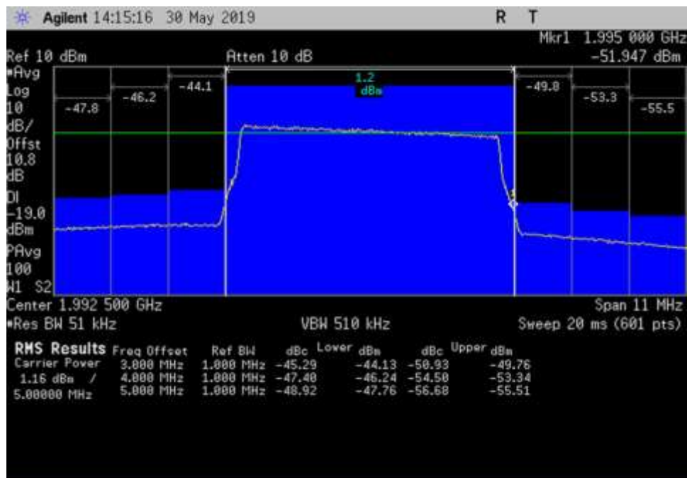
DL_1930-1995_LTE_ 1987- 1998MHz_100ft Cable
