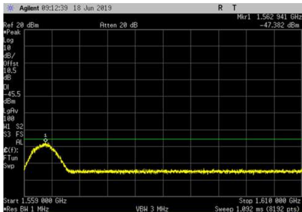
UL_776-787_ 1559- 1610MHz
