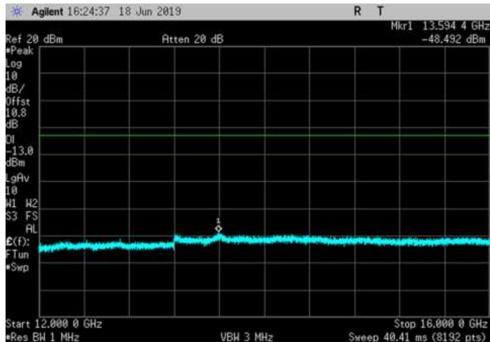
DL_1930-1995_ 12000- 16000MHz
