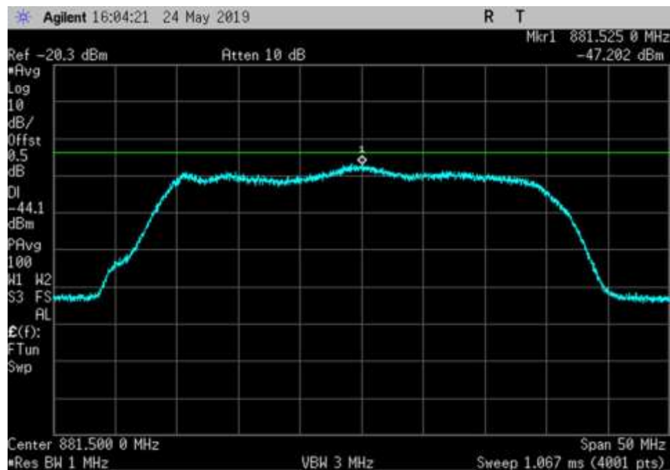
DL_869-894_881.5MHz_150ft Cable
