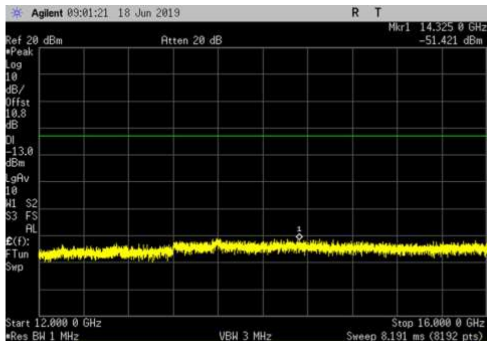
UL_1850-1915_ 12000- 16000MHz
