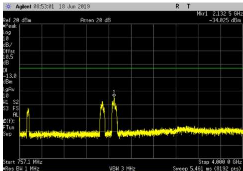
DL_746-757_757.1- 4000MHz
