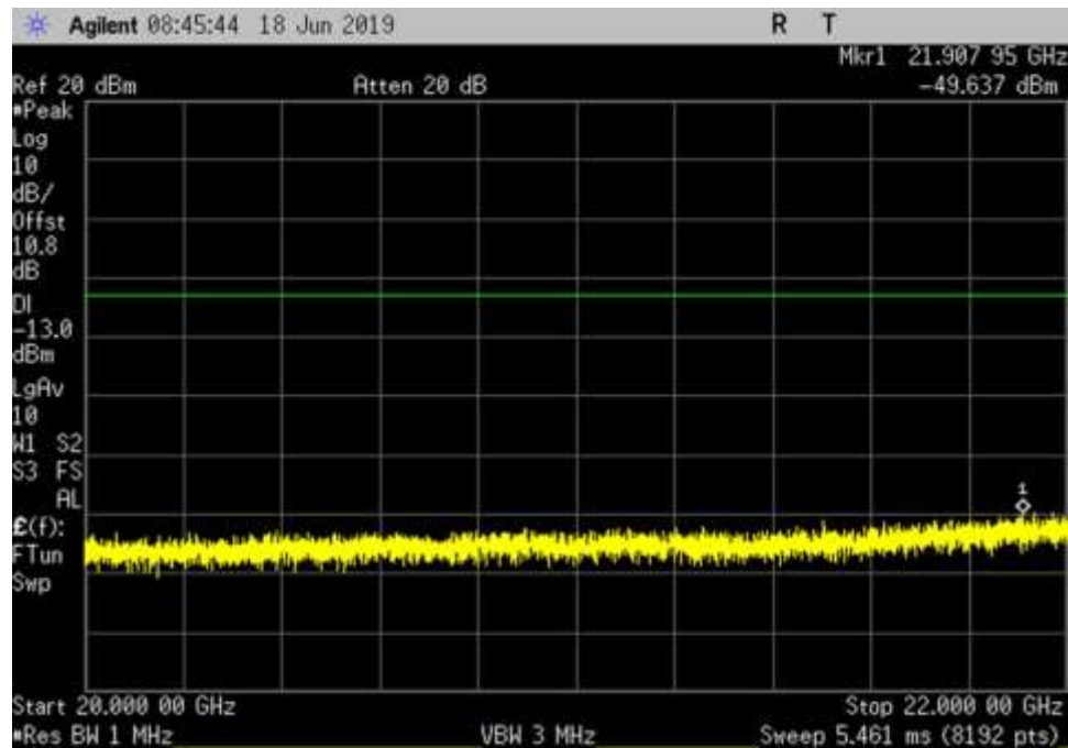
DL_2110-2155_ 20000- 22000MHz
