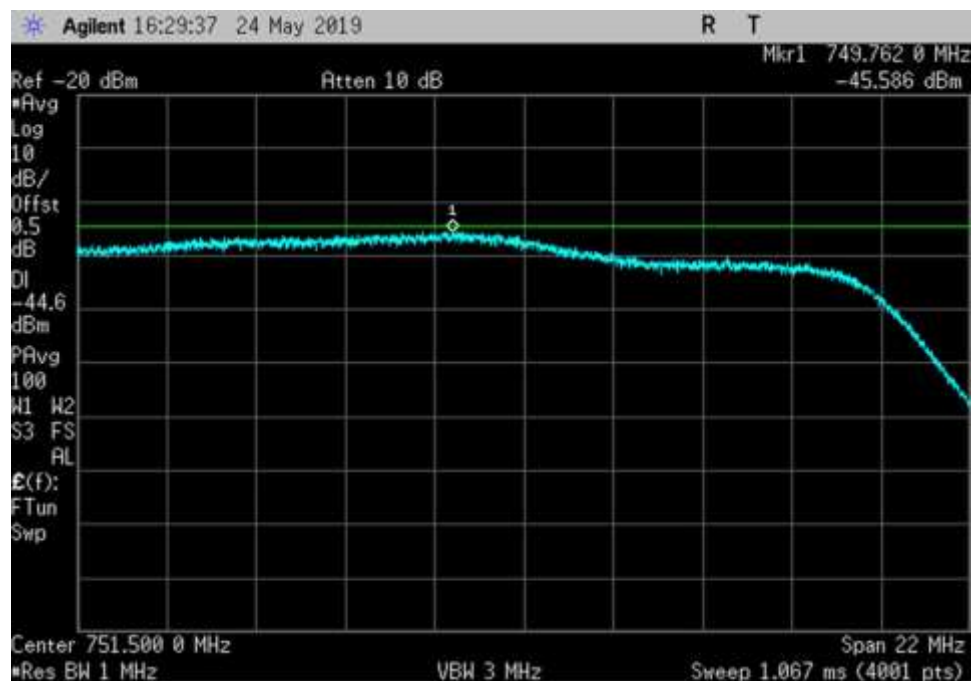
DL_746-757_ 751.5MHz_50ft Cable
