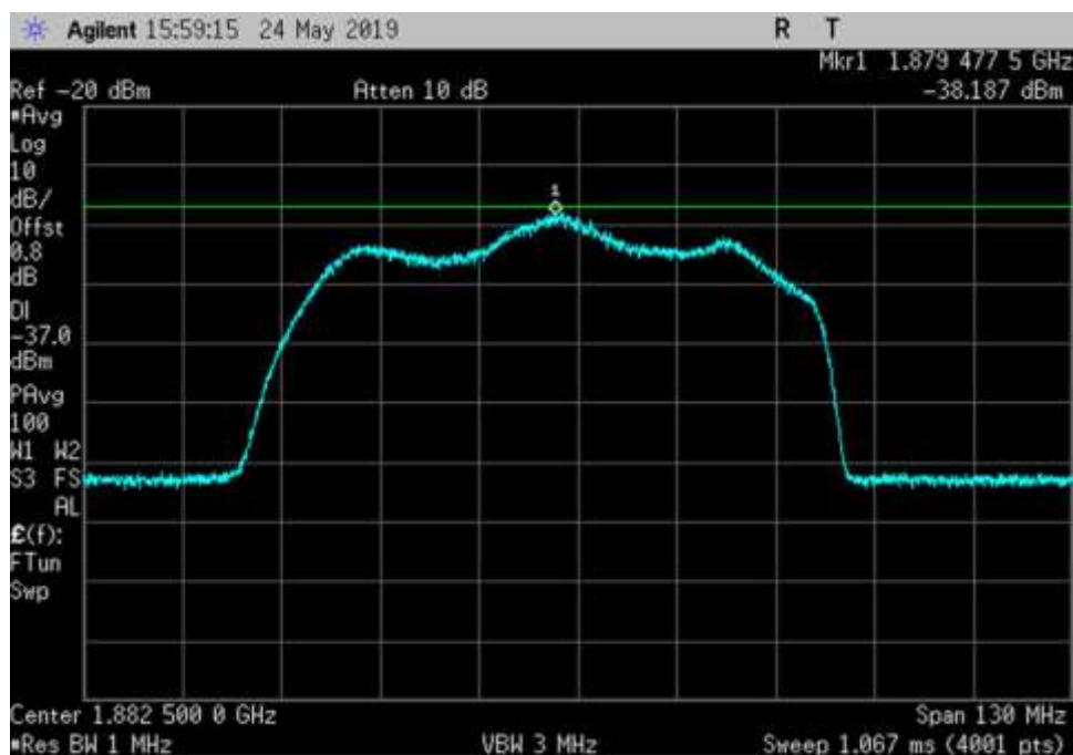
UL_1850-1915_1882.5MHz_150ft Cable
