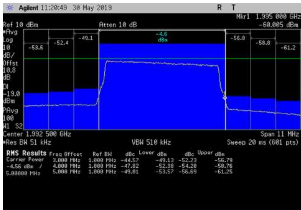
DL_1930-1995_LTE_ 1987- 1998MHz_150ft Cable
