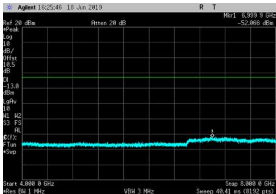
DL_869-894_4000-8000MHz
