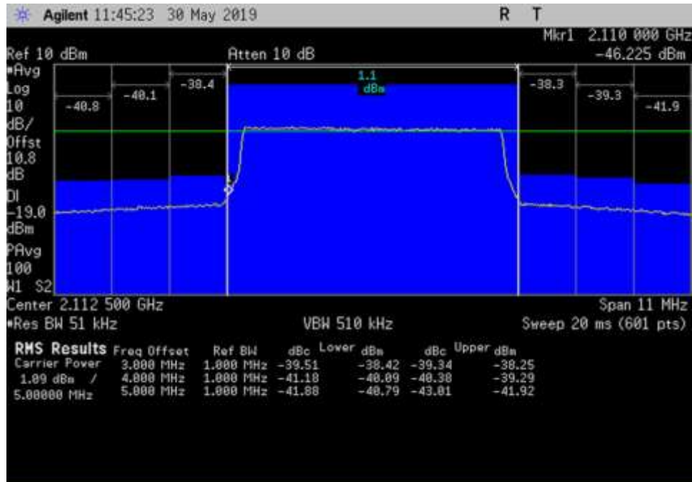
DL_2110-2155_LTE_2107- 2118MHz_100ft Cable
