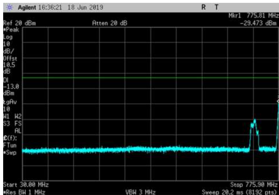
UL_776-787_ 30- 775.9MHz
