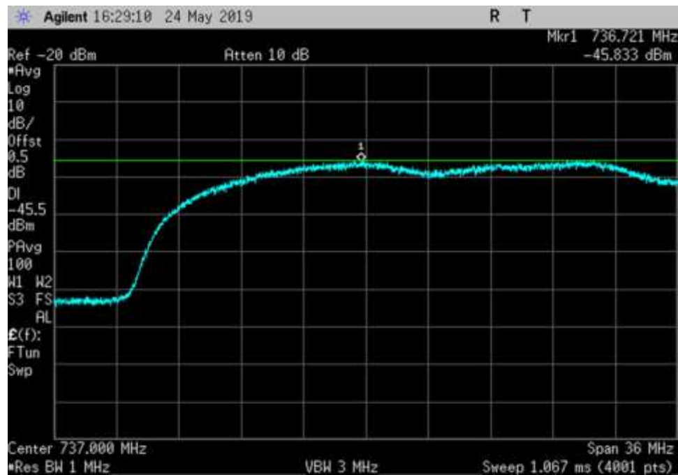
DL_728-746_ 737MHz_50ft Cable
