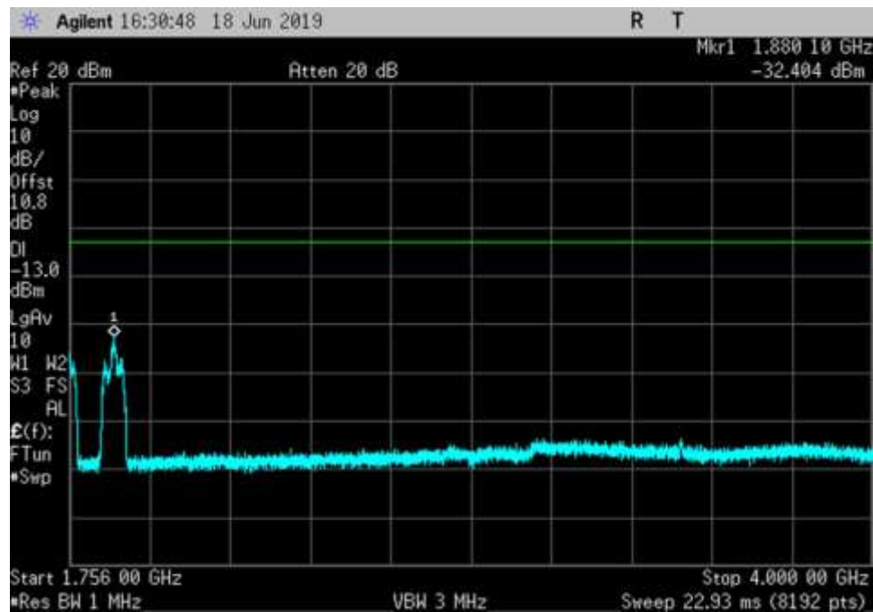
UL_1710-1755_ 1756- 4000MHz
