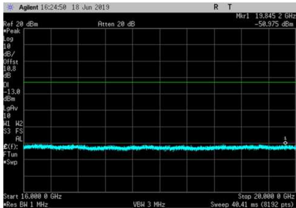
DL_1930-1995_ 16000- 20000MHz
