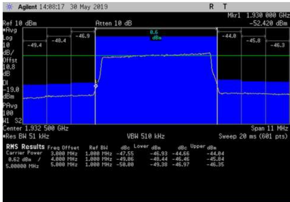
DL_1930-1995_LTE_ 1927- 1938MHz_100ft Cable
