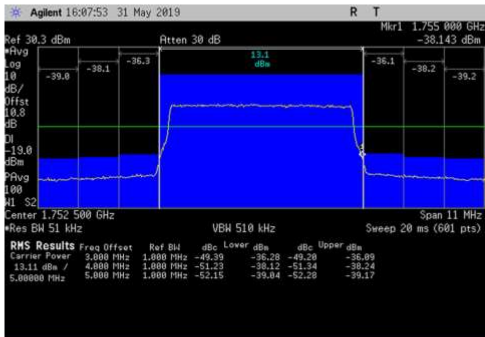
UL_1710-1755_LTE_1747- 1758MHz_100ft Cable
