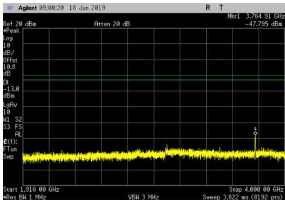
UL_1850-1915_1916- 4000MHz
