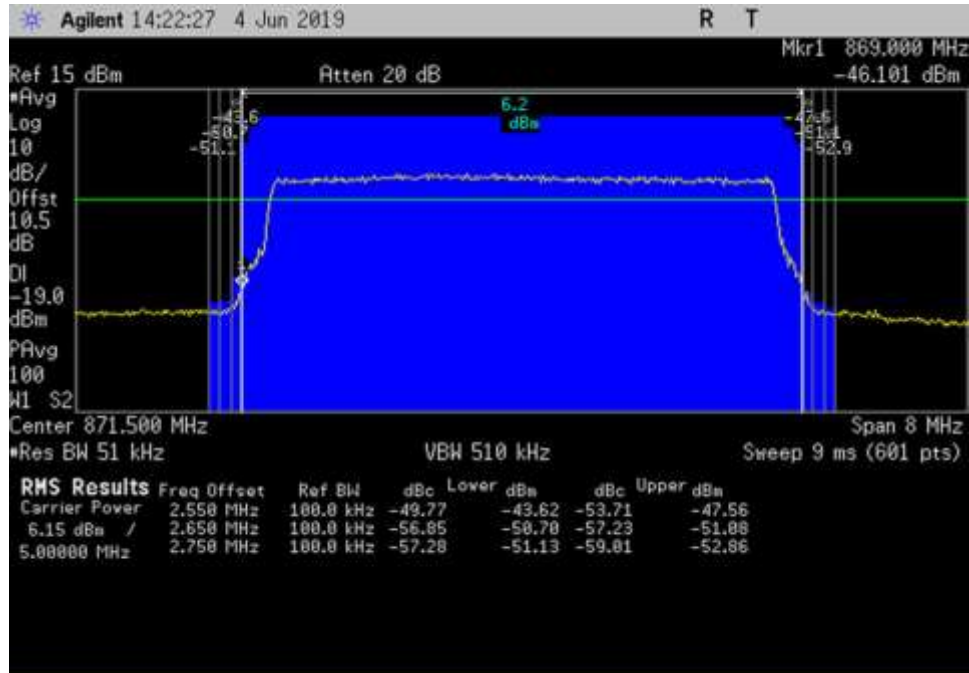
DL_869-894_LTE_ 867.5- 875.5MHz_50ft Cable
