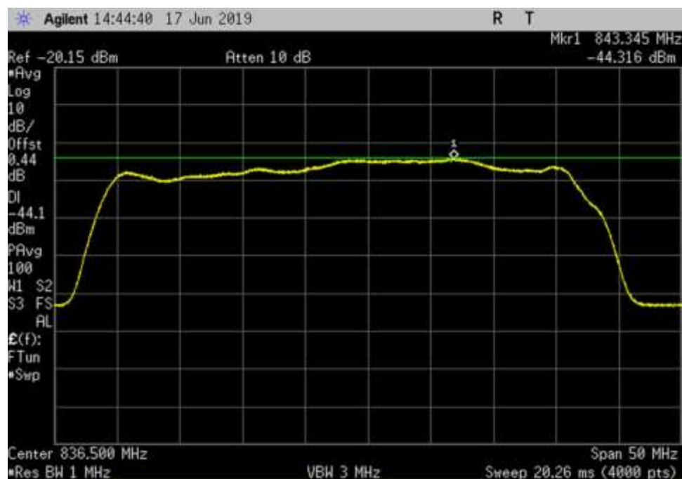
UL_824-849_ 836.5MHz
