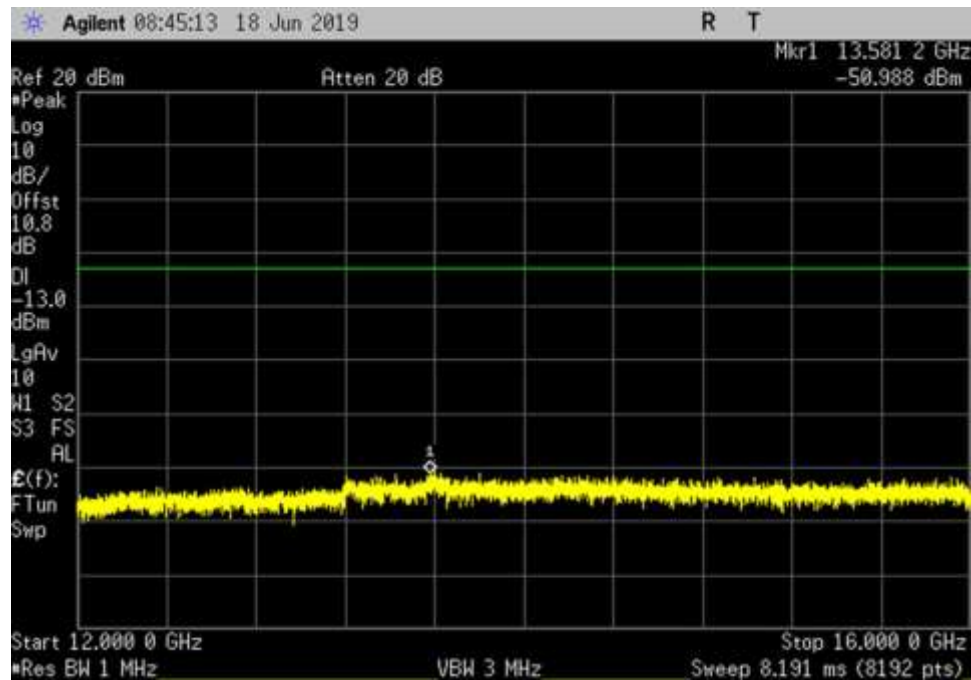
DL_2110-2155_ 12000- 16000MHz
