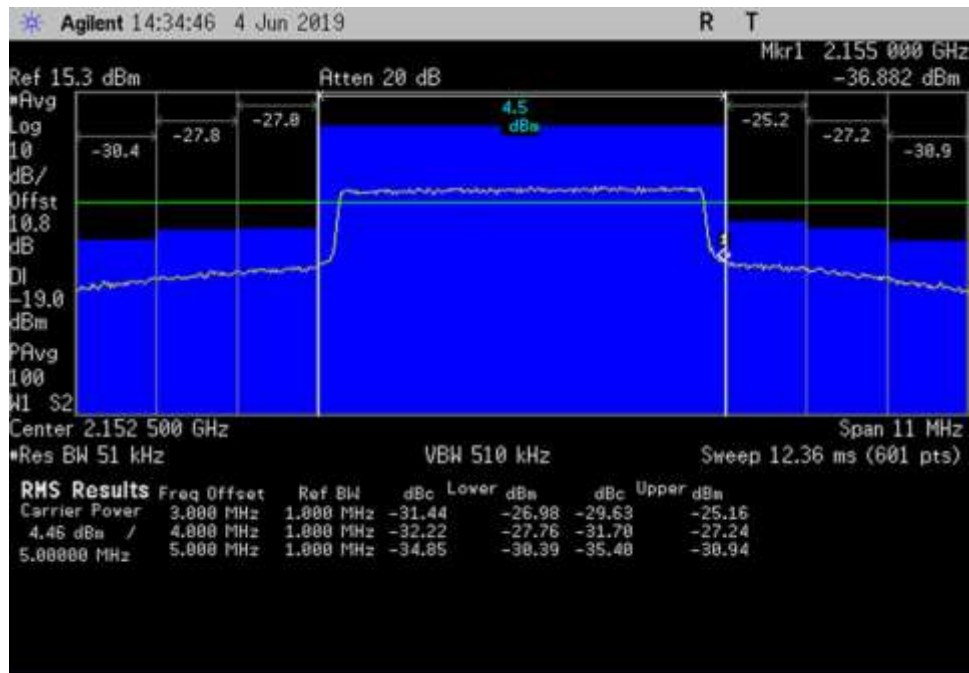
DL_2110-2155_LTE_2147-2158MHz_50ft Cable
