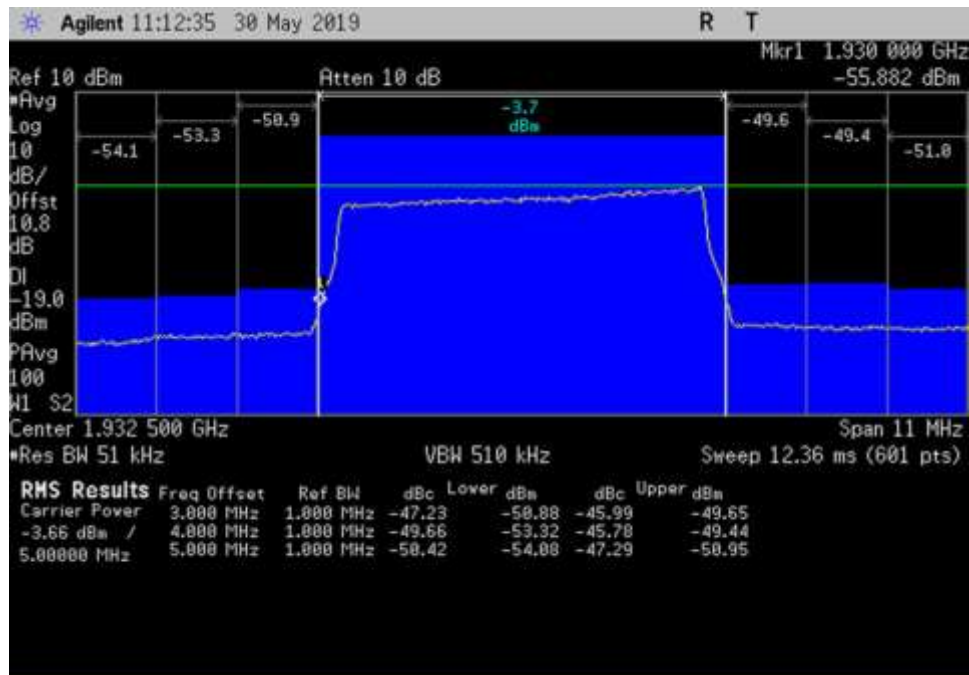
DL_1930-1995_LTE_ 1927- 1938MHz_150ft Cable
