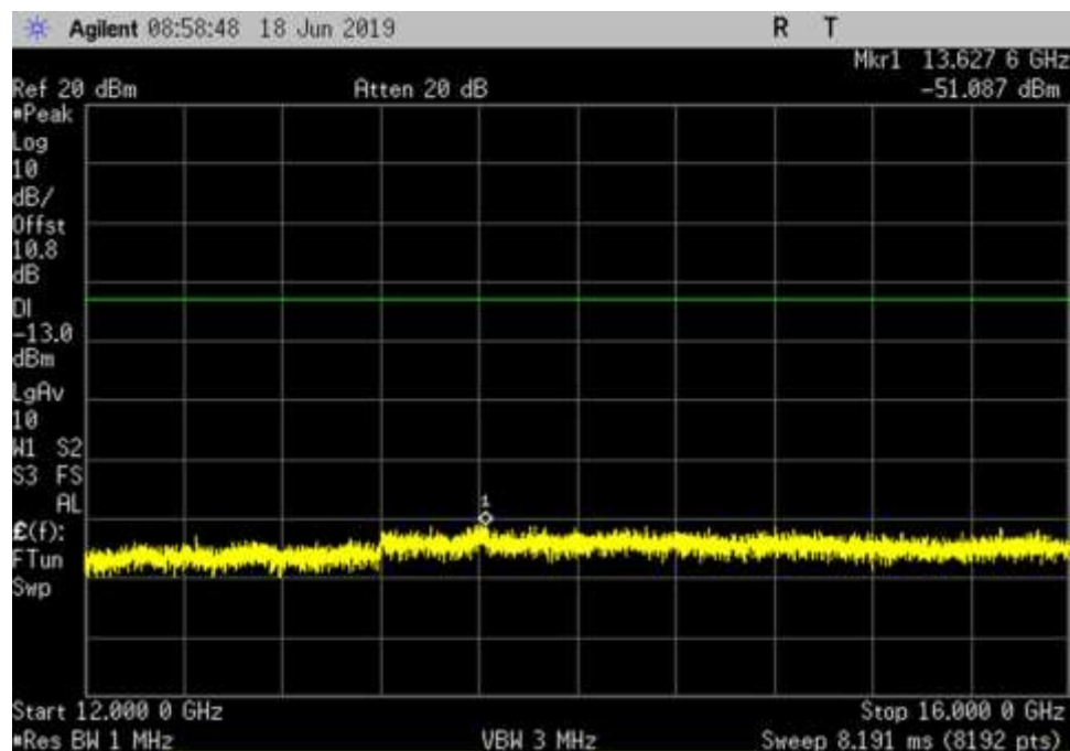
UL_1710-1755_12000- 16000MHz
