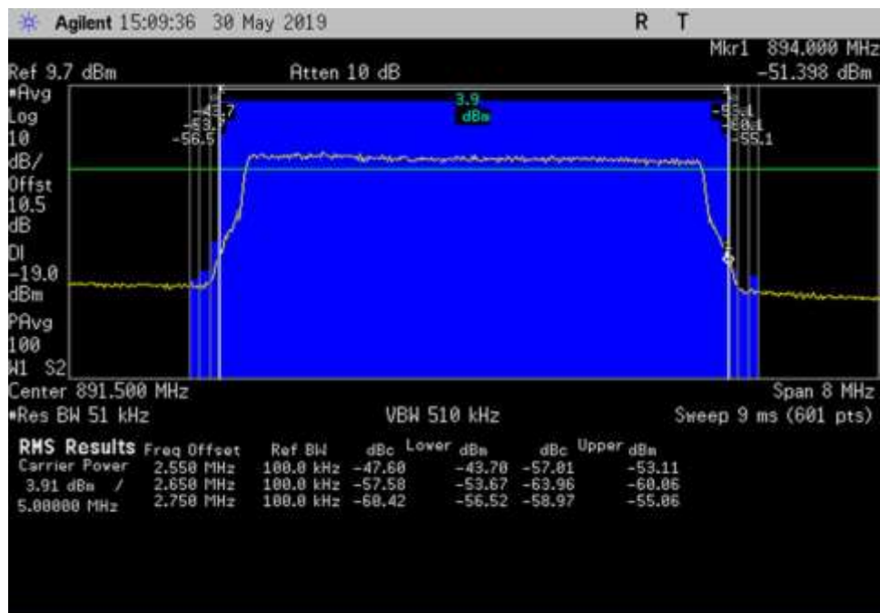
DL_869-894_LTE_887.5- 895.5MHz_100ft Cable
