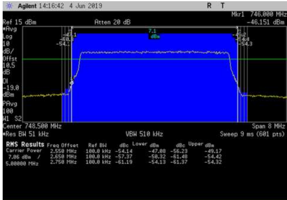
DL_746-757_LTE_ 744.5- 752.5MHz_50ft Cable
