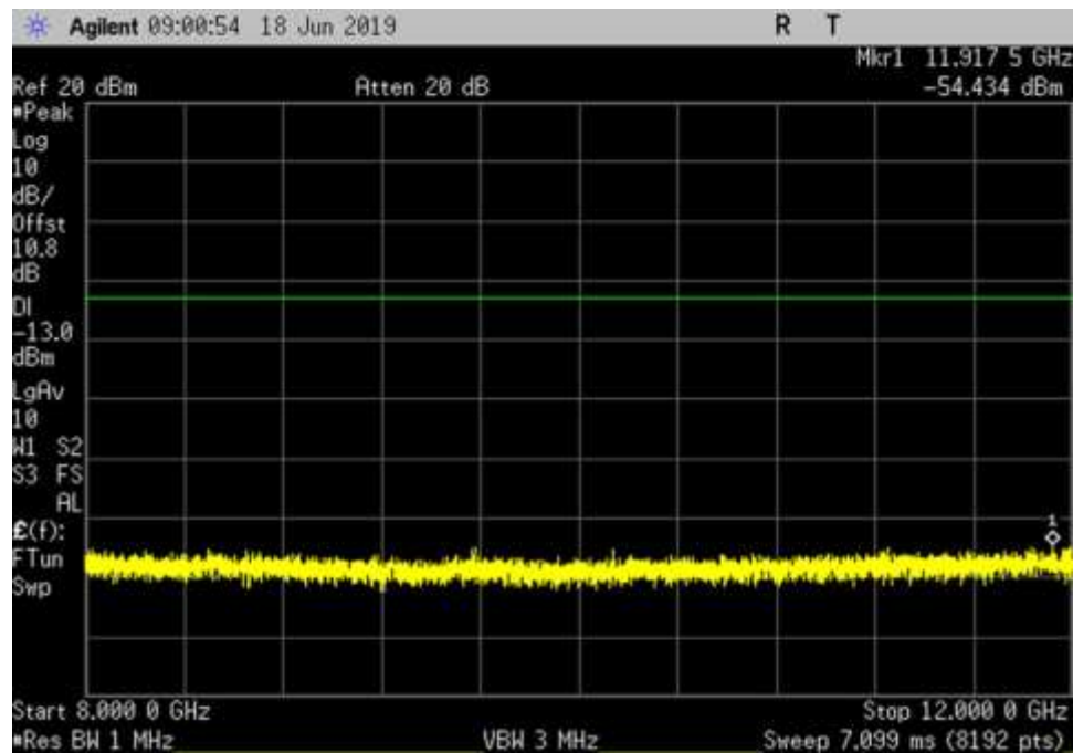
UL_1850-1915_ 8000- 12000MHz
