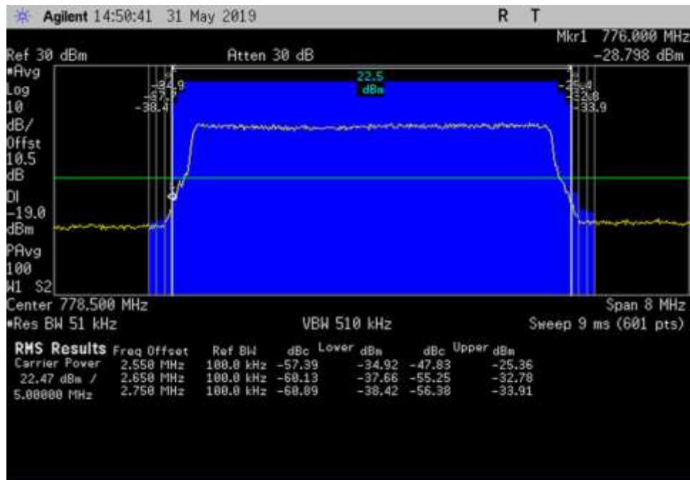
UL_776-787_LTE_ 774.5- 782.5MHz_100ft Cable
