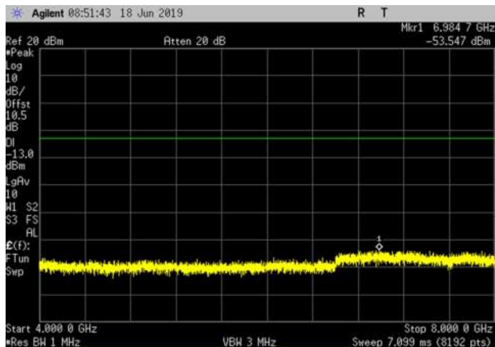
DL_728-746_4000- 8000MHz
