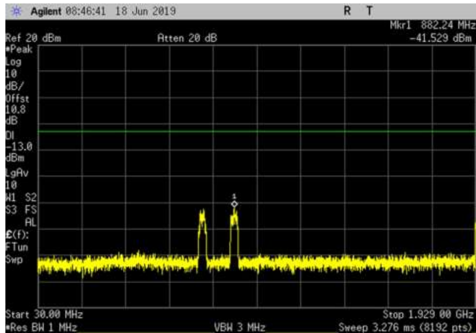
DL_1930-1995_ 30- 1929MHz
