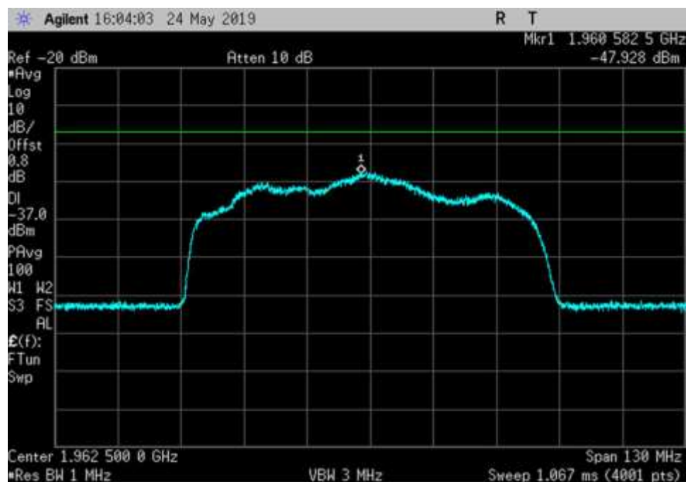
DL_1930-1995_1962.5MHz_150ft Cable
