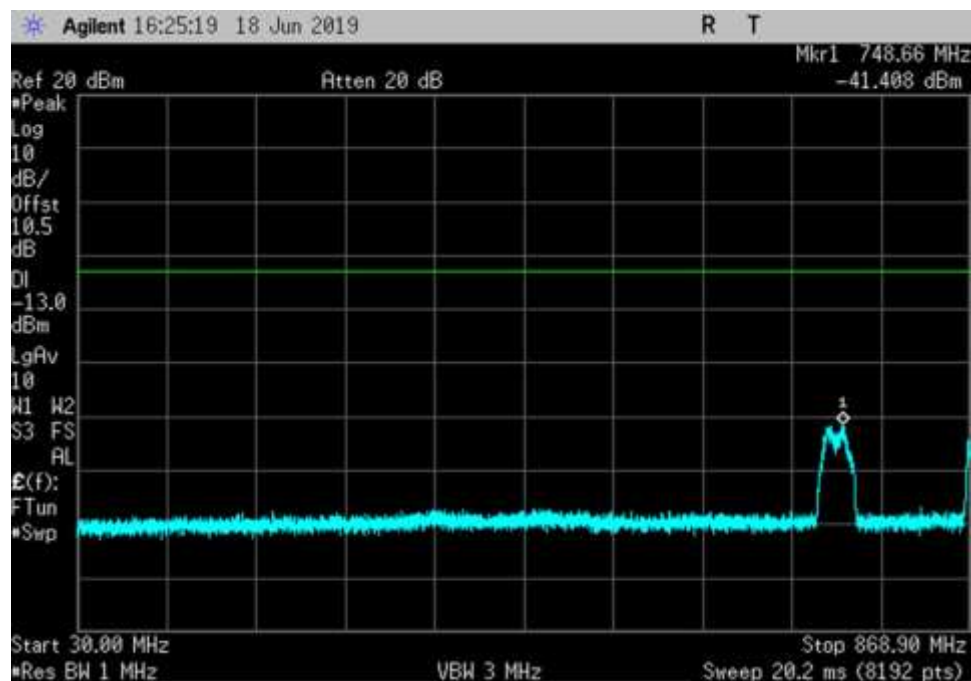
DL_869-894_ 30- 868.9MHz
