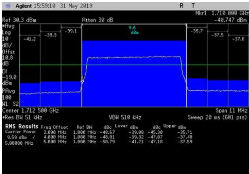
UL_1710-1755_LTE_1707- 1718MHz_100ft Cable
