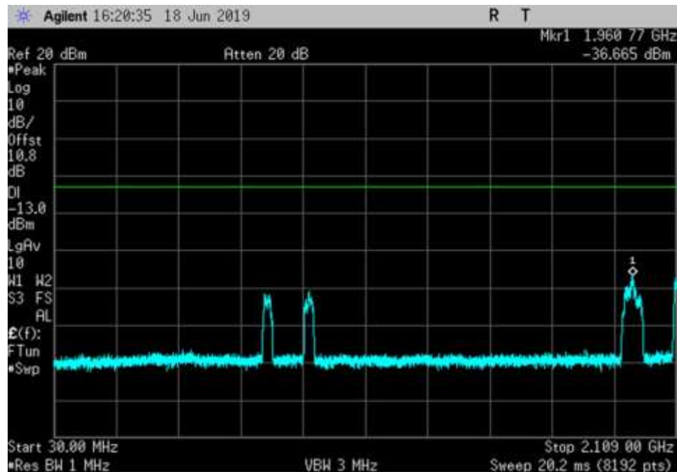
DL_2110-2155_ 30- 2109MHz
