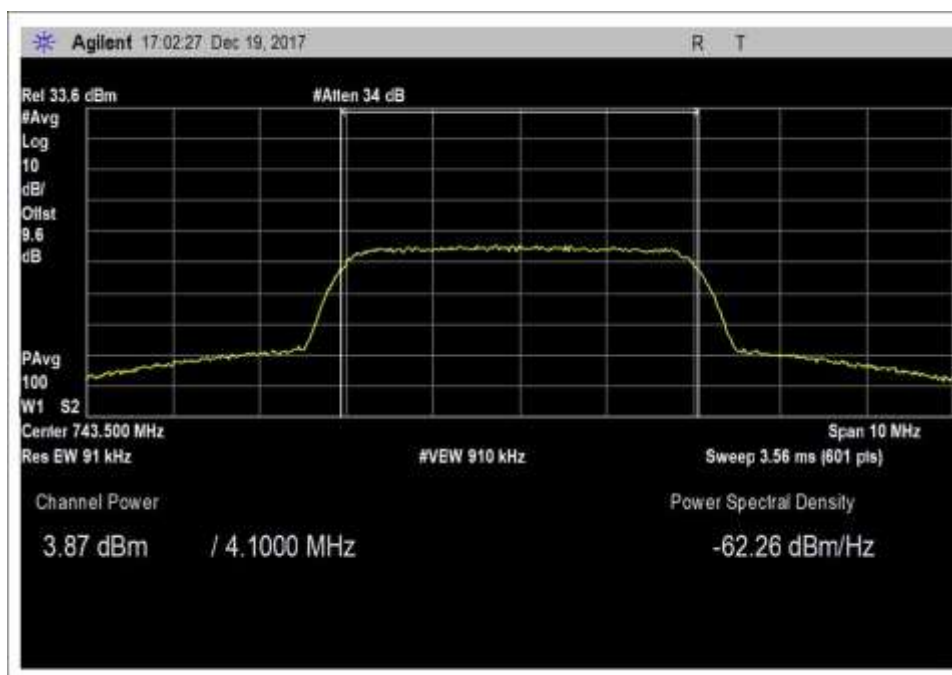
7.2 DL 728-746 AWGN_max
