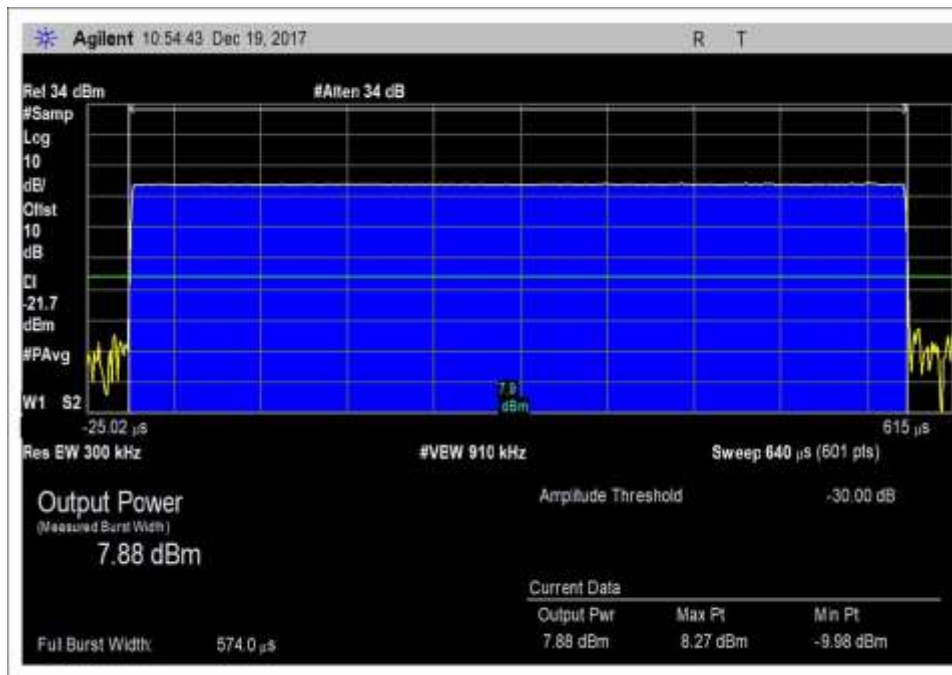
7.2 DL 1930-1995 pulse
