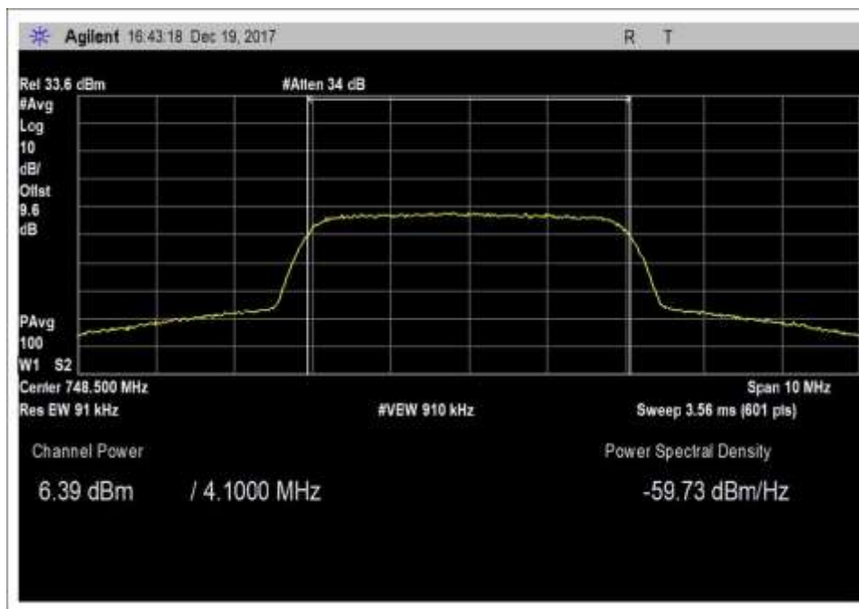
7.2 DL 746-757 AWGN
