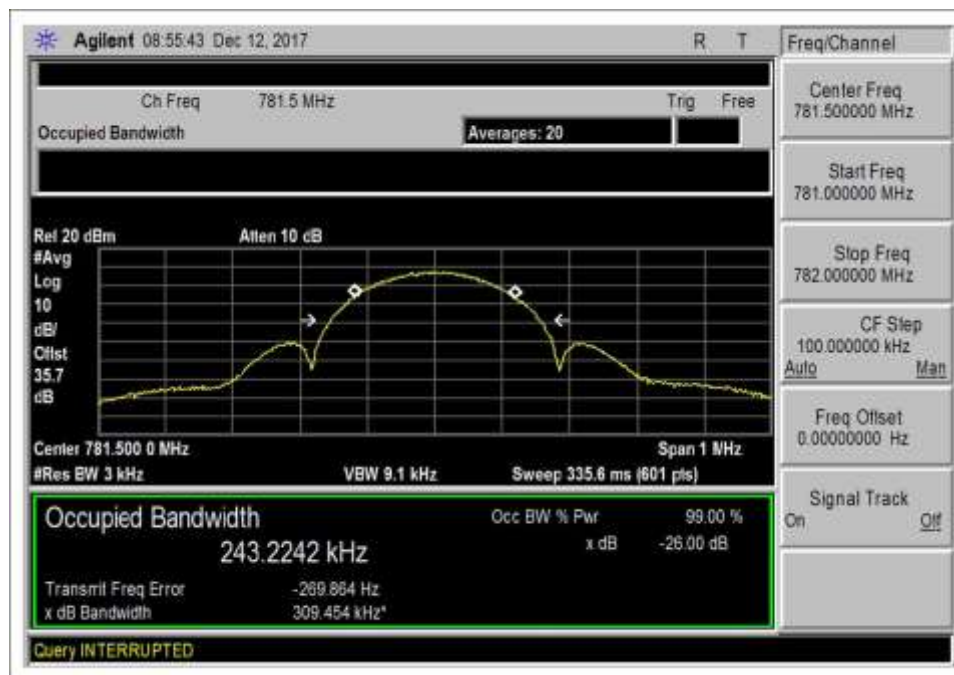
7.10 UL 776-787_EDGE_OUT
