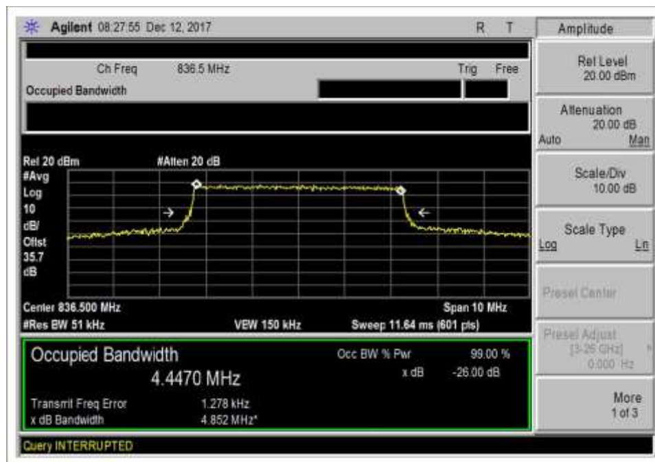
7.10 UL 824-849_LTE_OUT
