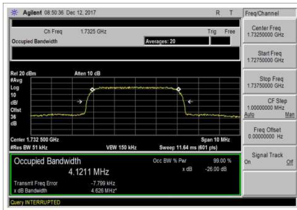
7.10 UL 1710-1755_WCDMA_OUT
