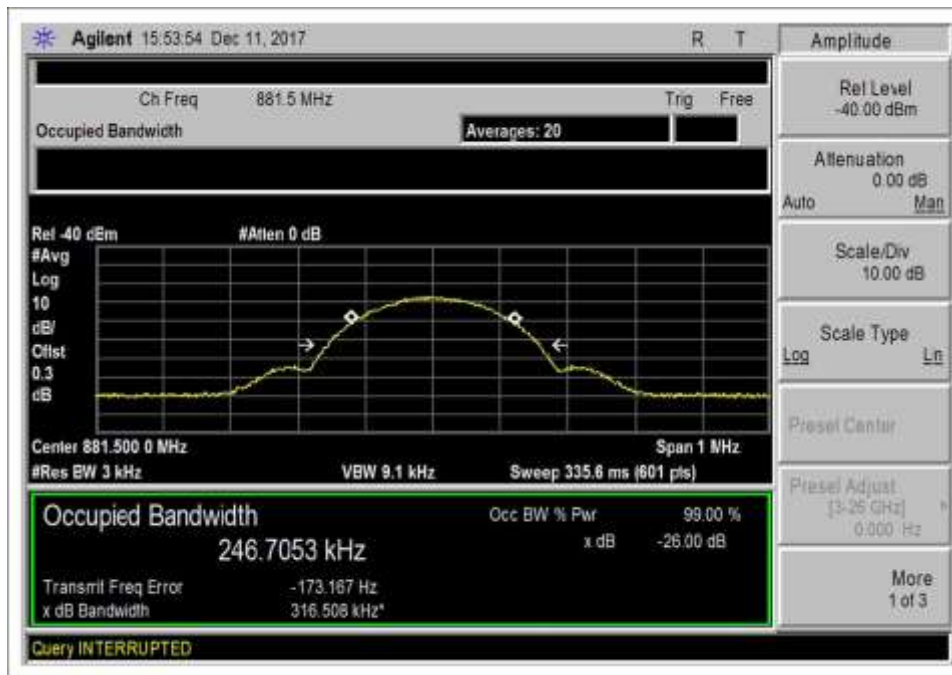
7.10 DL 869-894_GSM_IN
