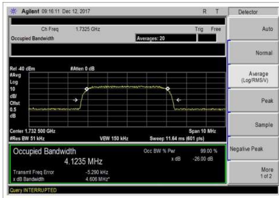
7.10 UL 1710-1755_WCDMA_IN
