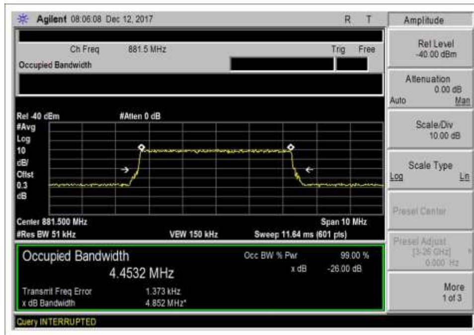
7.10 DL 869-894_LTE_IN
