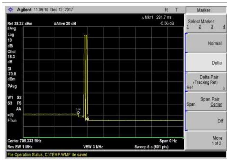
7.11.2 UL 698-716 time
