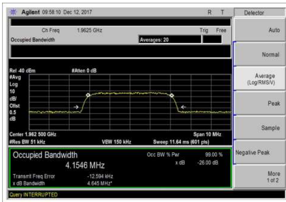
7.10 DL 1930-1995_WCDMA_IN
