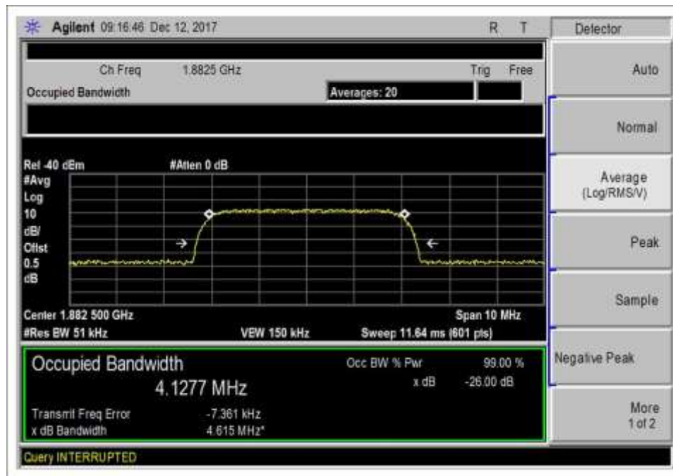
7.10 UL 1850-1915_WCDMA_IN
