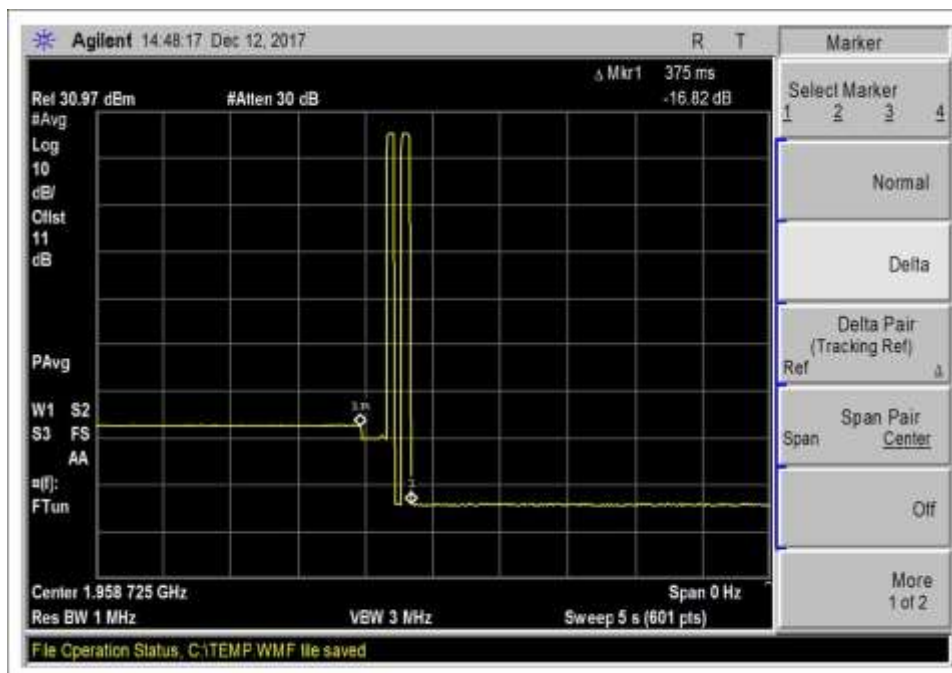
7.11.2 DL 1930-1995 time
