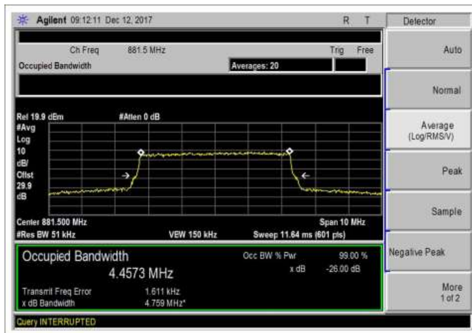
7.10 DL 869-894_LTE_OUT
