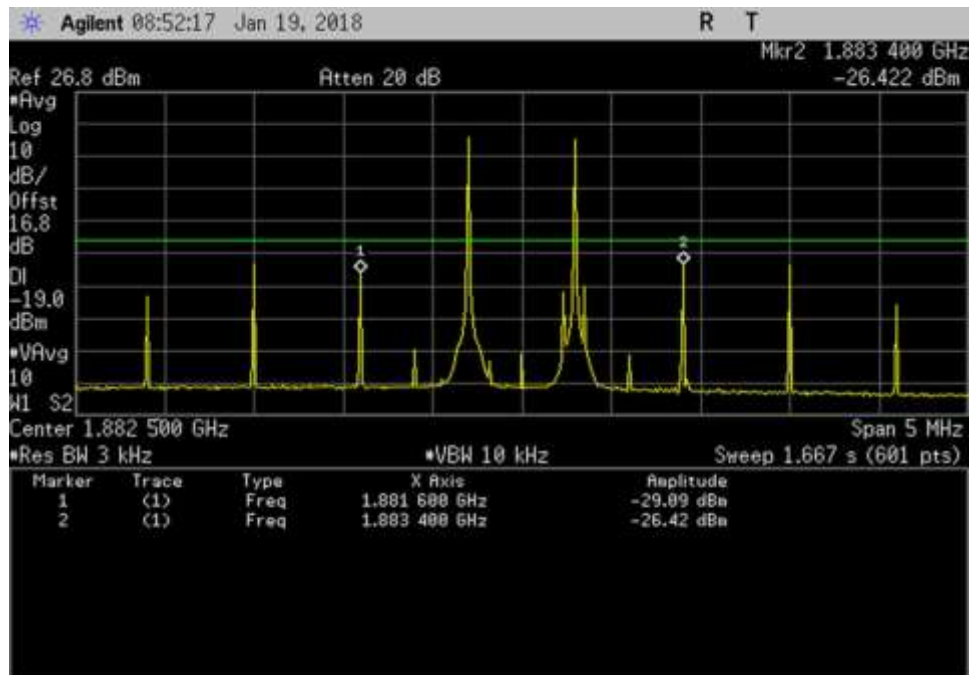
UL_ 1882.5MHz
