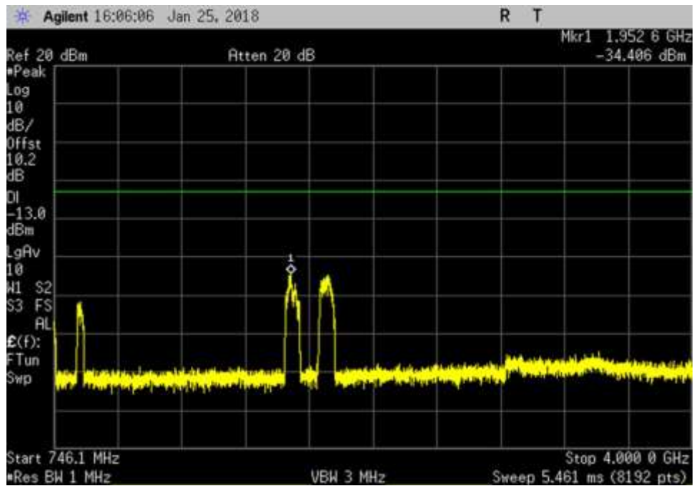
DL_ 746.1- 4000MHz_AWGN
