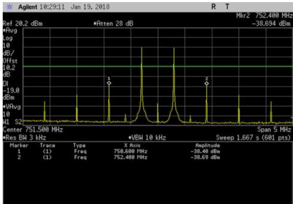
DL_ 751.5MHz
