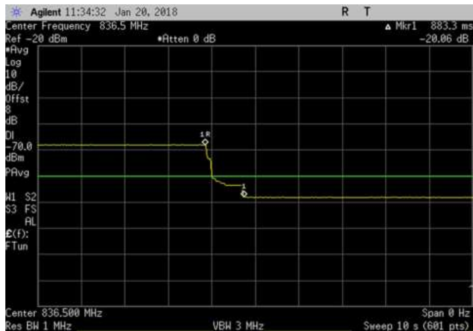
UL_836.5MHz_UL Time
