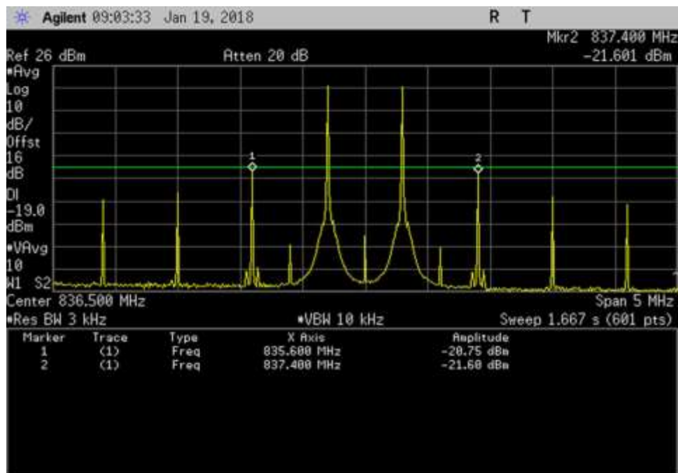
UL_ 836.5MHz
