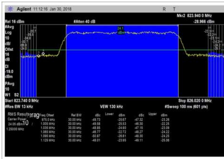
UL_824-849MHz_CDMA_rbw_30Khz_ACP_pre_agc_L_revB
