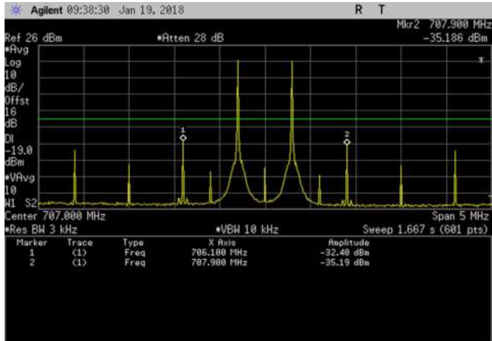
UL_707MHz
