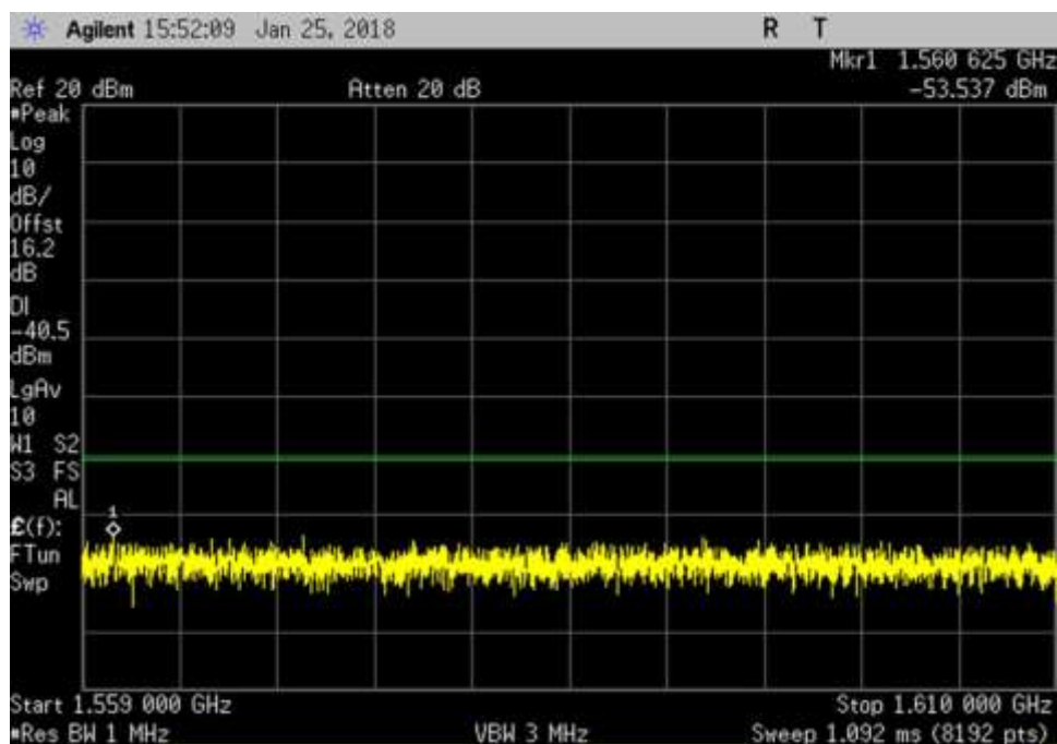
UL_ 1559- 1610MHz_AWGN
