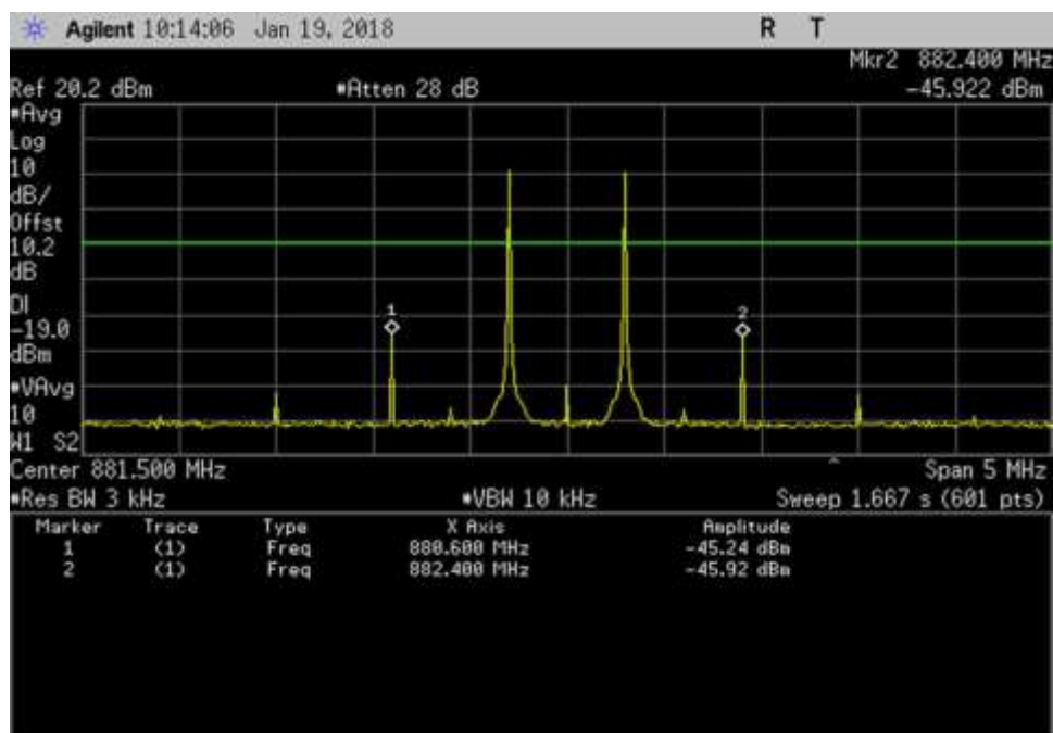
DL_ 881.5MHz
