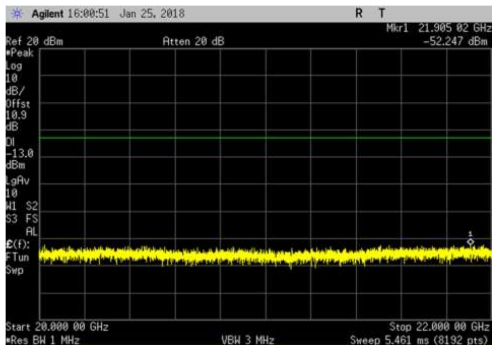
DL_ 20000- 22000MHz_AWGN
