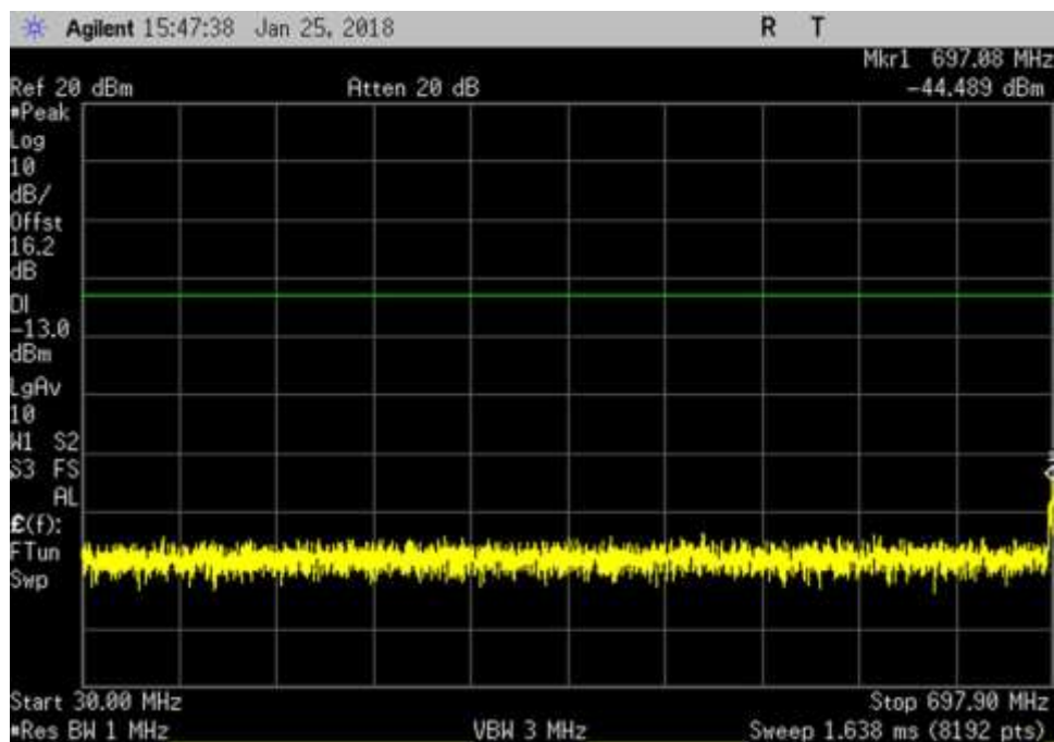
UL_30- 697.9MHz_AWGN
