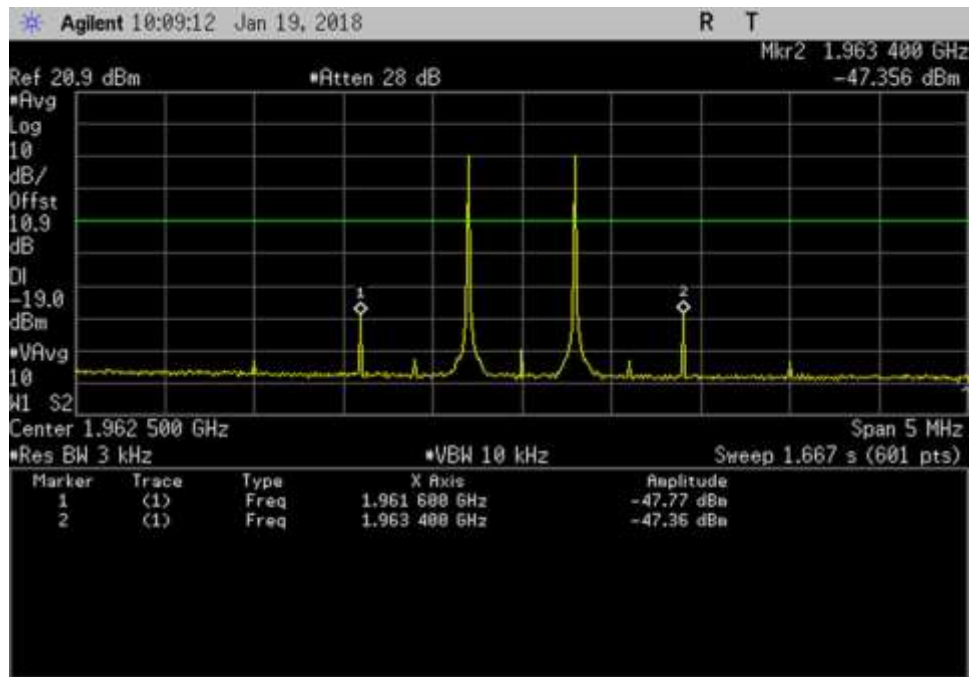
DL_1962.5MHz
