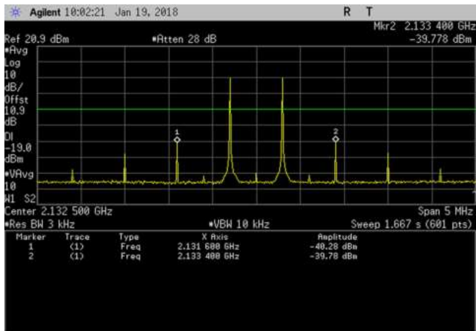
DL_2132.5MHz
