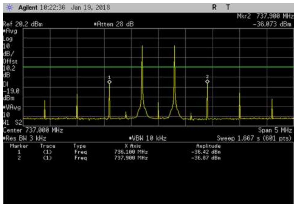
DL_ 737MHz
