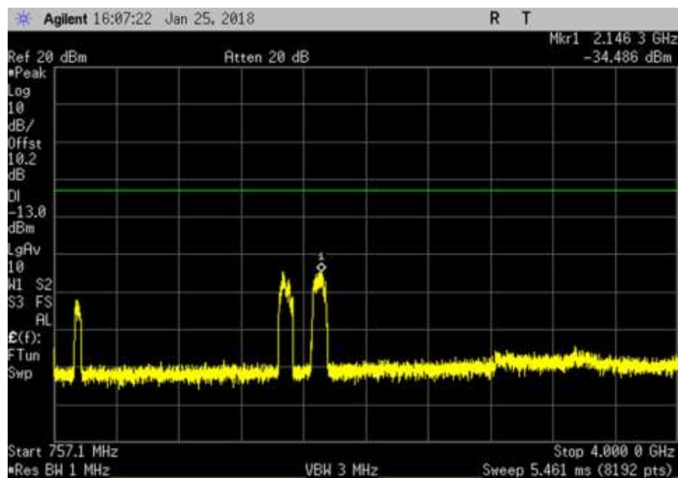
DL_ 757.1- 4000MHz_AWGN
