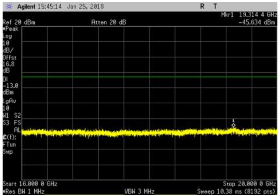
UL_ 16000- 20000MHz_AWGN
