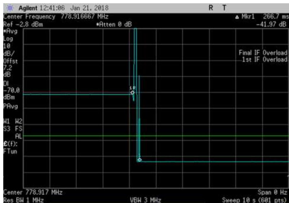
UL_ 778.916667MHz_time
