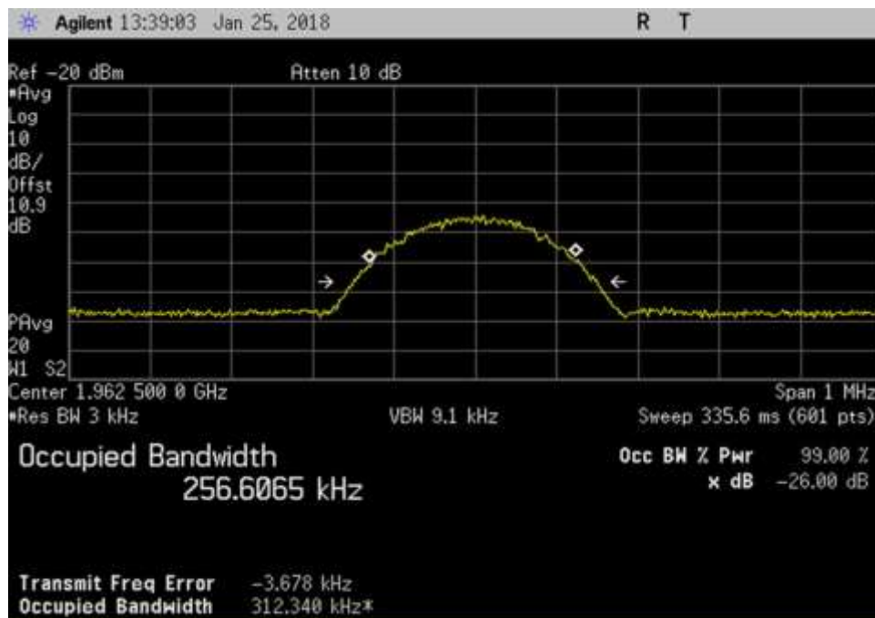
DL_1962.5MHz_EDGE
