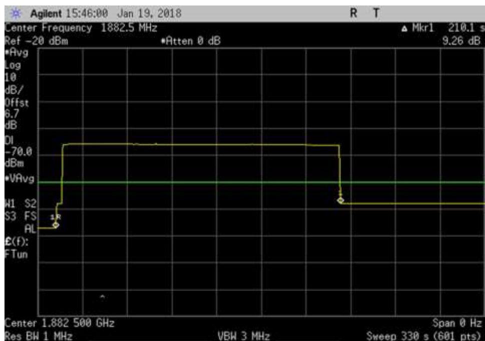
UL_1882.5MHz
