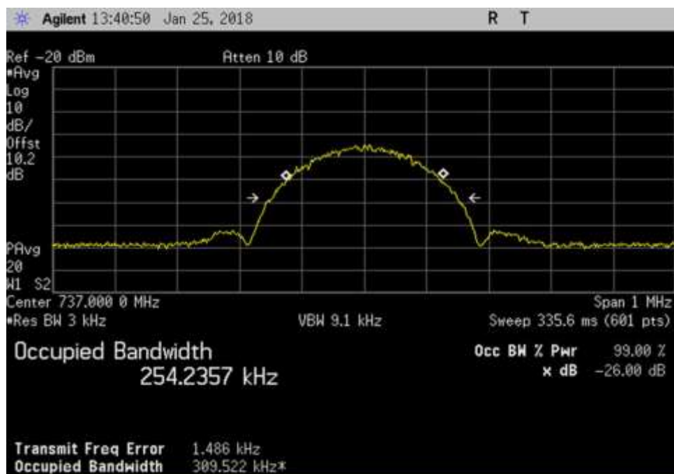
DL_737MHz_EDGE
