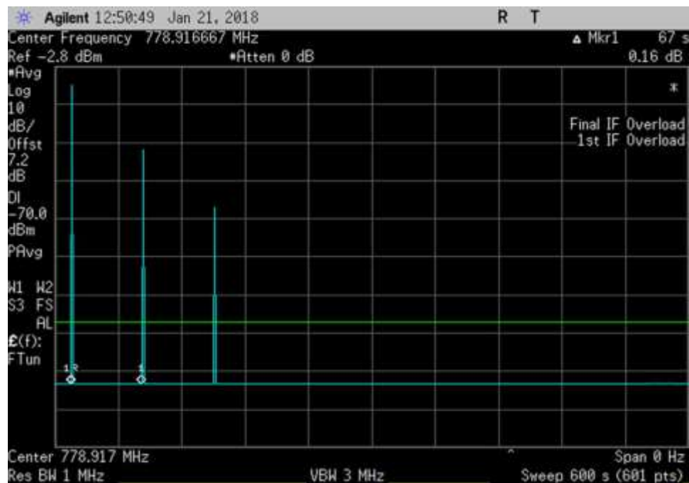
UL_ 778.916667MHz_600sec
