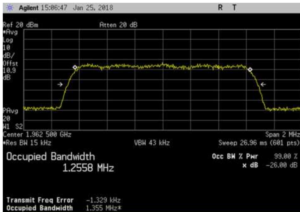
DL_1962.5MHz_CDMA
