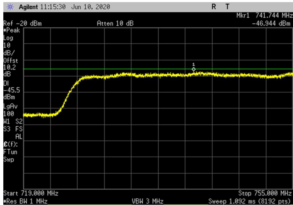
DL_728-746_737MHz_Max
