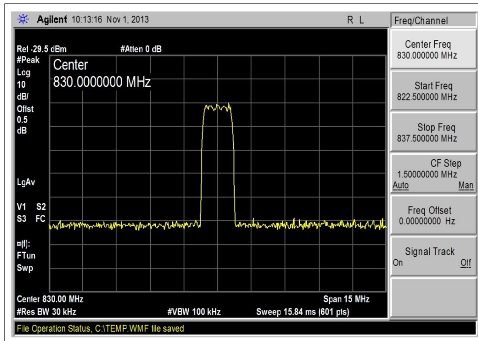
824-894MHz, UL_CDMA_Input
