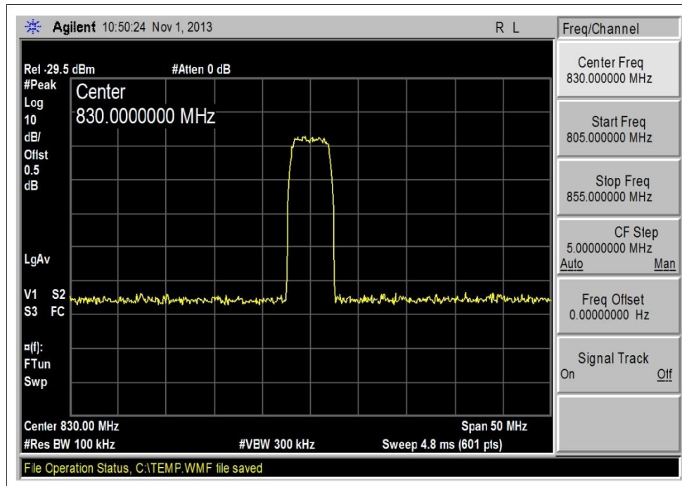
824-894MHz, UL_WCDMA_Input
