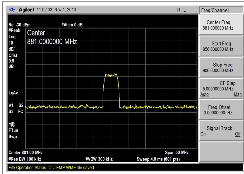
869-894MHz, DL_WCDMA_Input
