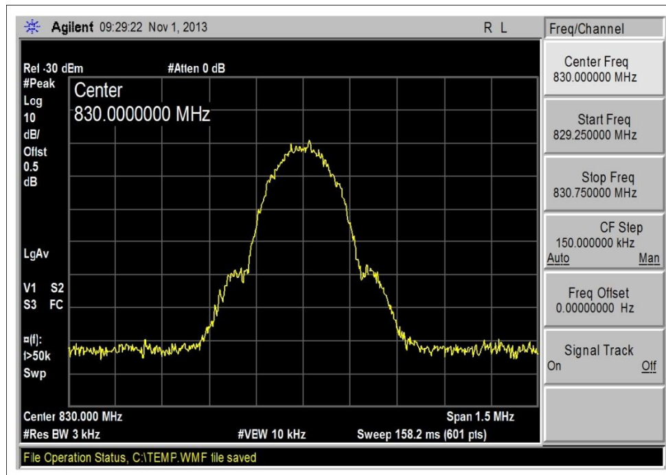
824-849MHz, UL_GSM_Input
