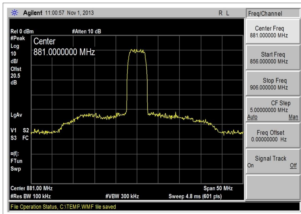
869-894MHz, DL_WCDMA_Output
