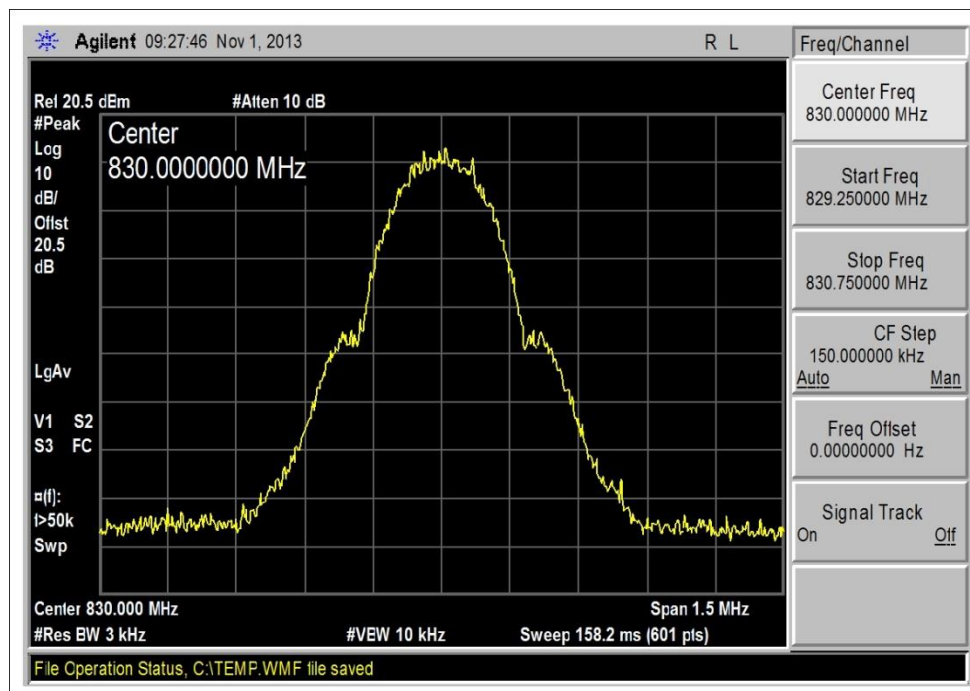
824-849MHz, UL_GSM_Output
