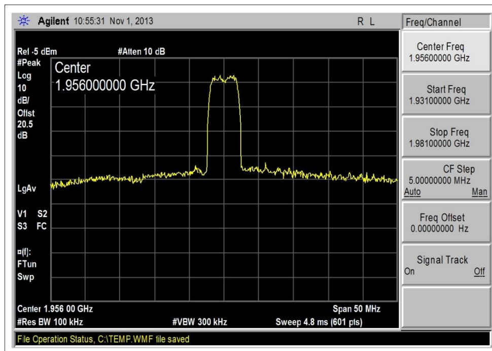
1930-1990MHz DL_WCDMA_Output
