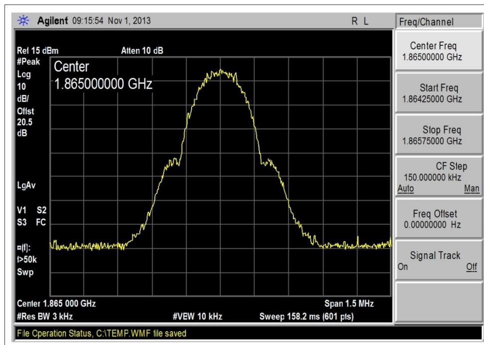
1850-1910MHz UL_GSM_Output
