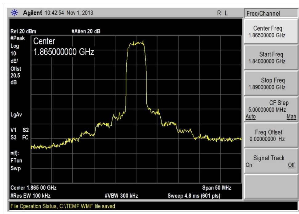
1850-1910MHz UL_WCDMA_Output
