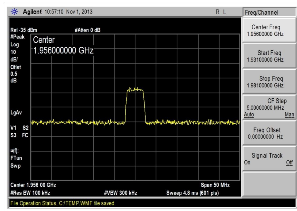
1930-1990MHz DL_WCDMA_Input
