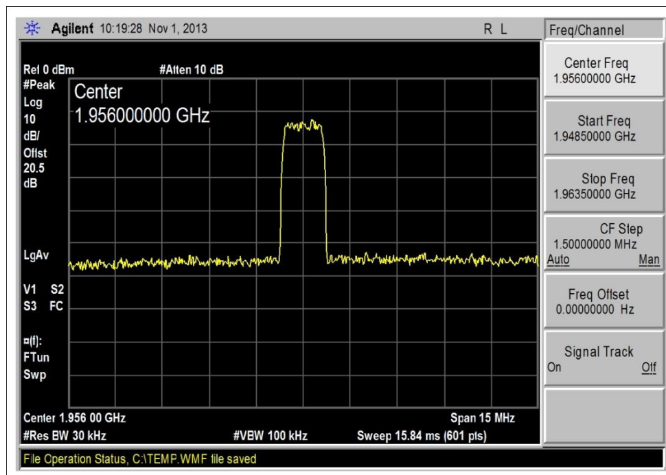
1930-1990MHz DL_CDMA_Output
