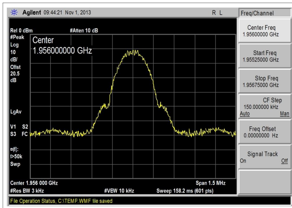
1930-1990MHz DL_GSM_Output
