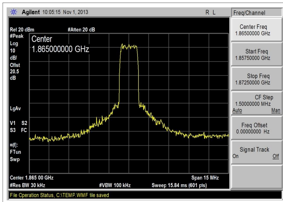
1850-1910MHz UL_CDMA_Output
