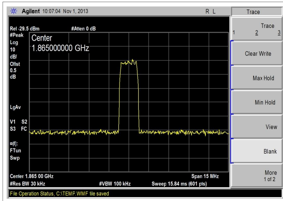
1850-1910MHz UL_CDMA_Input
