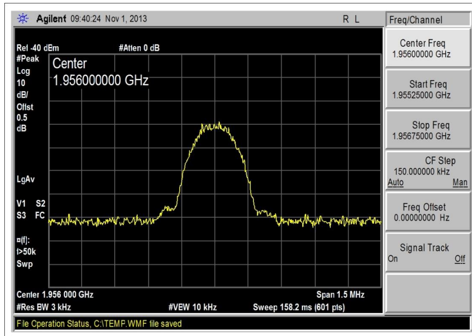
1930-1990MHz DL_GSM_Input
