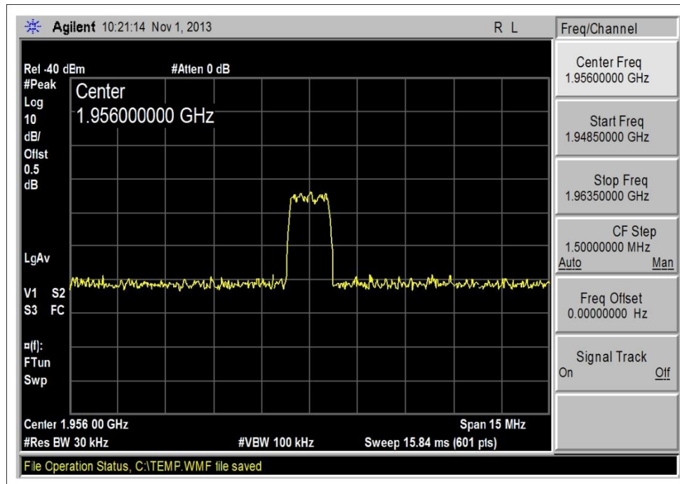
1930-1990MHz DL_CDMA_Input
