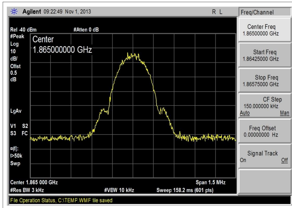
1850-1910MHz UL_GSM_Input
