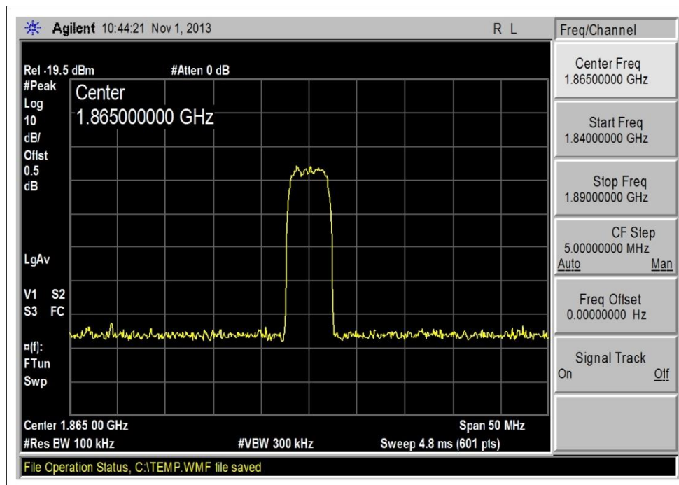
1850-1910MHz UL_WCDMA_Input
