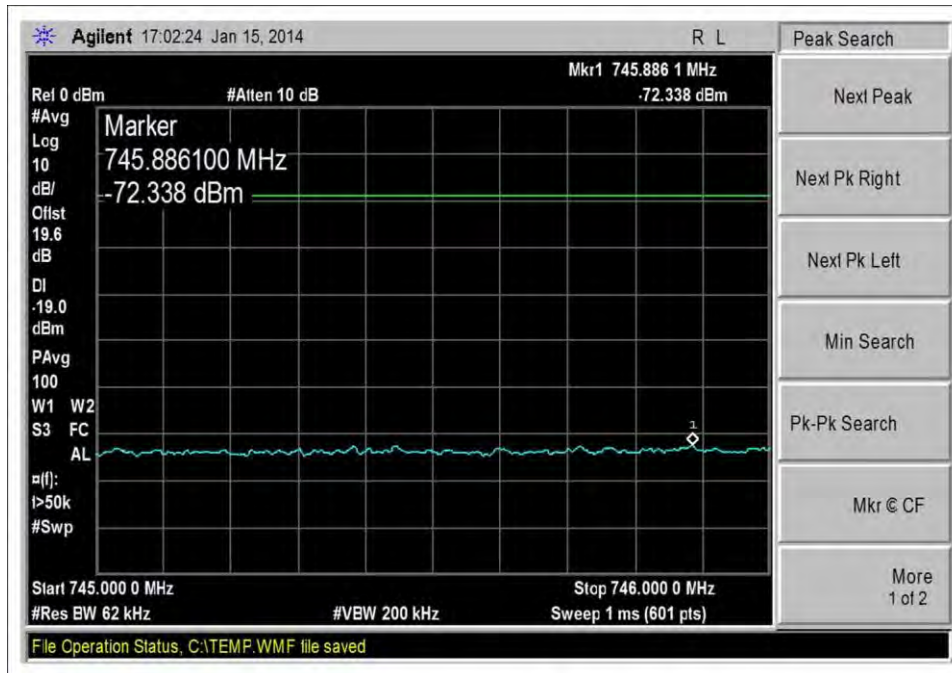
DL_746-757MHz_LTE_L_-20dBm
