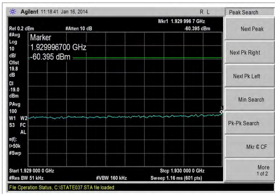
DL_1930-1995MHz_CDMA_L_-60dBm
