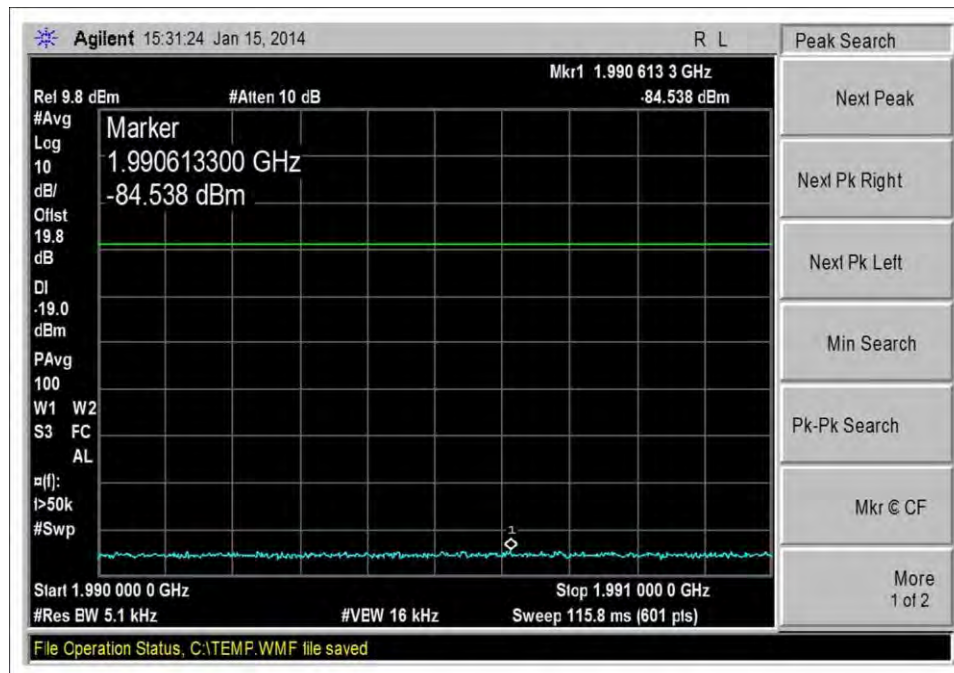
DL_1930-1995MHz_GSM_H_-20dBm
