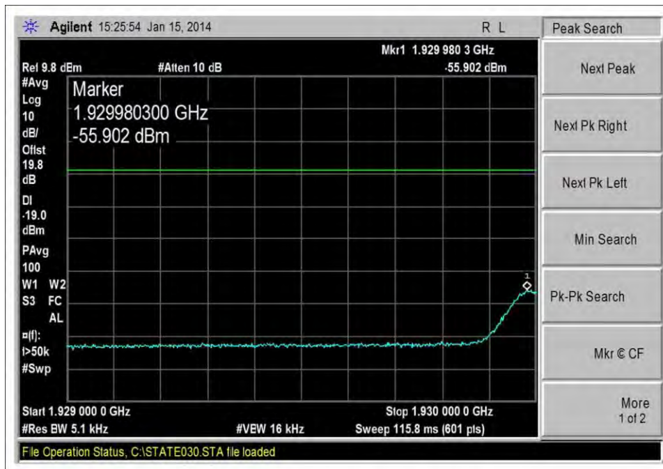
DL_1930-1995MHz_GSM_L_-60dBm
