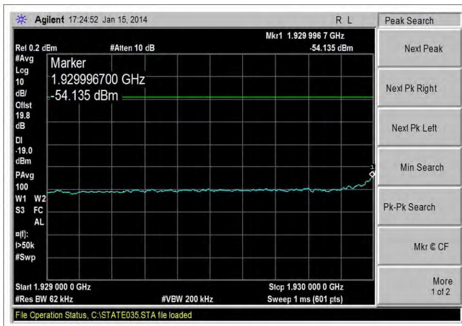
DL_1930-1995MHz_LTE_L_-60dBm
