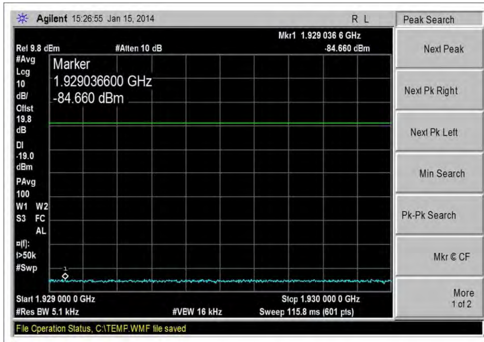
DL_1930-1995MHz_GSM_L_-20dBm
